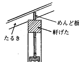
参考図 5.4.5 めんど板
