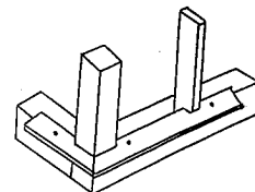
参考図 8.4.7 雨 押 え
