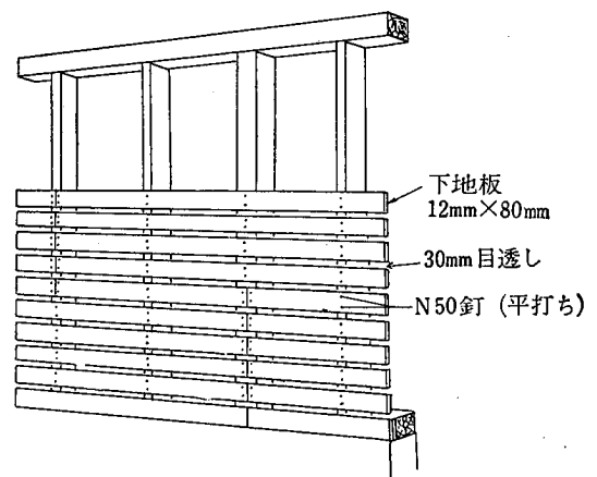
参考図 5.2.21 ラス下地板張り
