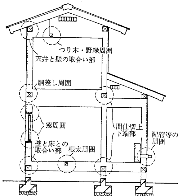
参考図 7.2.1.1-8 断熱材施工工事ですき間の生じやすい箇所
