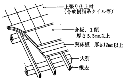
参考図 8.1.2.3 2重下地板
