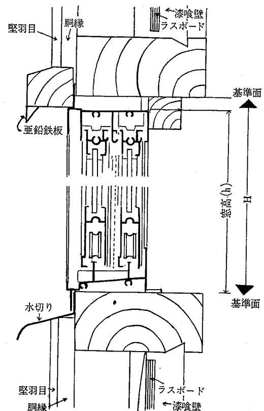
参考図 11.1-2 アルミサッシの一例 (断面)
