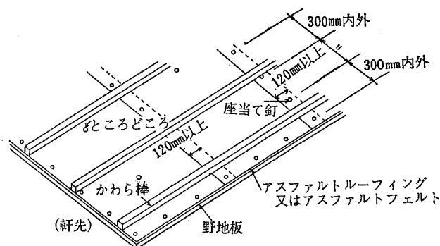
参考図 6.1.1-2 下ぶき工法
