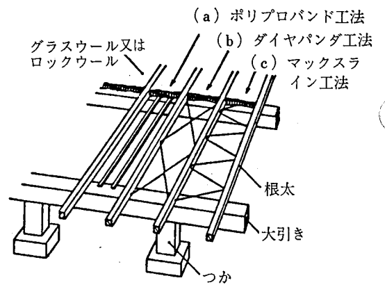
参考図 7.2.2 床断熱施工の新工法
