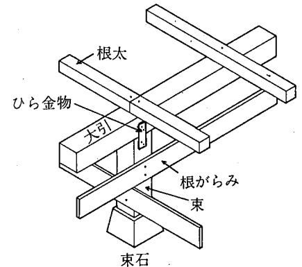
参考図 5.5.2-2 床組
