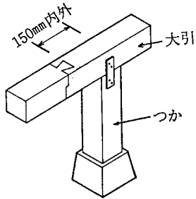
参考図 5.5.1-2 大引の継手
