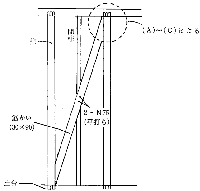
参考図 5.2.1-2 筋かい取付け
