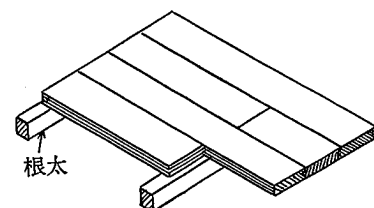
参考図 8.1.4 縁 甲 板
