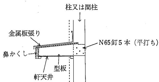
参考図 5.6.1 陸 ひ さ し
