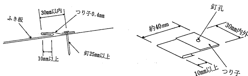
参考図 6.2.2-5 つり子止め
