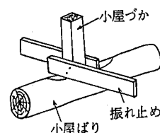
参考図 5.3.4 振れ止め
