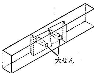
参考図 5.1.5-2 胴差の継手 (追掛大せん継ぎ)
