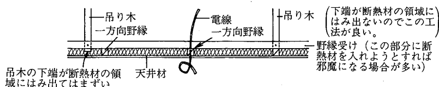
一方向野縁を設けた施工例
