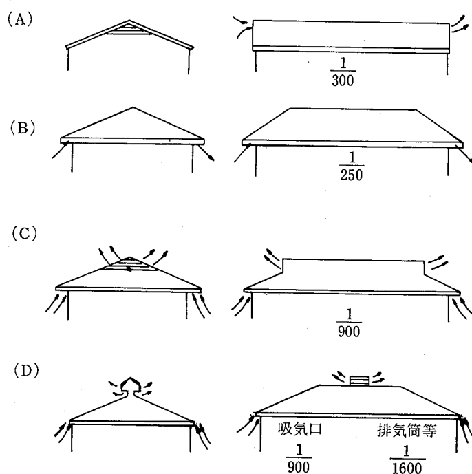
参考図 7.1.5.2-1 換気口の取り方例
