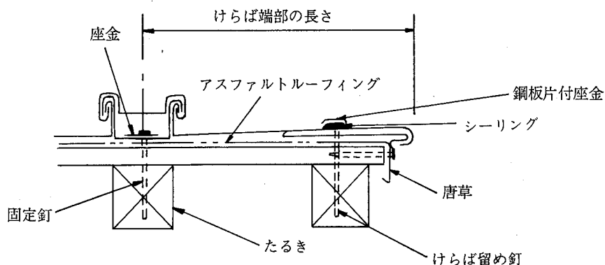
参考図 6.3.3-2 かわら棒ぶきの工法 (心木がなしの場合)
