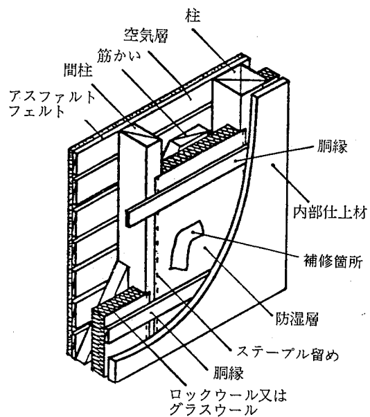
参考図 7.2.1.2 壁の断熱材施工例（無機繊維系）
