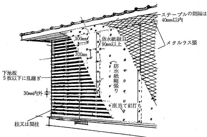
参考図 9.1.1-1 ラス張下地工法とメタルラス張
