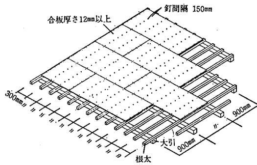
参考図 8.1.1.2 合板下地
