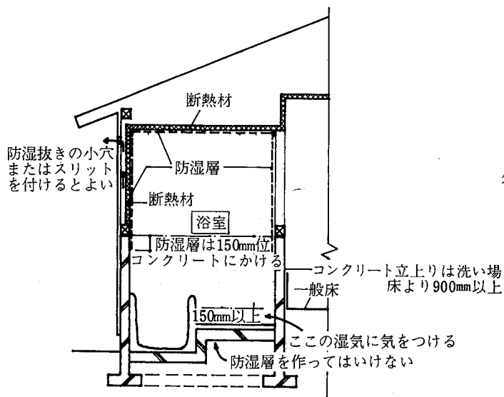
参考図 7.2.4 浴室 断面 例
