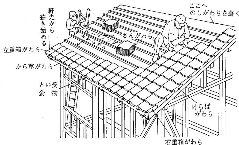
日本瓦葺の図
