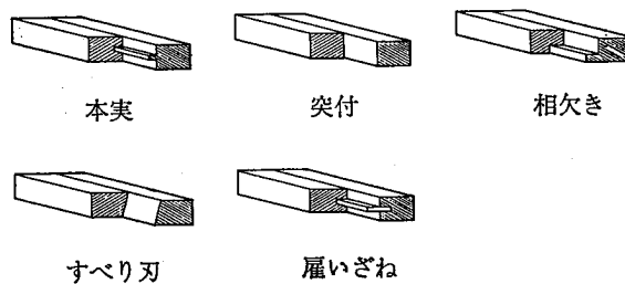
参考図 8.1.5 板 の 継 ぎ 方
