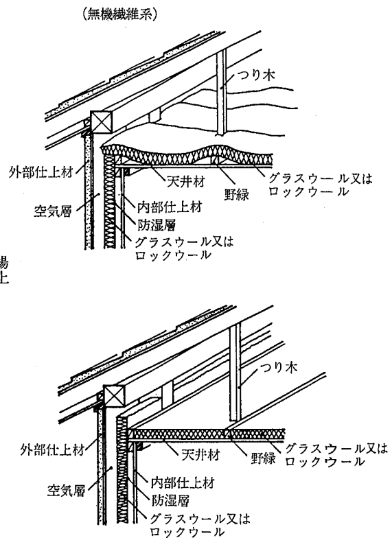
参考図 7.2.5 壁と天井回りの断熱材の納め方
