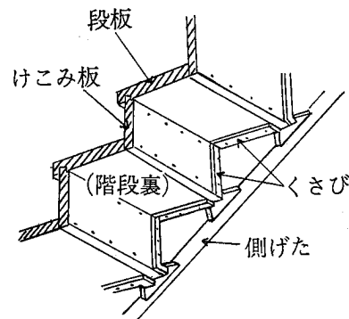
参考図 8.8.2 段板及びけこみ板
