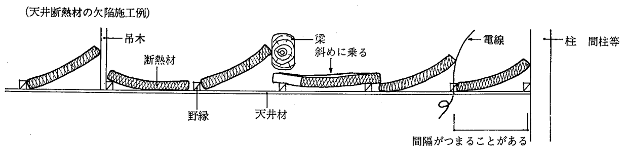
参考図 7.2.3-1 天井の断熱材施工の注意点
