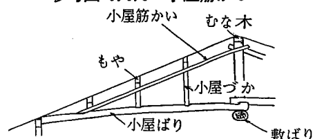
参考図 5.3.5 小屋筋かい
