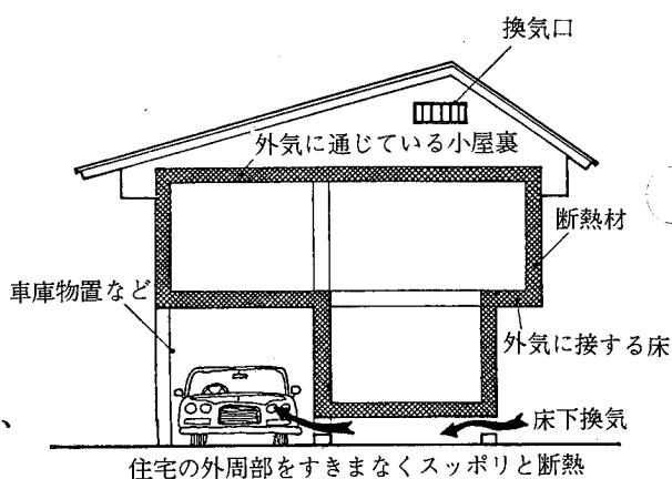
参考図 7.1.1 断熱材施工の基本
