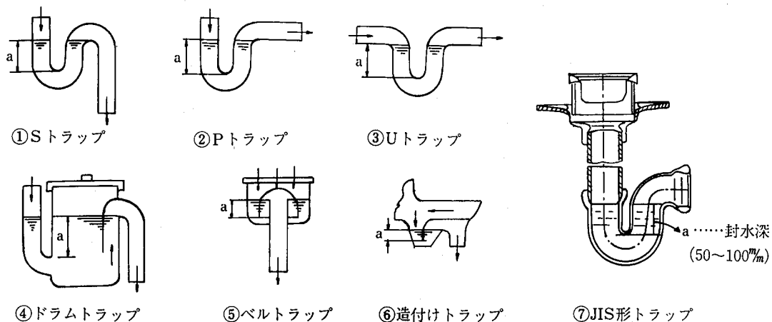
参考図 13.2.2-5 トラップの種類
