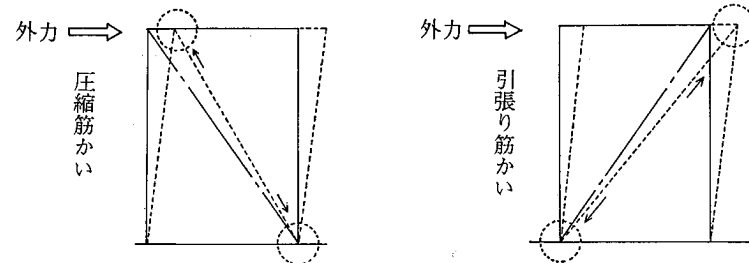
参考図 5.2.1-2 筋かい取付け
