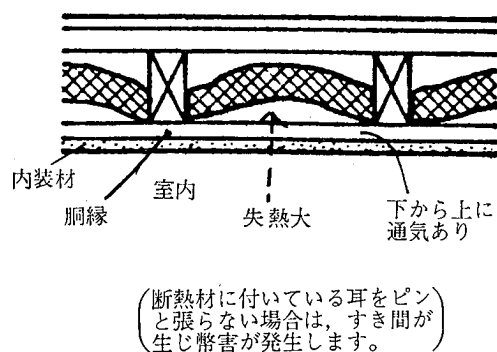
7.1.1.2 壁の施工例（悪い例）
