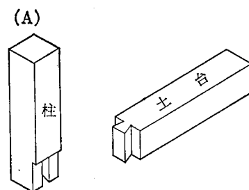
参考図 5.1.3-2 柱と土台の仕口 (落としあり)
