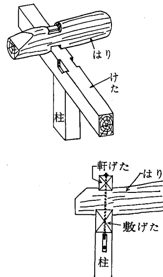
参考図 5.3.4 振れ止め
