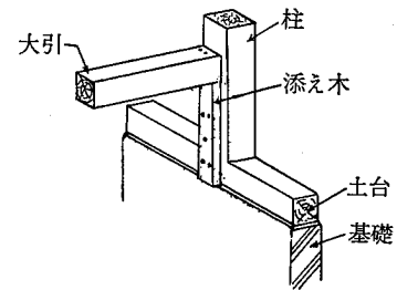
参考図 5.5.1-3 大引と柱との仕口
