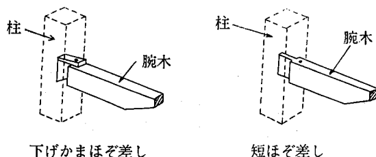
参考図 3.11.2-1 腕木の取付
