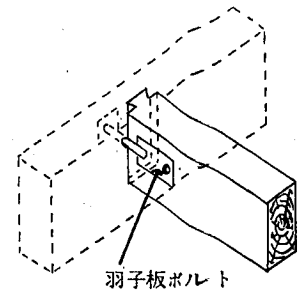
参考図 3.4.5-4 T字取合
