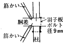
参考図 3.2.8-2 1, 2階とも同じ柱間に筋かい が取り付け場合
