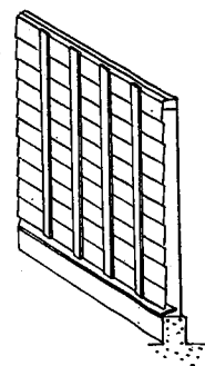
参考図 3.9.3 押縁下見板張り
