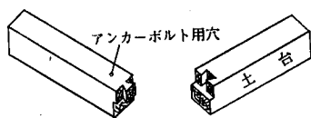
参考図 3.2.1-1 土台の継手 (腰掛けあり継ぎ)
