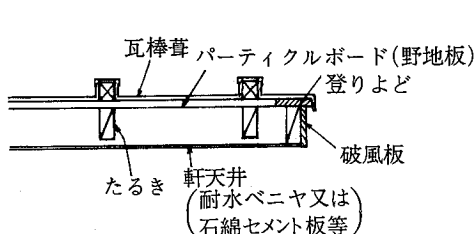
参考図 3.5.5-3 けらば及び軒先納まり
