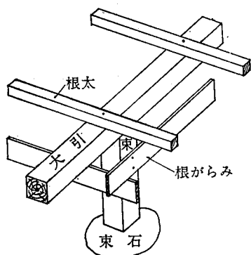
参考図 3.4.4 床 組
