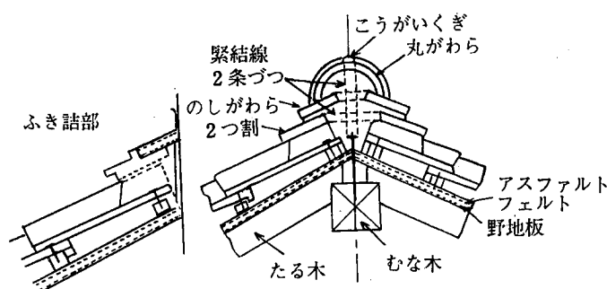
参考図 4.4.2-1
