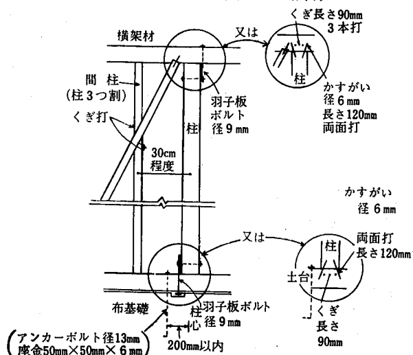
参考図 2.4.8 3.2.8 筋かいの取付け
