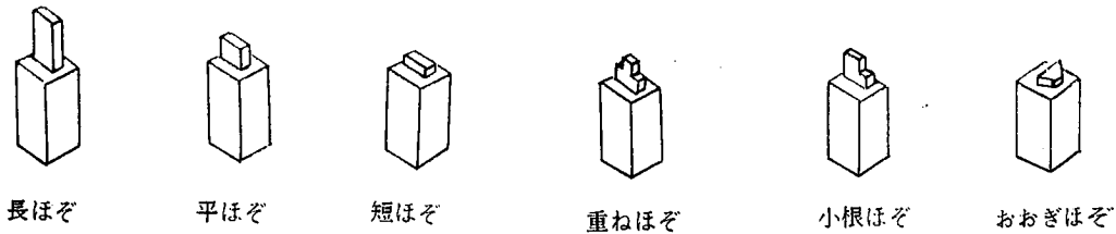
参考図 3.1.4 木 構 造 用 金 物
