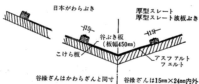
参考図 4.2.4-1 かわらぶきの谷の納り
