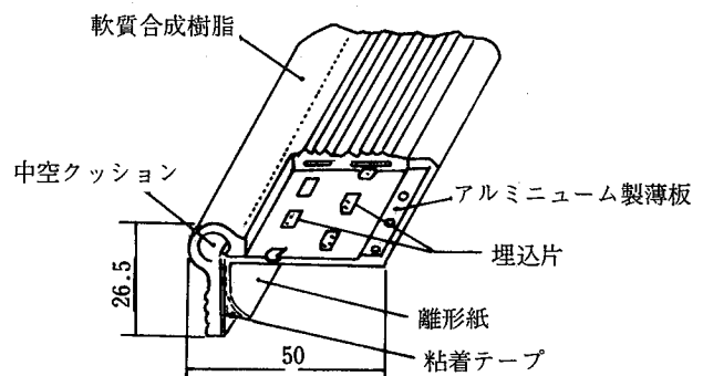
階段すべり止め例
