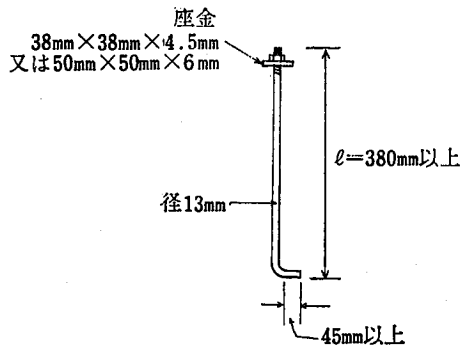
取付ボルト
