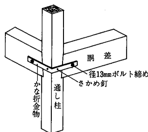
参考図 3.2.4-2 通し柱と胴差と の取合
