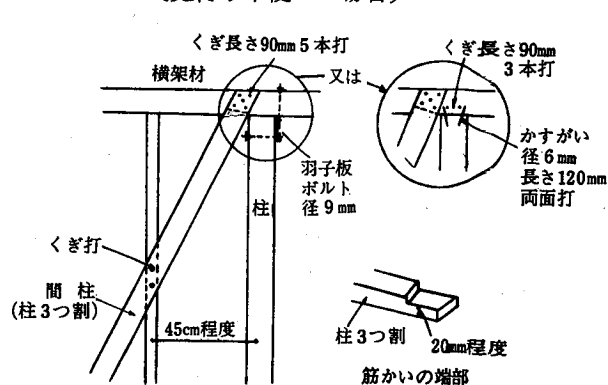
参考図 2.4.8 3.2.8 筋かいの取付け
