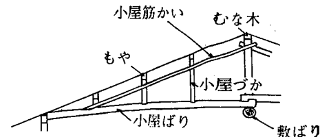
参考図 3.3.4 振れ止め
