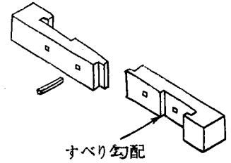
そぎ継ぎ
