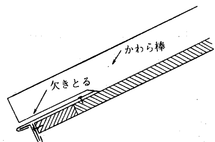
参考図 4.2.7-3
