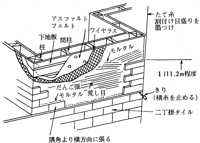
参考図 5.8.3-1 陶磁器質タイル張り
