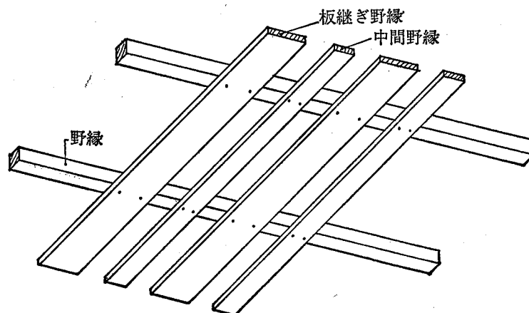
19図 天 井 下 地
