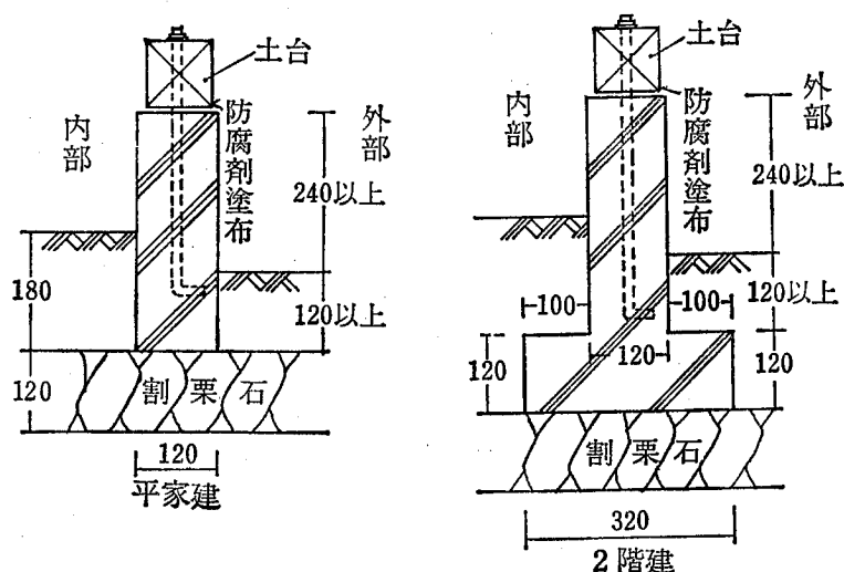
1 図 布 基 礎 詳 細
