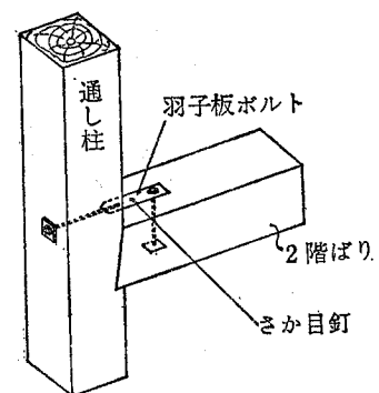
16図 通し柱と2階ばり との取合
