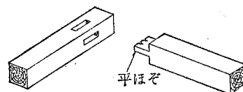
3図 土台すみ仕口 (平ほぞ打ち抜き割りくさび締め)
