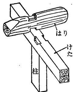
12図 小屋とけたとの取合(わたりあご)
