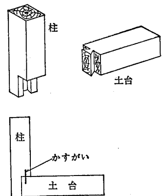
6図 柱と土台の取合 (落しあり)
