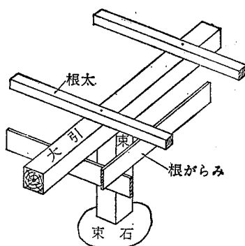
14図 床 組
