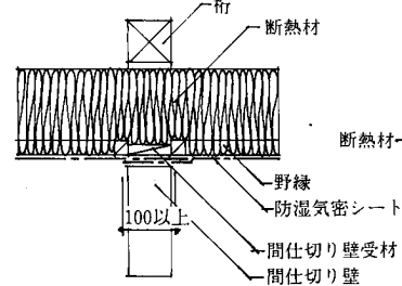
最上階の天井と間仕切り壁の取合い (間仕切り壁の上部で 防湿気密シートを継ぐ場合)
