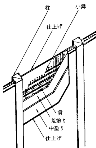
参考図 I.5.-1 真壁
