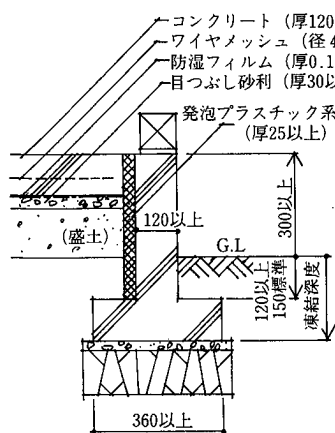
イ. 内断熱施工例
