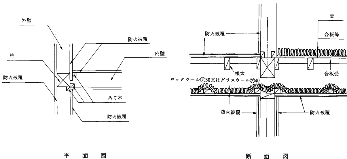
参考図18.1.4 界壁以外の内壁
