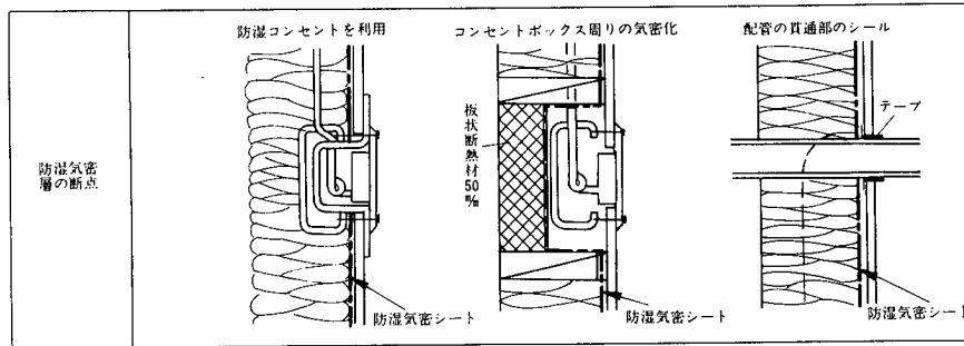
参考図 IV.8.6 防湿気密層の連続性を保つための方法
