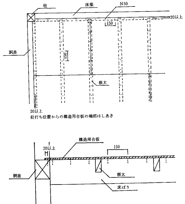
参考図 17.4.2-1 根太と床梁（胴差し）の上端高さが同じ場合の下地板の取り付け
