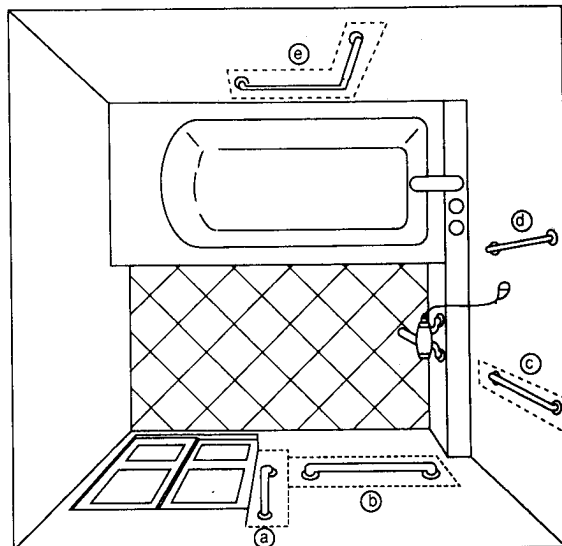
参考図 III.3.4-3 浴室手すりの標準的な設置例
