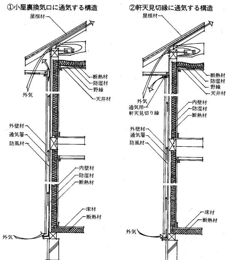
参考図Ⅱ.9-2 外壁に通气層を設け壁体内通気を可能とする構造
