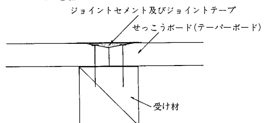
ニ. テーピング処理
