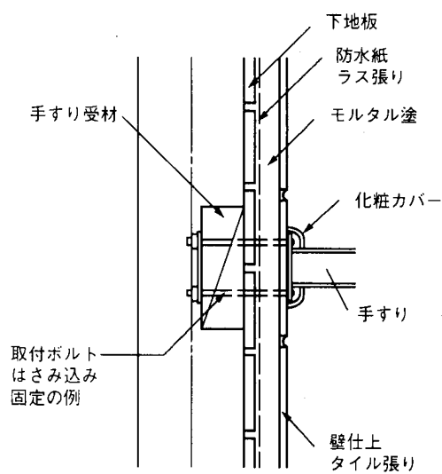
浴室の受け材設置の例
