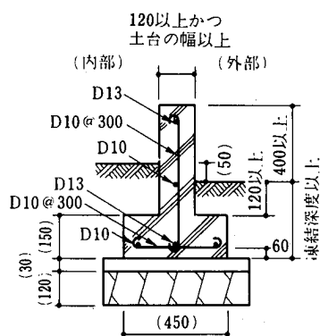
イ. 布基礎詳細 (mm)
