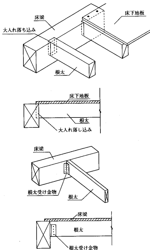
参考図 17.4.2-1 根太と床梁の上端高さが同じ場合の根太の取り付け例
