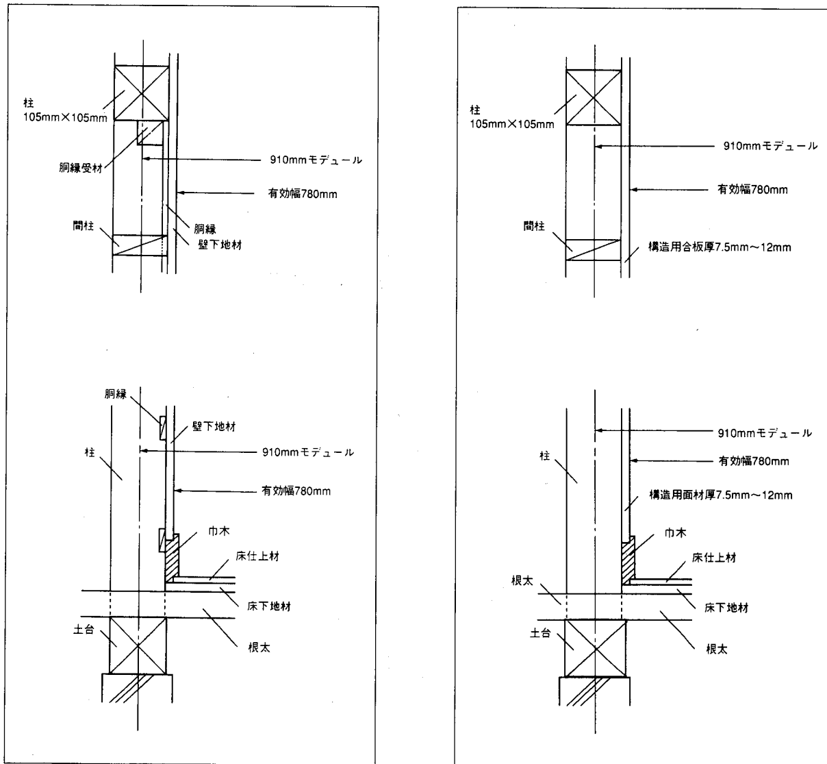
(イ) 胴縁を用いる場合
