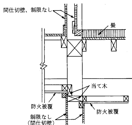
参考図 17.6.7 間仕切壁直上の当て木
