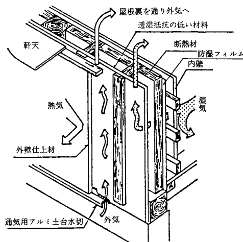
参考図 I.5.-3 通気層を設けた外壁
