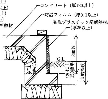
ロ. 外断熱施工例
