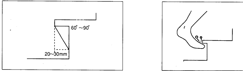
参考図 III.3.2-2 蹴込み部分の留意点
