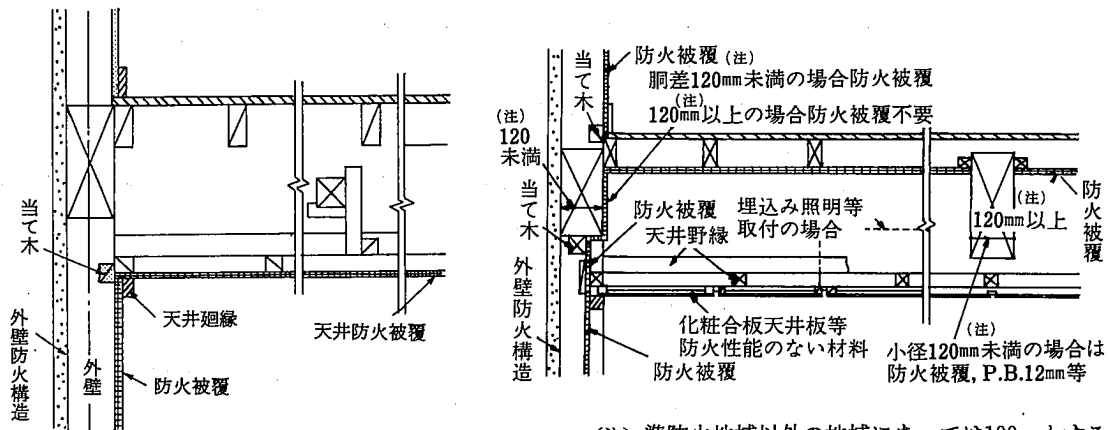
参考図 17.6.5 天井等の防火被覆
