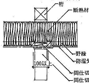
最上階の天井と間仕切り壁の取合い (間仕切り壁の上部で 防湿気密シートを継ぐ場合)
