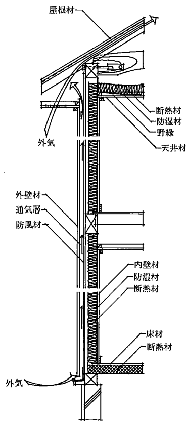
①小屋裏換口に通気する構造
