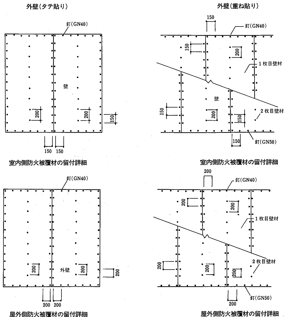
参考図23.6 防火被覆材の留付方法
