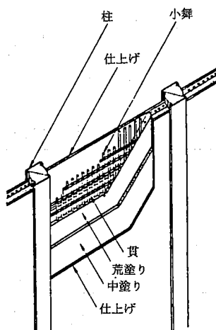
参考図 18.5.-1 真壁
