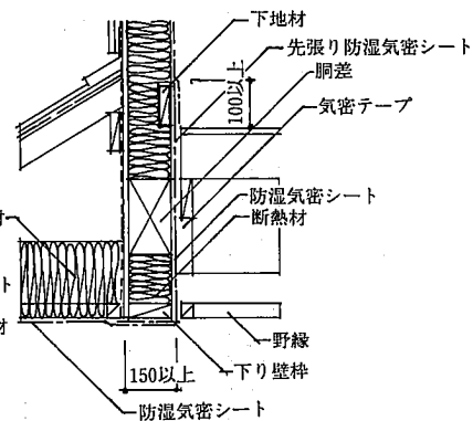
下屋部分の天井と外壁の取合い (外壁及び下がり壁部分に先張り防湿気密シートを 張る場合)
