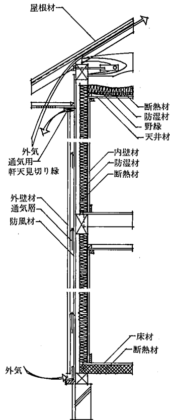
②軒天見切縁に通気する構造
