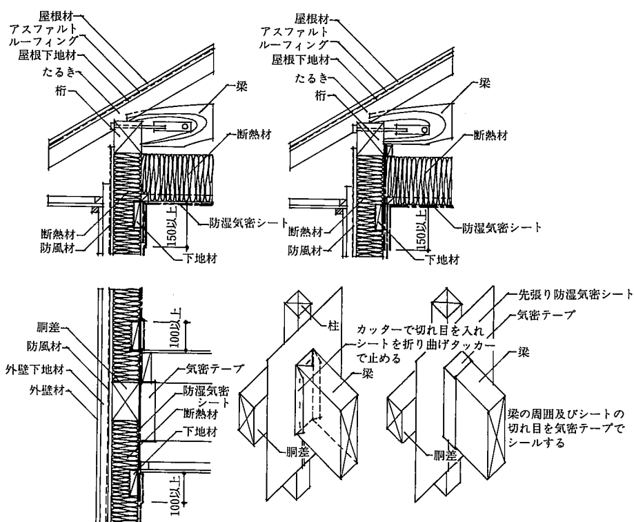
外壁部と最上階の天井との取合い (最上階の天井と取合う外壁部に先張り 防湿気密シートを桁まで留め付ける場合)
