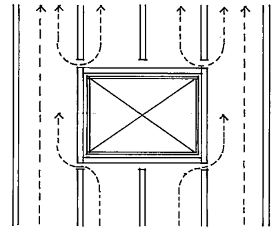
④開口部まわり横胴縁の施工例
