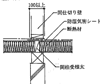
最上階の天井と間仕切り壁の取合い (間仕切り壁の上部で 防湿気密シートを継ぐ場合)
