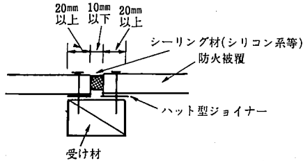
ハ. シーリング目地
