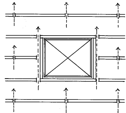
④開口部まわり横胴縁の施工例
