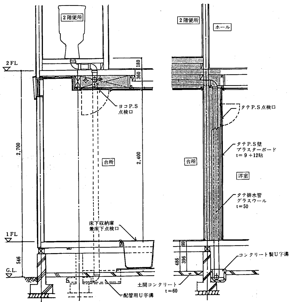
参考図 19.11.2 配 管
