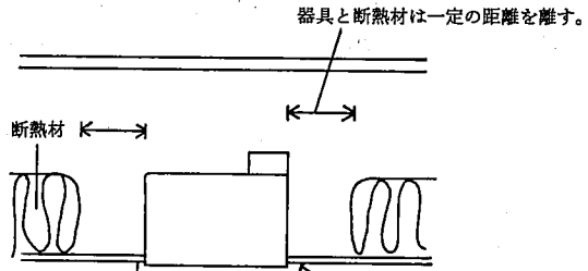
参考図 7.6.6 ダウンライトの取合い
