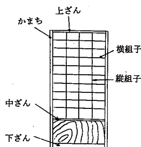
腰付き障子
