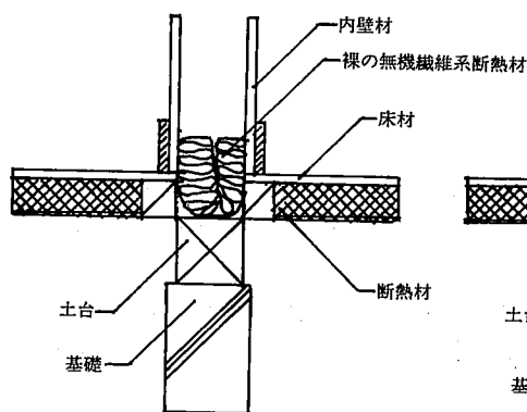
間仕切り壁と床との取合い部 (床根太が直行する場合)
