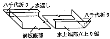
参考図 6.2.7-1 八千代折り
