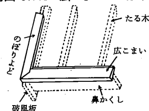
参考図 5.7.4 めんど板
