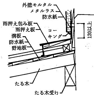
水上部分と壁との取合い
