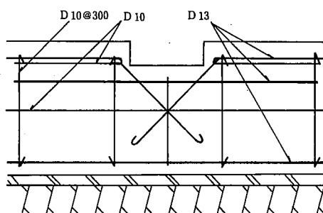
ロ. 換気口廻りの補強
