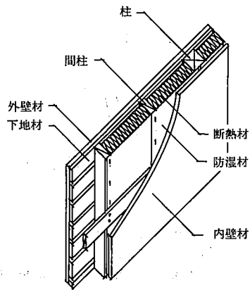
参考図 7.6.4 図 壁の断熱材施工例
