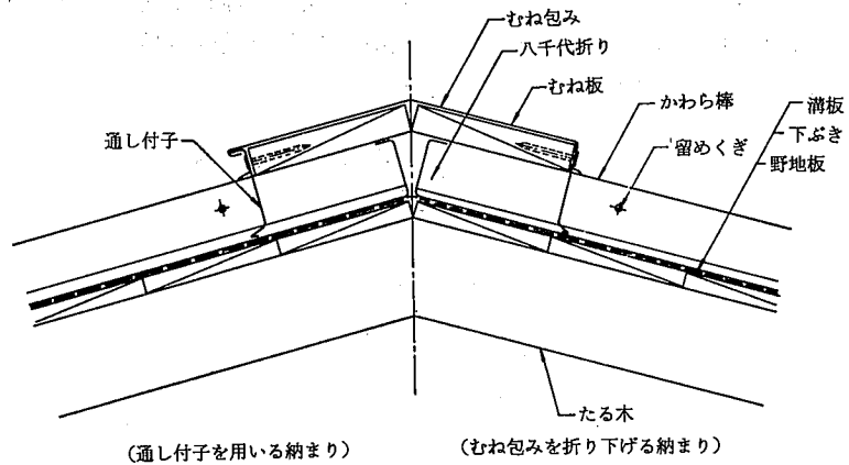
参考図 6.2.8
