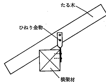
参考図 5.5.5-4 たる木とひねり金物
