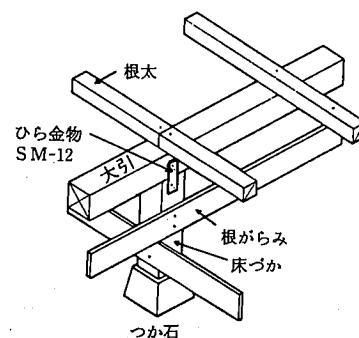
参考図 5.8.1 床組
