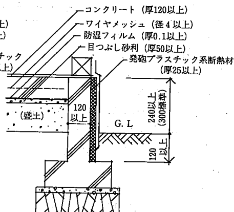
(ロ) 外壁断熱施工例
