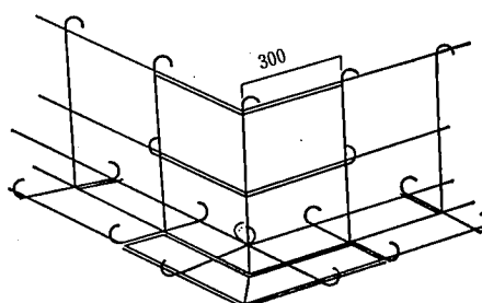
ハ. コーナー部補強
