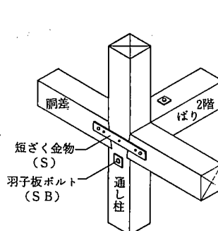
参考図 5.8.5 通し柱と2階ばり との取合
