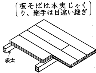
参考図 8.1.5 普通床板 (縁甲板)
