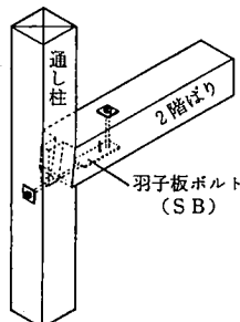
参考図 5.8.5 通し柱と2階ばり との取合
