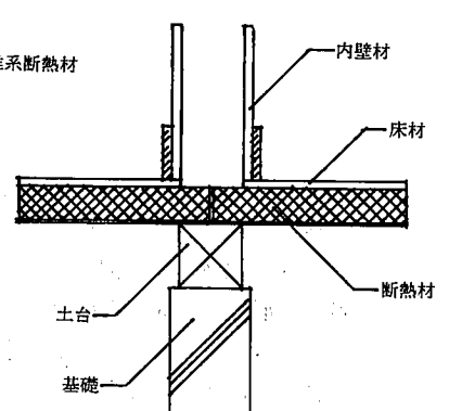
間仕切り壁と床との取合い部 (床根太が直行する場合)
