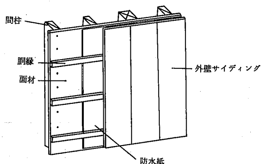
参考図 8.5 サイディングの施工例
