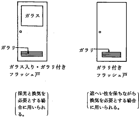
参考図 11.2.5 フラッシュ戸
