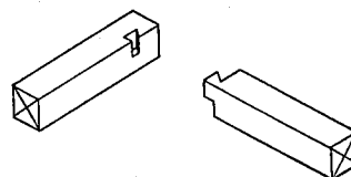
参考図 5.1.3 柱と土台の仕口 (落しあり)
