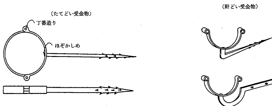
参考図 6.7.4 とい受金物
