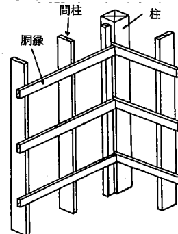
参考図 8.3.1 胴 縁
