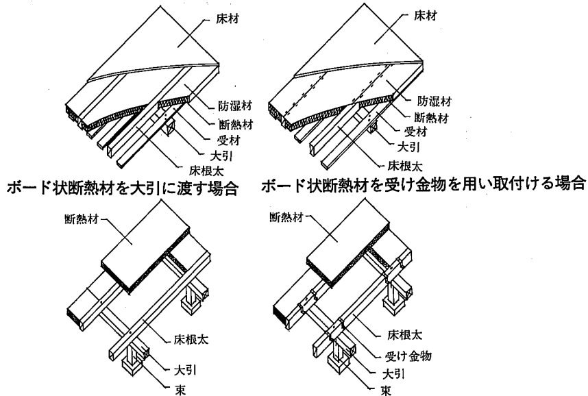
参考図 7.6.3 床の断熱材施工例
