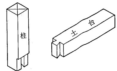
参考図 5.1.3 柱と土台の仕口 (落しあり)
