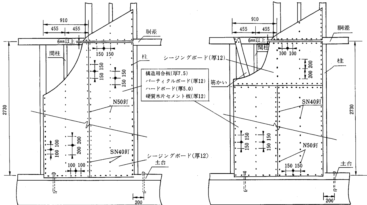
(A) 3'×9'版の縦張りの場合
