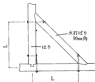
参考図 5.8.6 火打ばり
