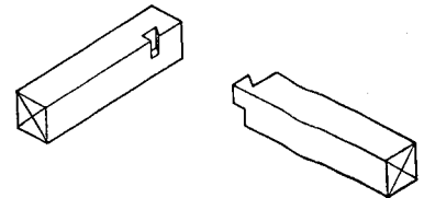
参考図 5.1.3 柱と土台の仕口 (落しあり)
