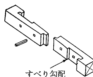
そぎ継ぎ
