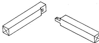
参考図 5.1.2 火打土台仕口 (かたぎ入れN90釘2本打ち)
