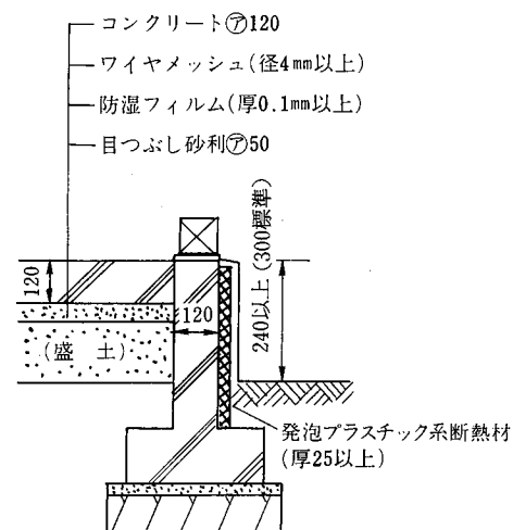
ロ. 外断熱施工例
