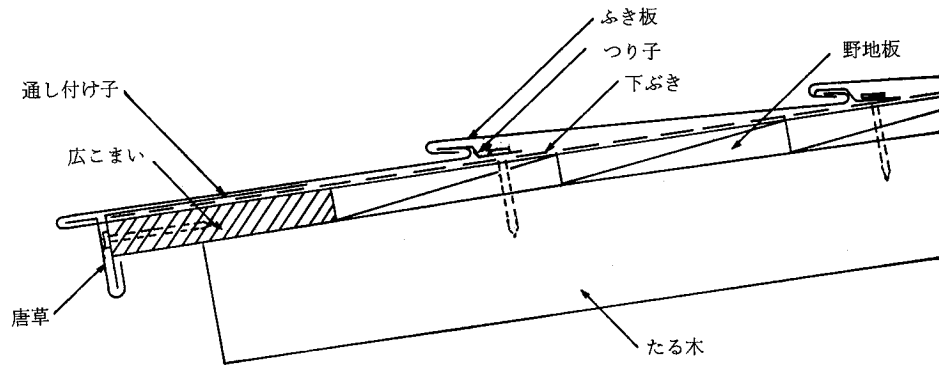
参考図 6.2.5-2 銅板による一文字ぶき
