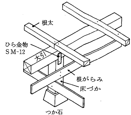
参考図 5.8.1 床組
