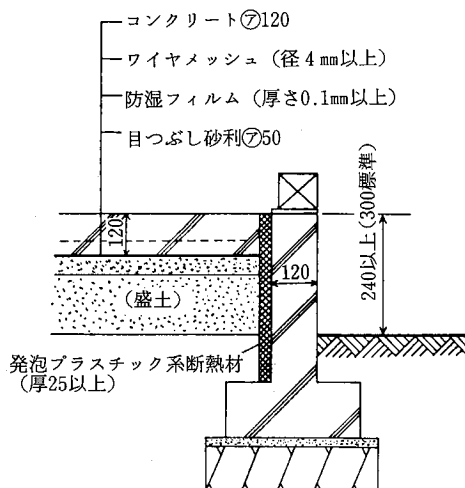
イ. 内断熱施工例
