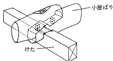
参考図 5.5.1-2 小屋ばりの継手 (台持継ぎ) 参考図 5.5.1-4 小屋ばりと軒げたとの仕口 (かぶとあり)
