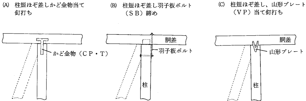
参考図 5.2.2-1 筋かいの上端部が取付く柱の仕口
