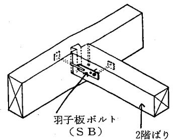
参考図 5.8.5 T字仕口
