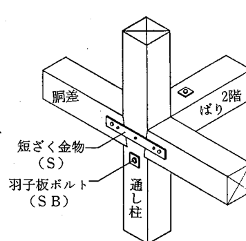
参考図 5.8.5 通し柱と2階ばりとの取合
