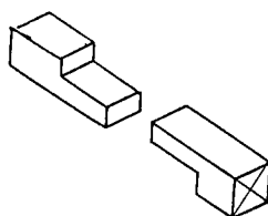
相欠き継ぎ・腰掛け継ぎ
