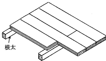
参考図 8.1.5 普通床板（縁甲板）
