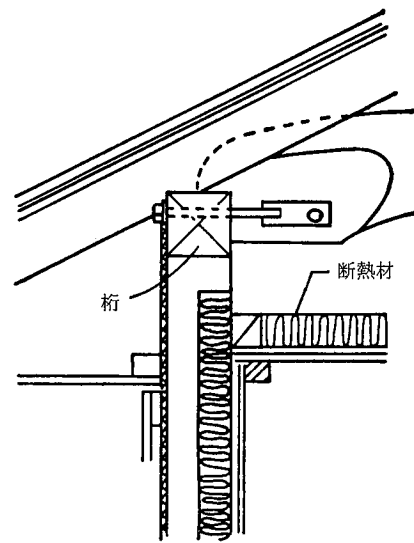
(B) 外壁
