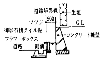
参考図 19.13.2 植栽（既存擁壁のバリエーション）
