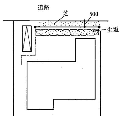
参考図 19.13.2 植栽（既存擁壁のバリエーション）
