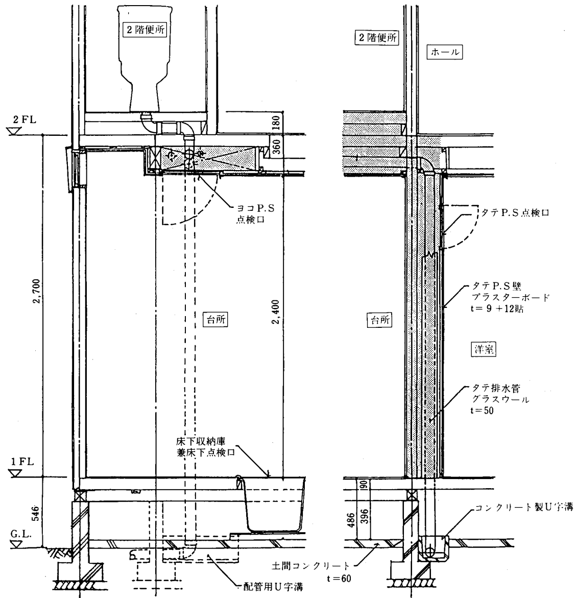
参考図 19.12.2 配 管
