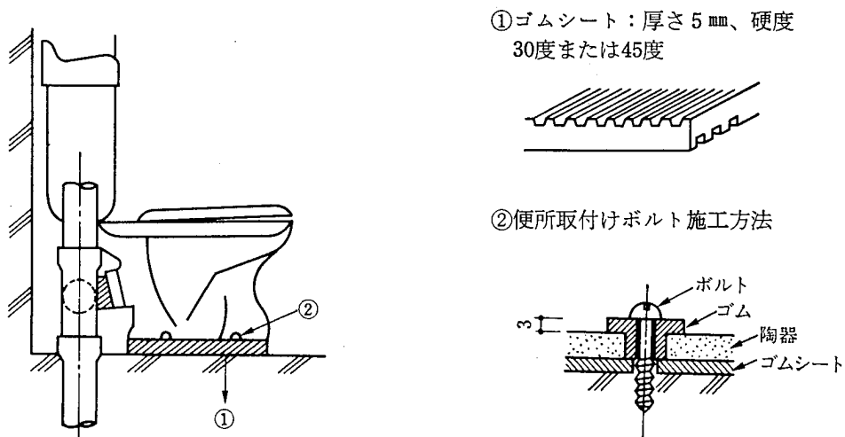
参考図 19.12.3-2 便器の取付け
