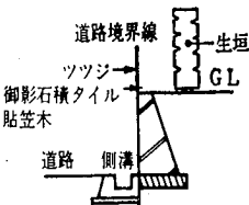
参考図 19.13.2 植栽（既存擁壁のバリエーション）
