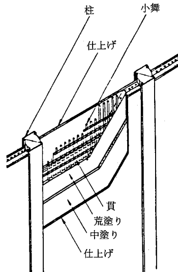
参考図 18.5.-1 真 壁
