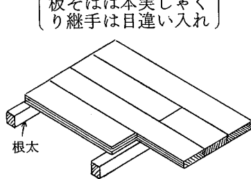
参考図 8.1.5 普通床板（縁甲板）
