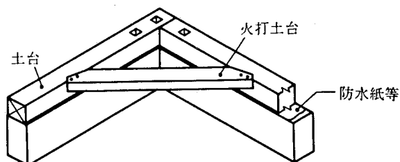
参考図 19. 7 土台の防腐措置
