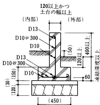
イ. 布基礎詳細(mm)
