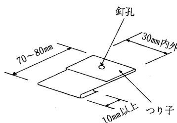
参考図 6.2.2-3 つり子止め
