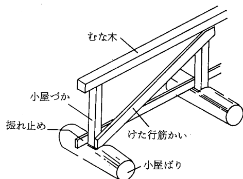
参考図 5.5.4 けた行筋かい・振れ止め
