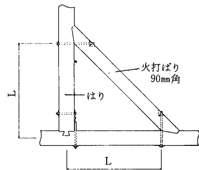
参考図 5.8.6 火打ばり
