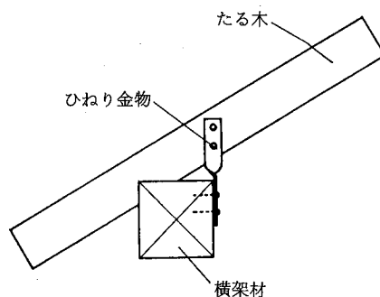
参考図 5.5.5-4 たる木とひねり金物
