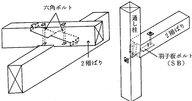
参考図 5.8.5 2階ばり継手 (台持継ぎ)
