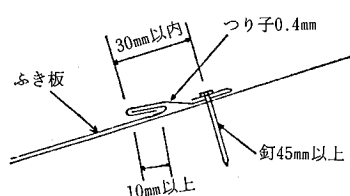
参考図 6.2.2-3 つり子止め
