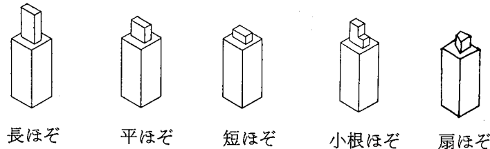
ほ ぞ の 種 類
