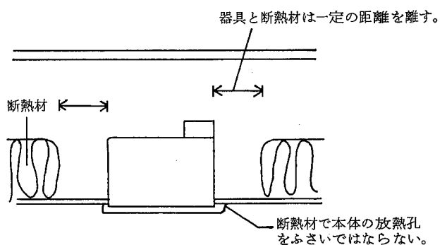
M型ダウンライト
