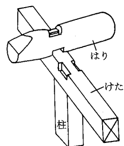
(渡りあり)
