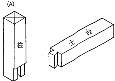
参考図 5.1.3 柱と土台の仕口 (落としあり)
