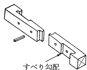
そぎ継ぎ
