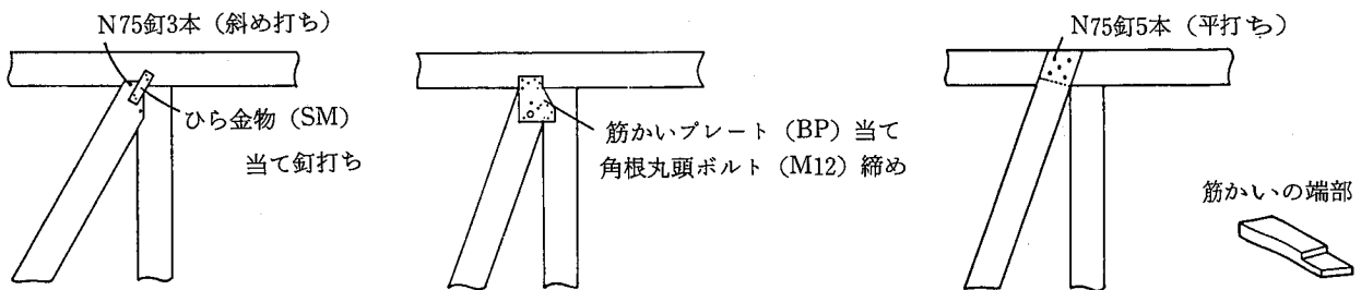
参考図 5.2.2 隅部通し柱の 下部
