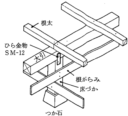
参考図 5.8.1 床組
