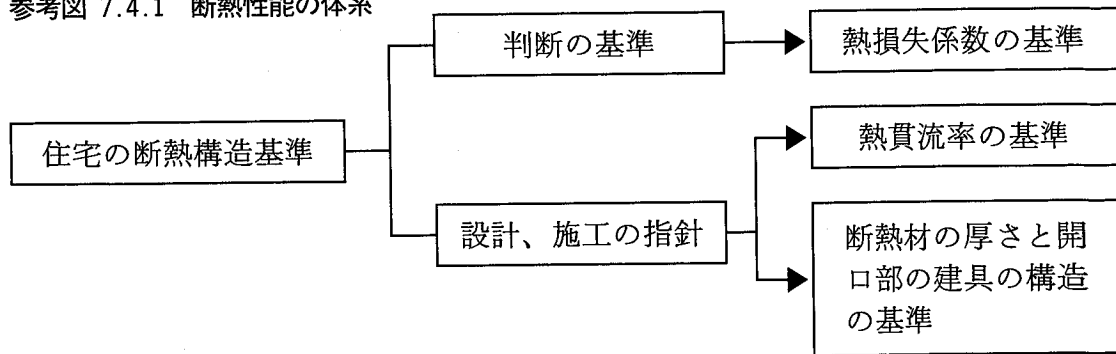
参考図 7.4.1 断熱性能の体系
