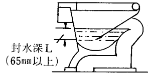
⑥-1 器具内蔵トラップ (洋風サイホン大便器の例)
