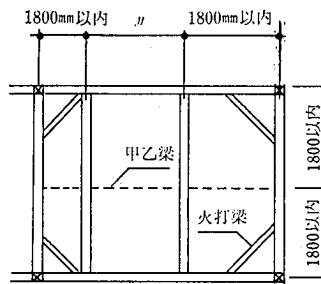
甲乙梁の取付け
