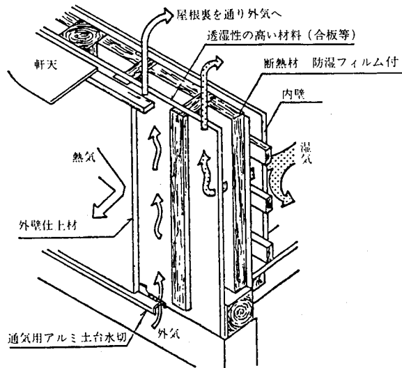
参考図 18.5.-3 通気層を設けた外壁
