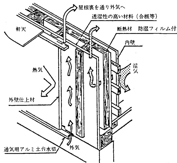
図 18.5.-3 通気層を設けた外壁
