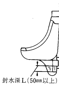
⑥-2 器具内蔵トラップ (壁掛け小便器の例)
