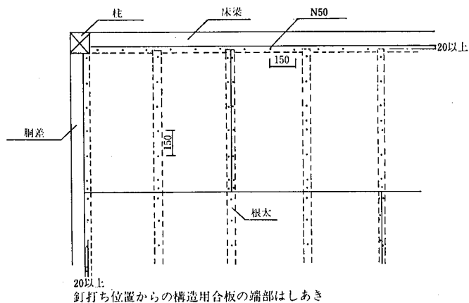
参考図 17.4.2-1 根太と床梁（胴差）の上端高さが同じ場合の下地板の取付け
