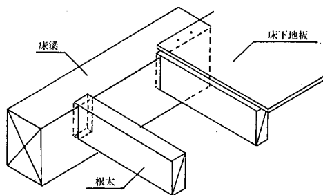
参考図 17.4.2-1 根太と床梁の上端高さが同じ場合の根太の取付け例
