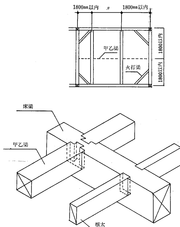
甲乙梁の取付け
