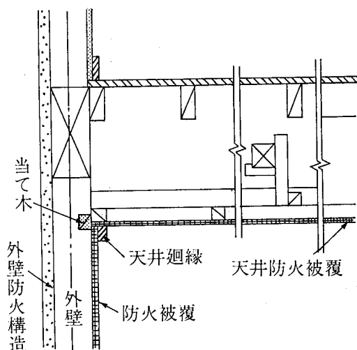
(a) 天井面で防火被覆をする場合
