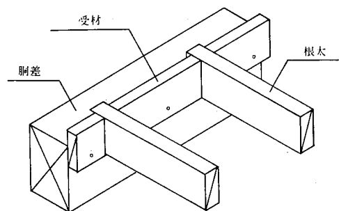
参考図 17.4.2-2 根太と床梁（胴差）の上端高さが異なる場合の根太の取付け例
