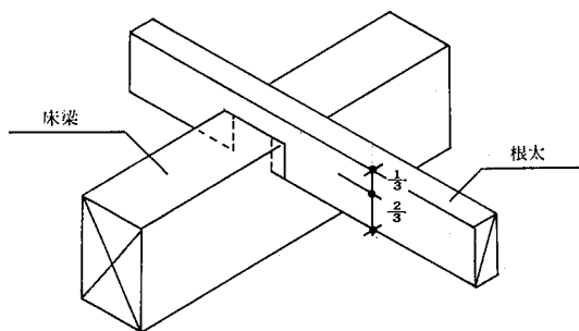
参考図 17.4.2-2 根太と床梁（胴差）の上端高さが異なる場合の根太の取付け例
