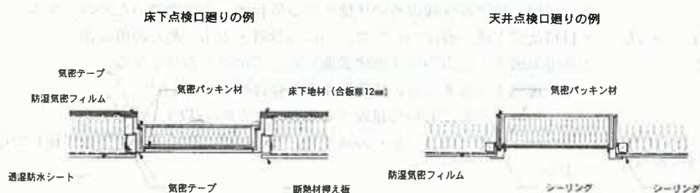
参考図7.9.4.7-1 点検口まわり
