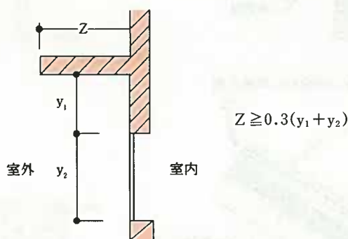
参考図7.5 ひさしによる日射の遮蔽
