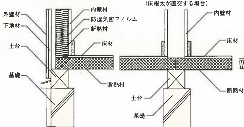
外壁と床との取合い部
