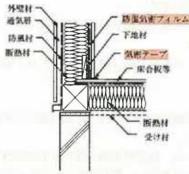
ロ、床合板等を土台に直接釘留め
