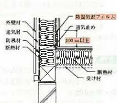
ハ、取合い部外壁内に通気止めを用いる場合
