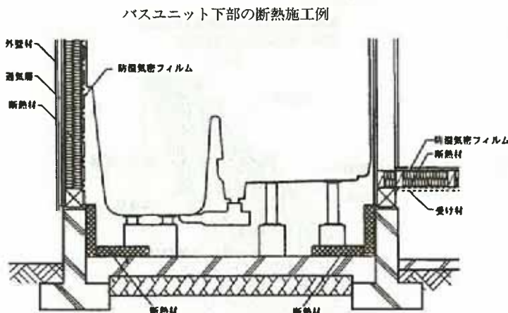
参考図7.4.6-1 特殊な床
