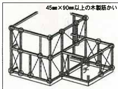
チの仕口
