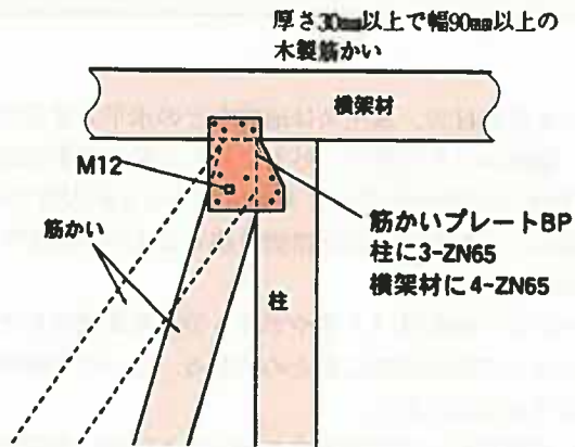
参考図5.2.1-2 筋かいの端部の仕口
