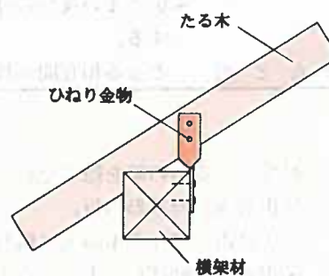
参考図5.5.5 たる木とひねり金物
