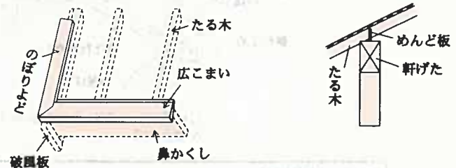
参考図5.7.3 広こまい・のぼりよど 参考図5.7.4 めんど板
