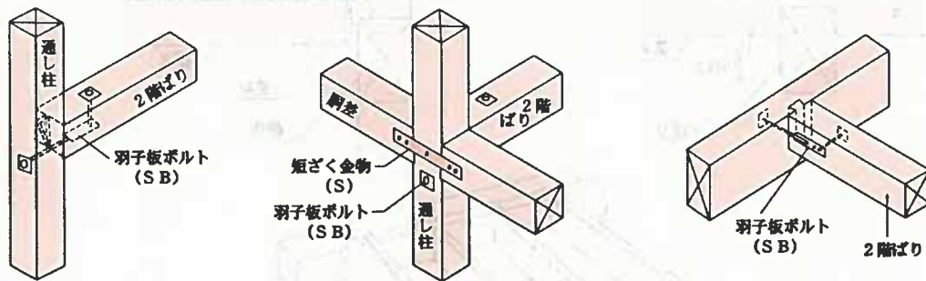
参考図5.8.7-2 床ばり、胴差、柱の緊結の例
