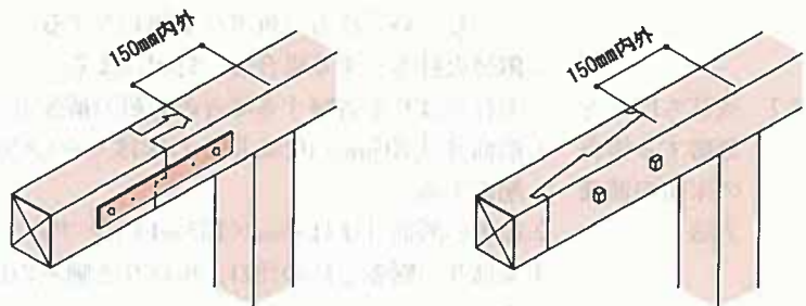
参考図5.8.5-2 2階床ばりの継手
