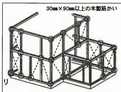
リの仕口
