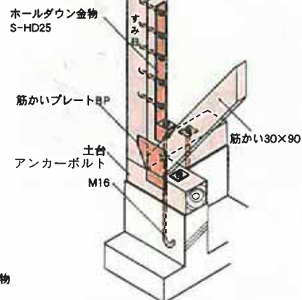
リの仕口 ホールダウン金物 S-HD25
