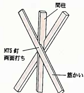
参考5.1.8 たすき掛筋かい交差部
