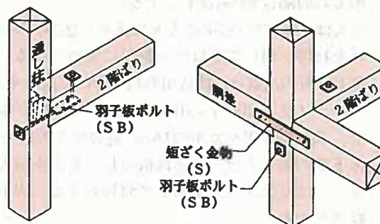
参考図5.8.5-3 通し柱と2階ばりとの取合
