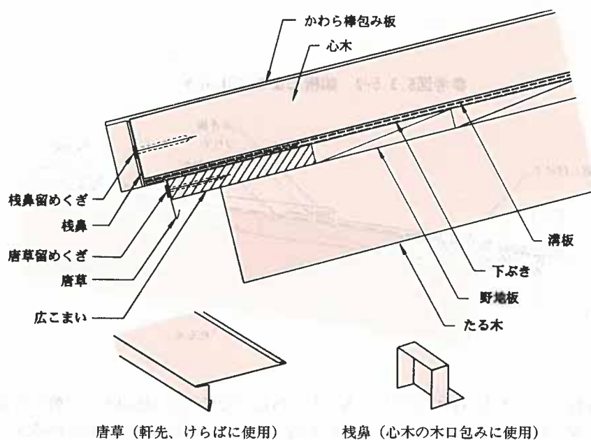
参考図6.3.9 軒部の納り
