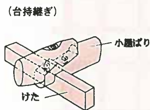
参考図5.5.1-1 小屋ばりの継手
