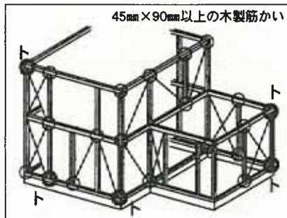
トの仕口
