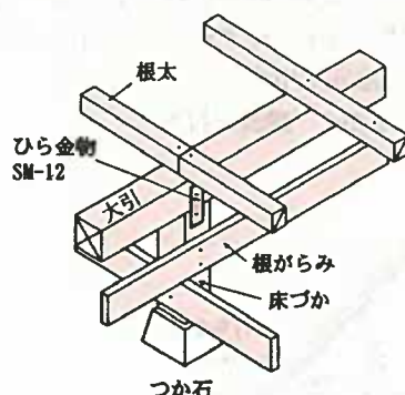
参考図5.8 床組
