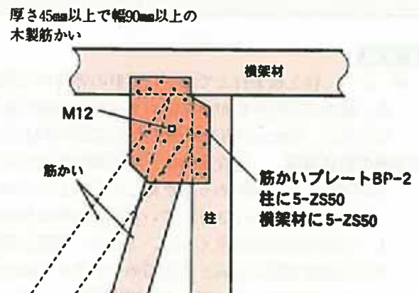
参考図5.2.1-2 筋かいの端部の仕口
