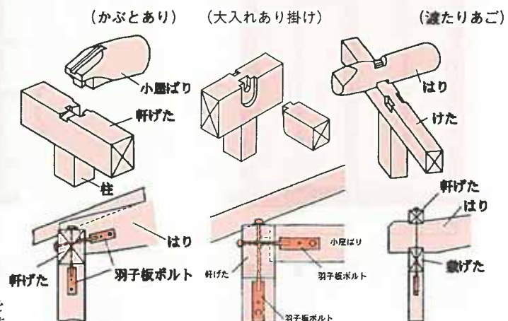
参考図5.5.1-2 小屋ばりと軒げたとの仕口
