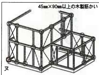
ヌの仕口
