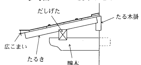
参考図 5.9.2 腕木ひさし
