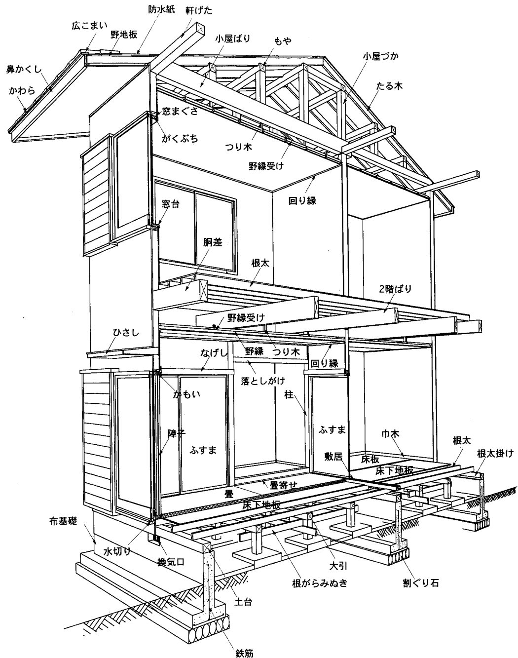
参考図 8.2 敷居・かもし・その他
