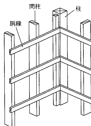
参考図 8.3.1 胴 縁
