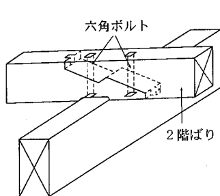
参考図 5.8.5 2階ばり継手 (台持継ぎ)
