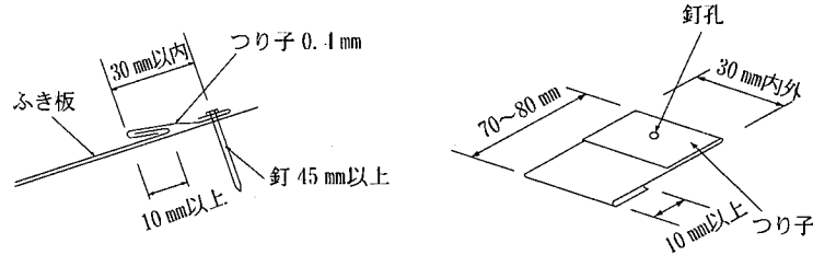
参考図 6.2.2-3 つり子止め
