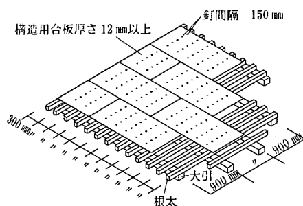
参考図 8.1.2 構造用合板下地板
