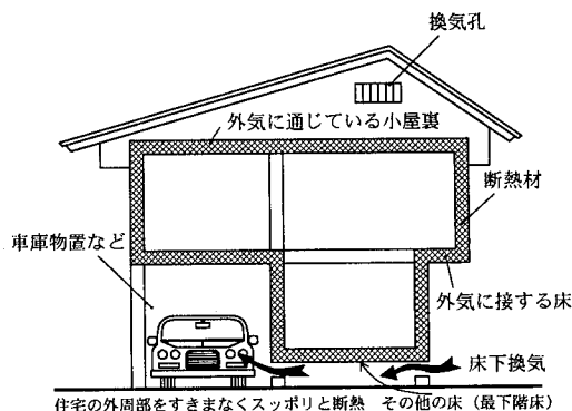
参考図 7.3.1 断熱材施工の基本
