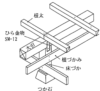
参考図 5.8.1 床組
