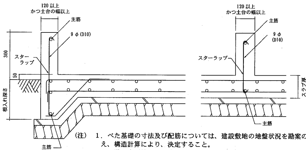
べた基礎詳細図 (mm)
