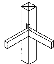
参考図 8.12.2 回り縁入すみ (下端留め)
