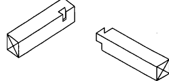
参考図 5.1.1 土台すみ仕口 (片あり掛け)
