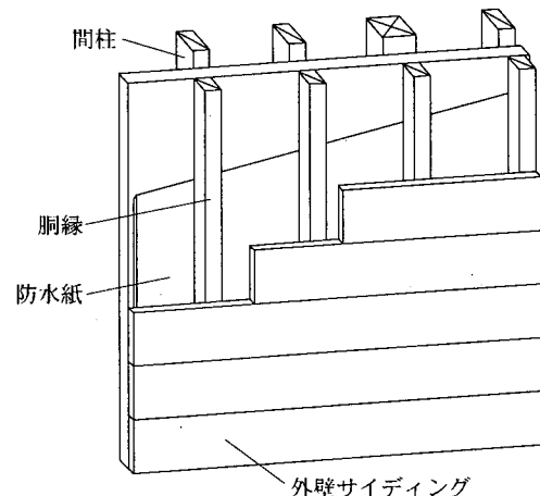
ロ、縦胴縁を介してサイディングを施工する場合
