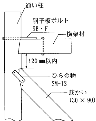
参考図 5.2.1 筋かいと通し柱の取合い
