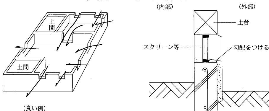
参考図 3.3.7 床 下 換 気
