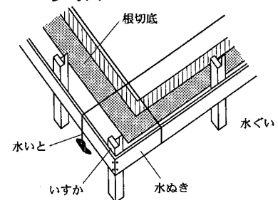
参考図 2.1.3 やりかた
