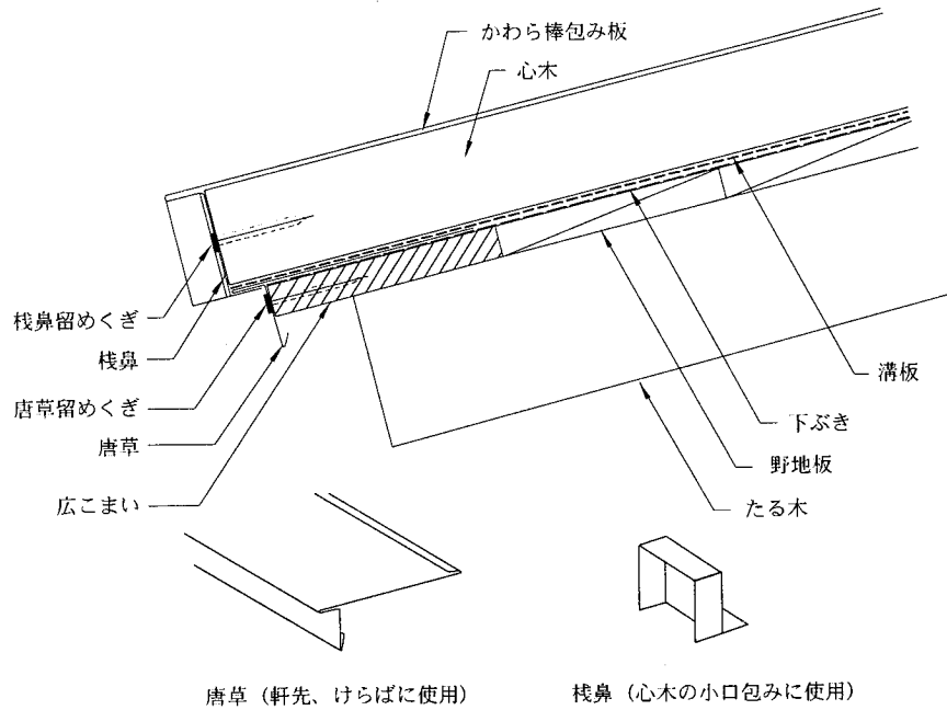
参考図 6.2.9 軒部の納り
