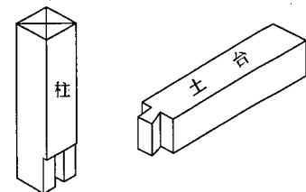
参考図 5.1.3 柱と土台の仕口 (落しあり)
