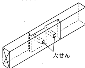
参考図 5.1.5 胴差の継手 (追掛け大せん継ぎ)
