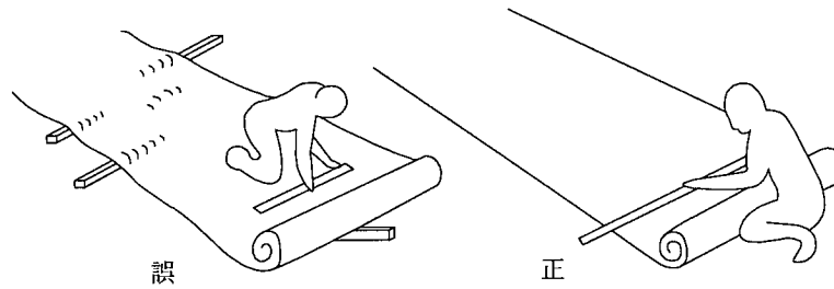
参考図 7.5.1 防湿材の加工（床を清掃し踏みつけない。）
