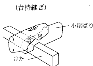
参考図 5.5.1-2 小屋ばりの継手
