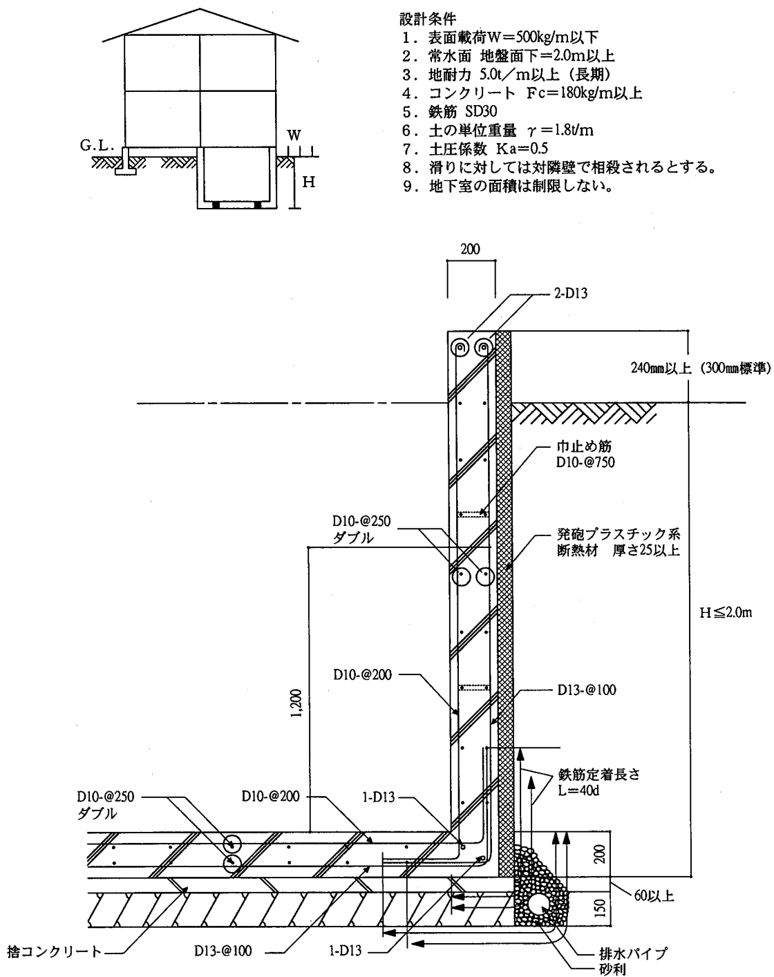
参考図 3.4.2 基礎 壁
