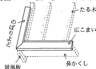
参考図 5.7.3 広こまい・のぼりよど
