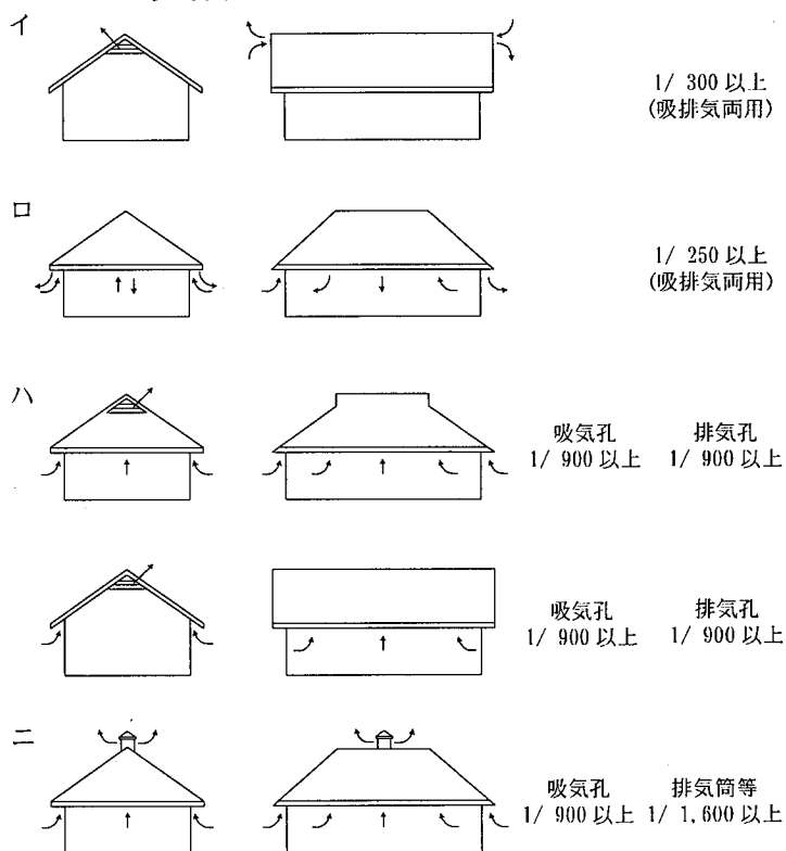
参考図 8.8.1 小屋裏換気孔の取り方例
