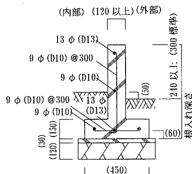
イ. 標準配筋図
