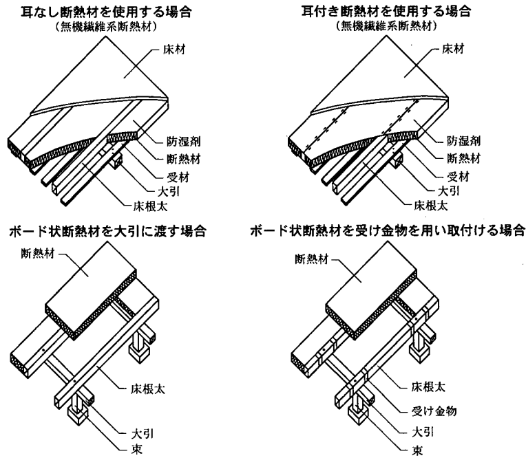
参考図 7.6.3 床の断熱材施工例
