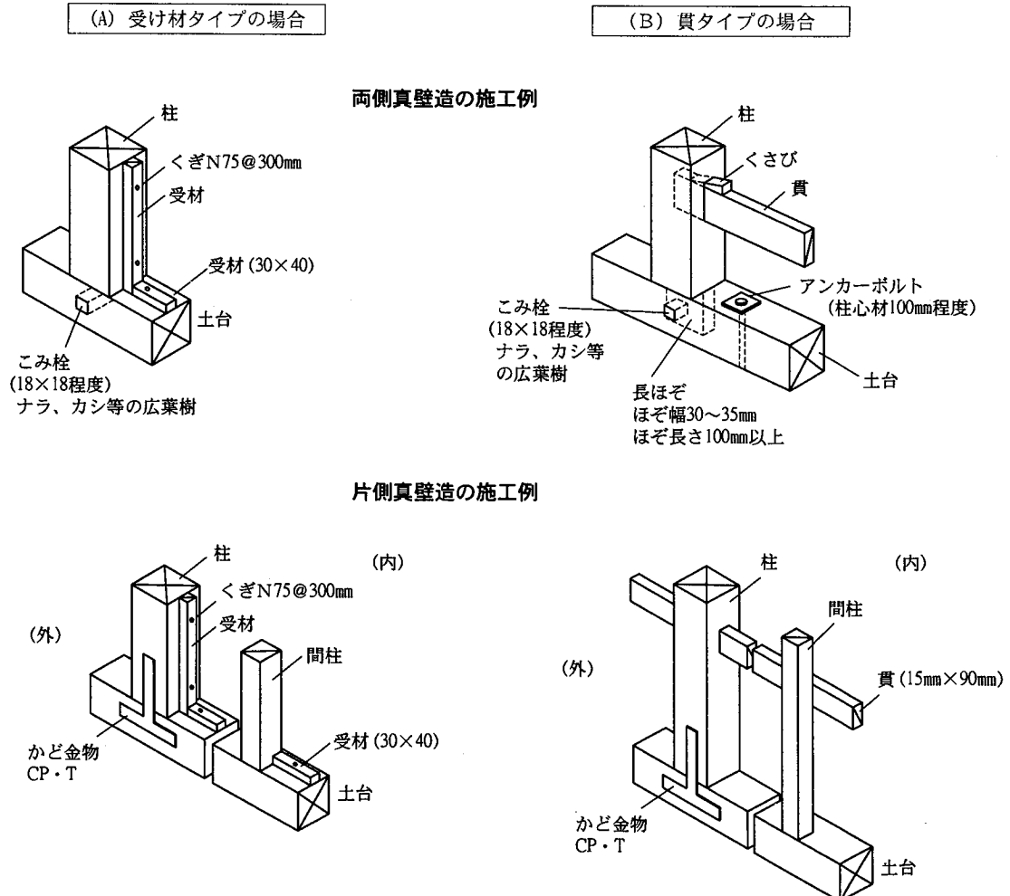
参考図 5.4 真壁造における構造用面材の張り方
