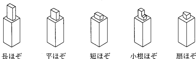
長ほぞ
