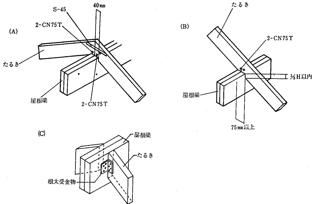
4.10—15図 屋根梁とたるき接合
