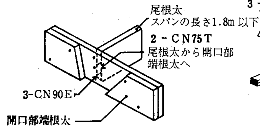
4.5-7 図 尾根太の釘打ち
