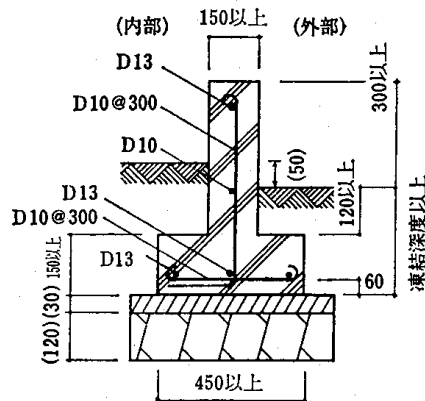
3.5—1 図 3階建の布基礎詳細
