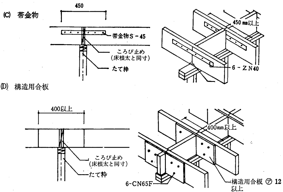
4.5-3 図 端根太と側根太又は床根太との仕口
