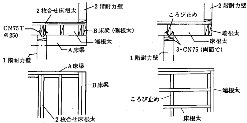
4.5-12図 隅角部の補強
