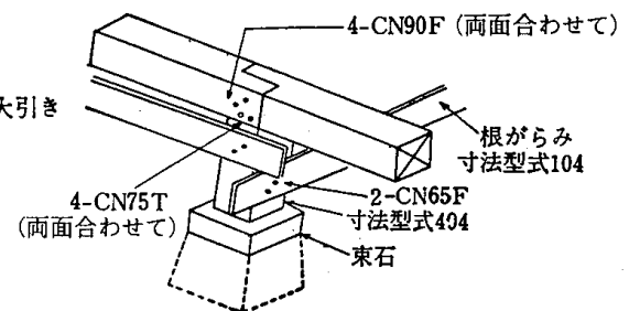
4.4-4 図 大引きの継手
