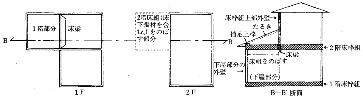
4.5—14図 床枠組の構成（床梁を設ける場合）
