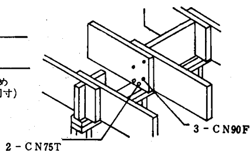
4.5—2図 床根太の継手
