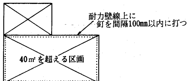
4.5—24図 「 40\text{m}^2 を超える区画」の床下張り
