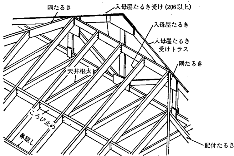
4.10—21図 入母屋の構成図
