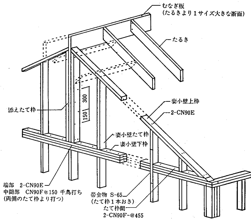
4.10—6 図 むなぎの支持
