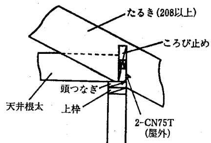
4.10-12図 たるきのころび止め
