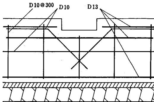
(B) 換気口廻りの補強
