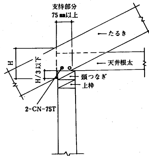
4.10-8 図 たるきのおさまり
