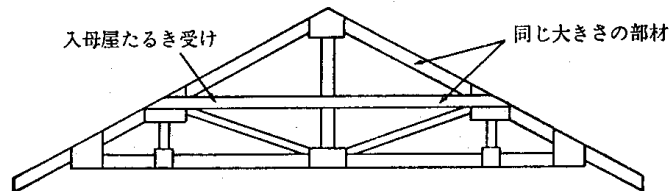
4.10—20図 入母屋たるき受けトラス
