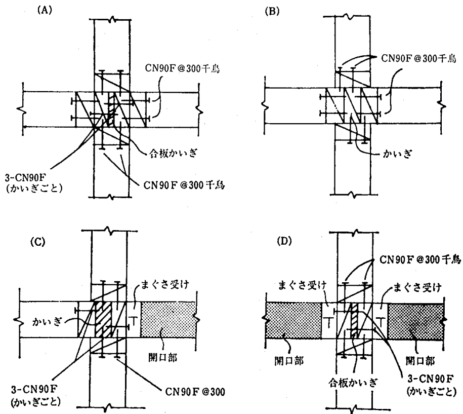
4.7—5 図 耐力壁が十字壁に接合する場合の隅柱の構成
