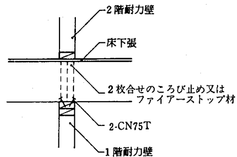
4.5—24図 「 40\text{m}^2 を超える区画」の床下張り
