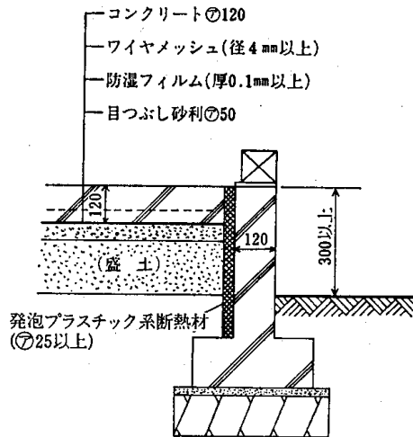
3.4—4 図 土間コンクリート床
