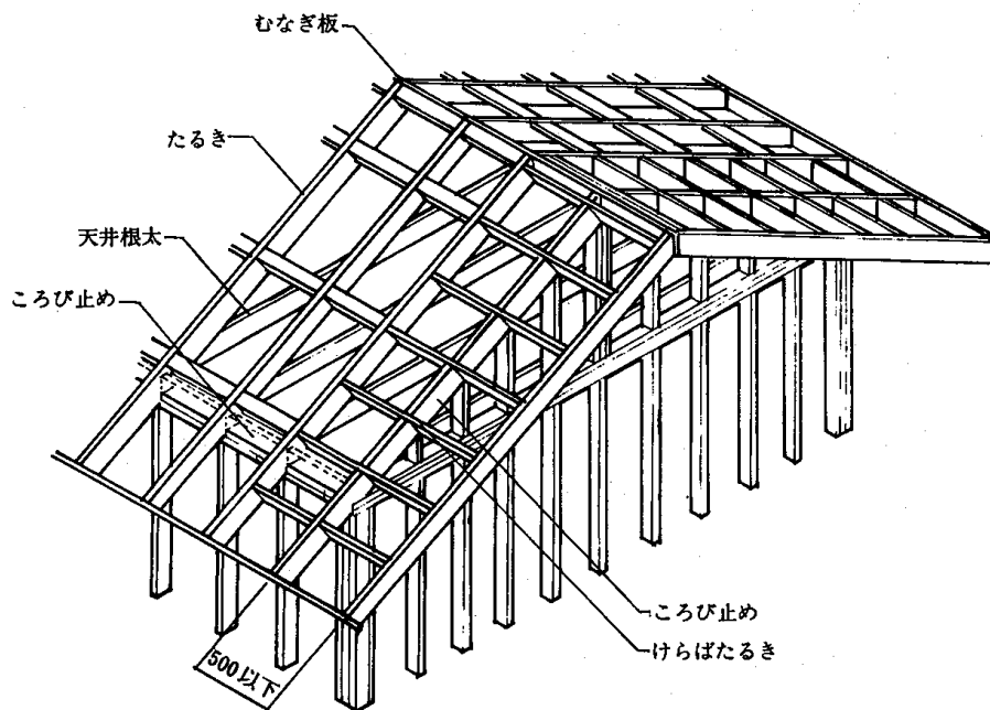
4.10-10 図 軒のはりだし方
