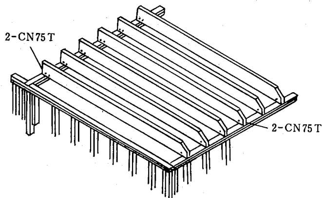
4.10—2図 天井根太と頭つなぎの釘打ち
