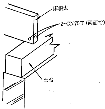
4.5—1図 床根太と土台と釘打ち
