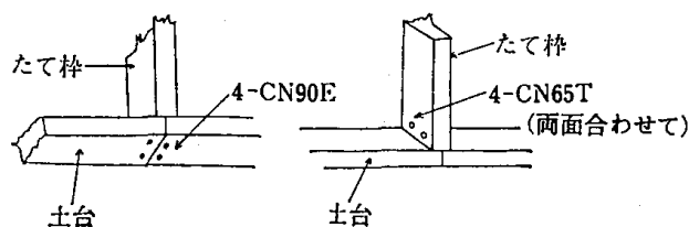
4.4-6 図 土台を下枠として使用する場合の継手
