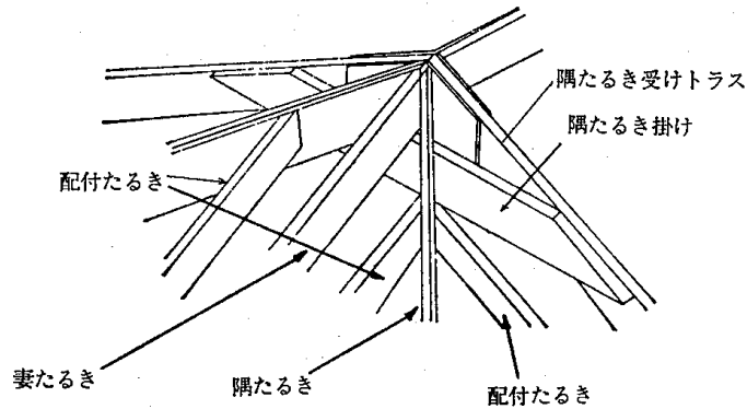
4.10—17図 寄棟部分の構成
