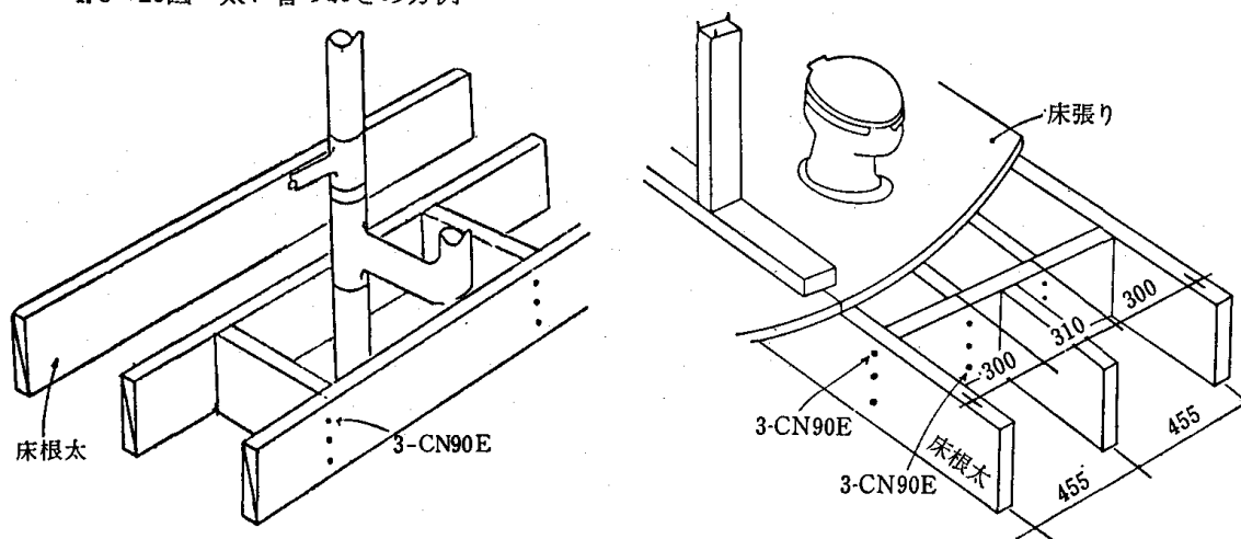
4.5—20図 太い管のおさめ方例
