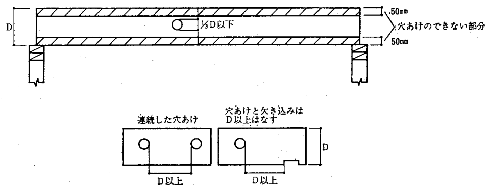
4.5—19図 床根太の穴あけの制限
