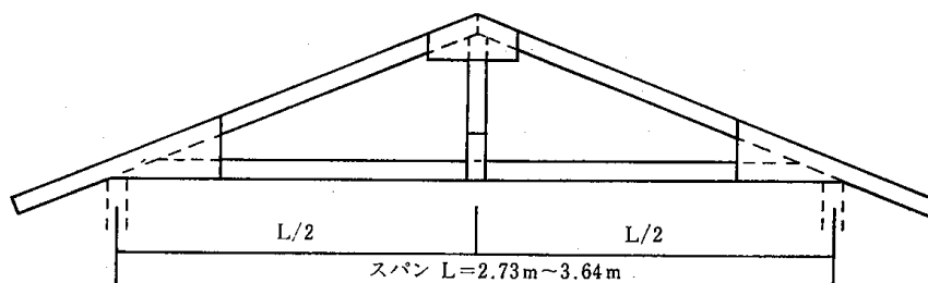
4.10—16図 トラスの種類
