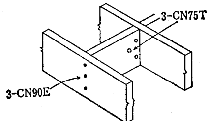
4.5-5 図 床根太と同寸法によるころび止め
