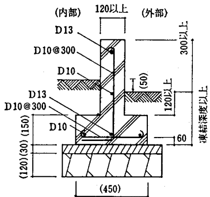
(A) 標準配筋図(mm)
