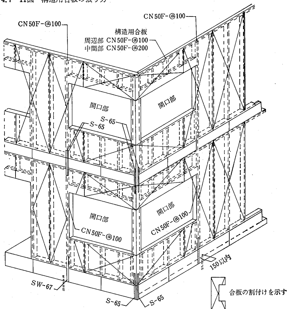
4.7-11図 構造用合板の張り方
