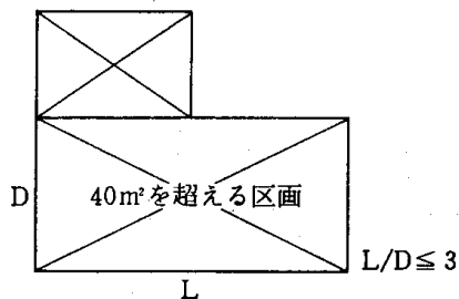
4.5—22図 40\text{m}^2 を超える区画の形状比
