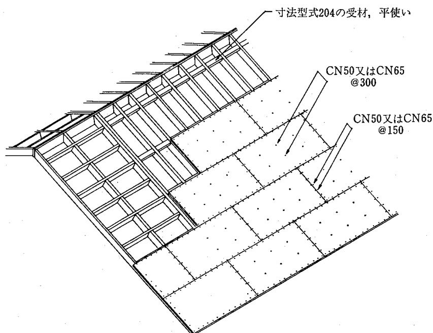
4.10—30図 屋根下張りの釘打ち
