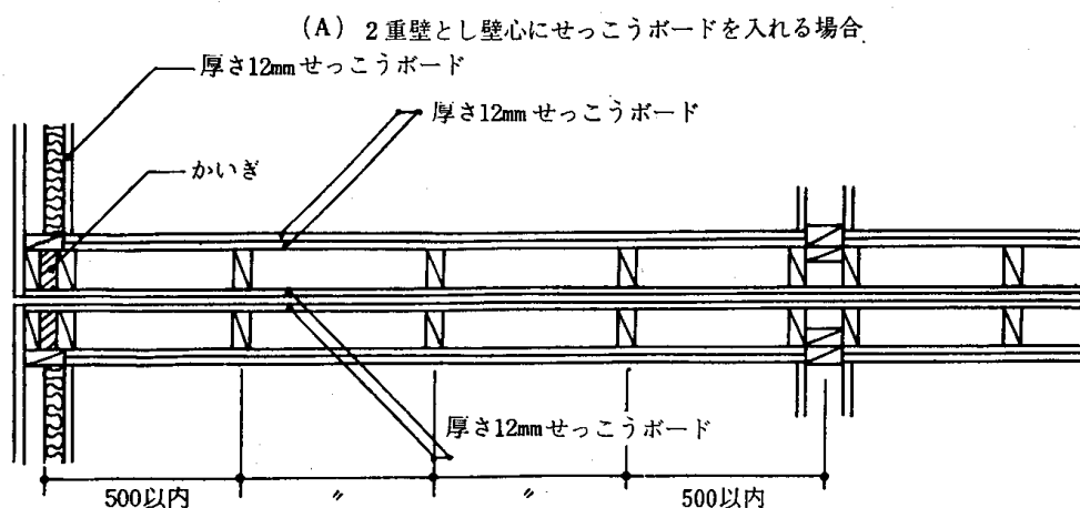
4.7-21図 連続建の住戸間界壁
