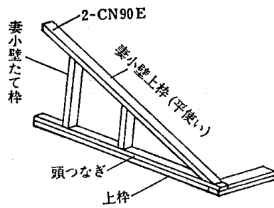
4.10—5 図 妻小壁
