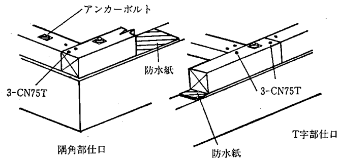
4.4-1 図 寸法型式 404 の土台の仕口及び継手の釘打ち
