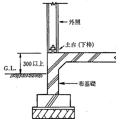
3.4—5 図 床と一体の布基礎
