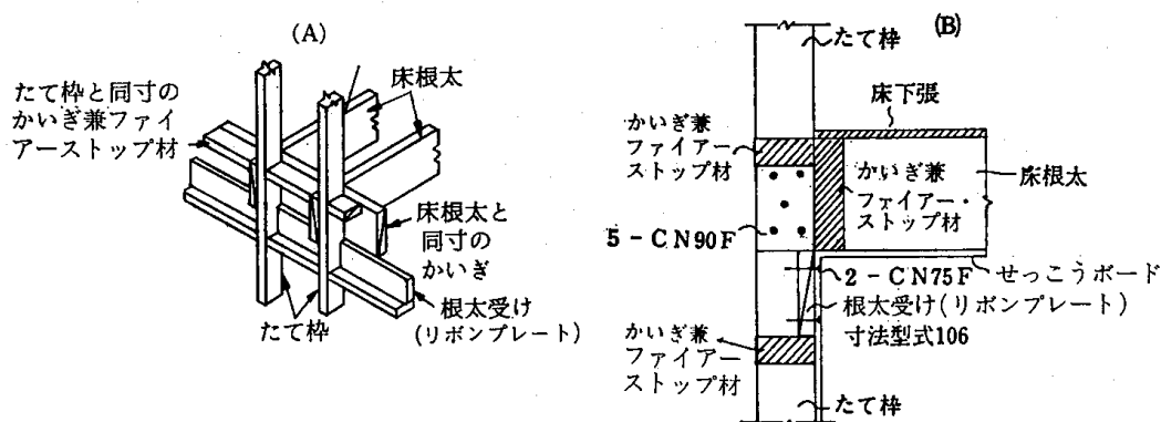
4.7-20図 スキップフロアの構成例
