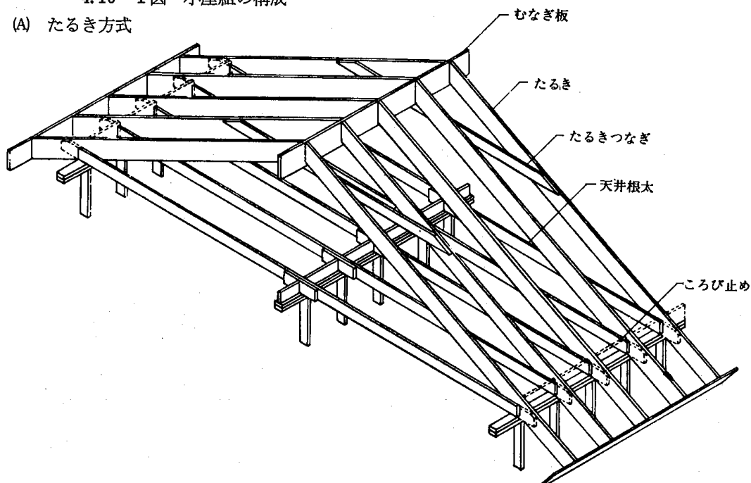
4.10-1図 小屋組の構成
