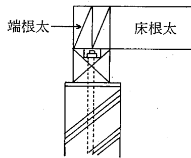
4.4-2 図 座金ぼり
