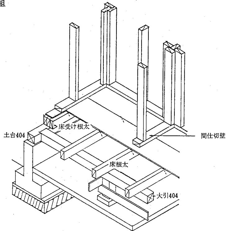
4.4—5 図 化粧を施した構造用合板による床組
