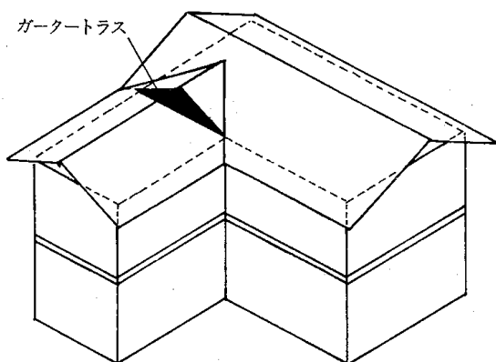
4.10—27図 L字屋根
