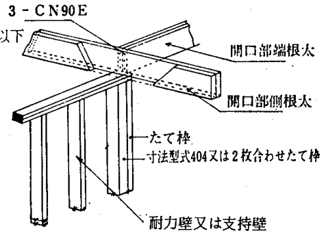
4.5-8 図 開口部端根太端部の支持
