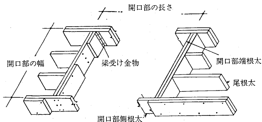
4.5—6図 床開口部回りの補強
