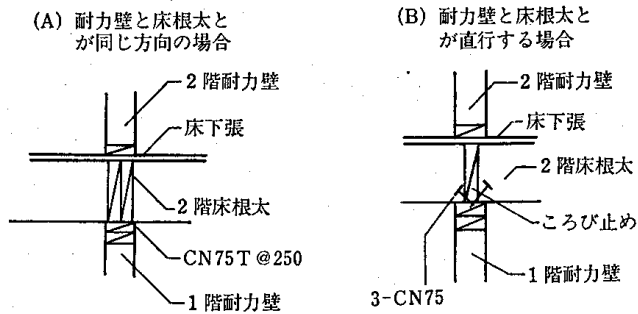
4.5-10図 2階耐力壁下部の補強
