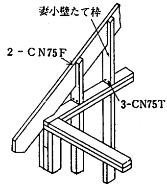
4.10—4 図 妻小壁たて枠
