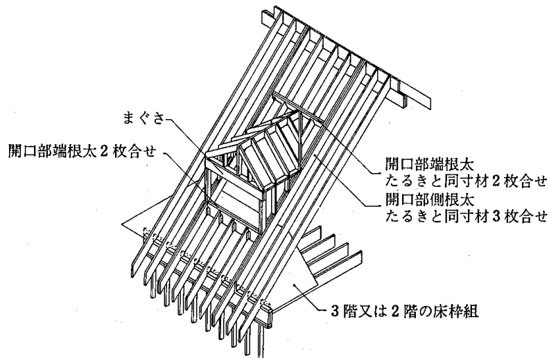
4.10—29図 屋根開口部のとり方
