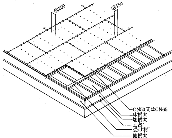
4.5—21図 床下張材の張り方と釘打ち
