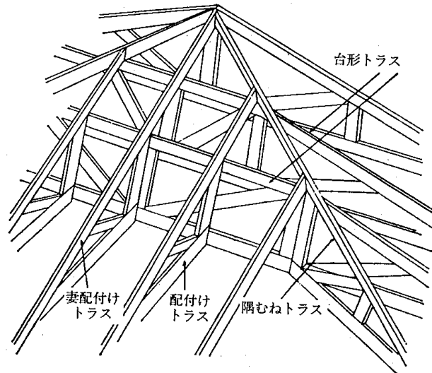
4.10—19図 トラスによる寄棟のおさまり例
