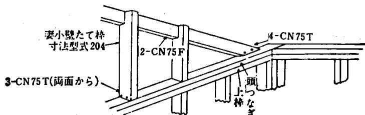
4.10-23図 妻小壁の詳細
