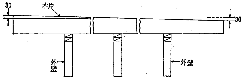
4.10—24図 陸屋根の勾配のとり方
