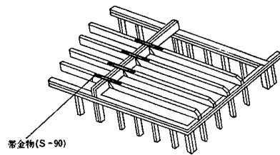
4.10—3 図 梁への接合例
