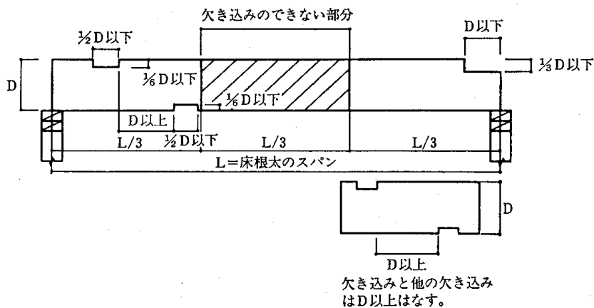
4.5—18図 床根太の欠き込みの制限
