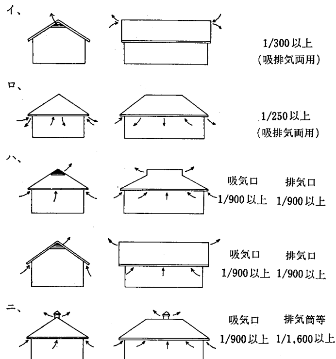
4.11-1 図 換気口の取り方例
