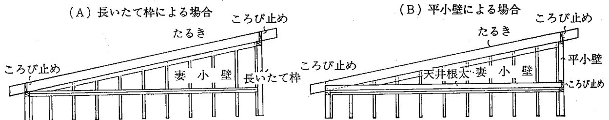
4.10-22図 片流れ屋根の構成
