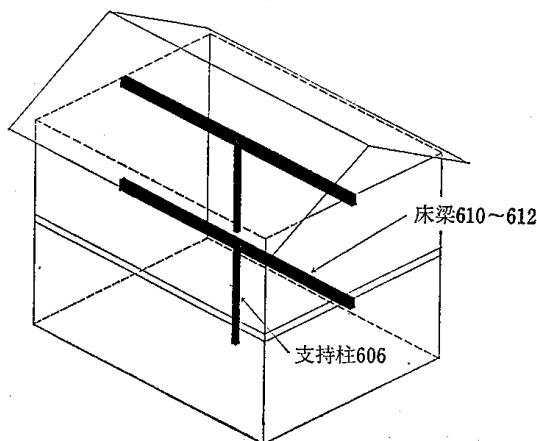
4.8-1図 支持柱
