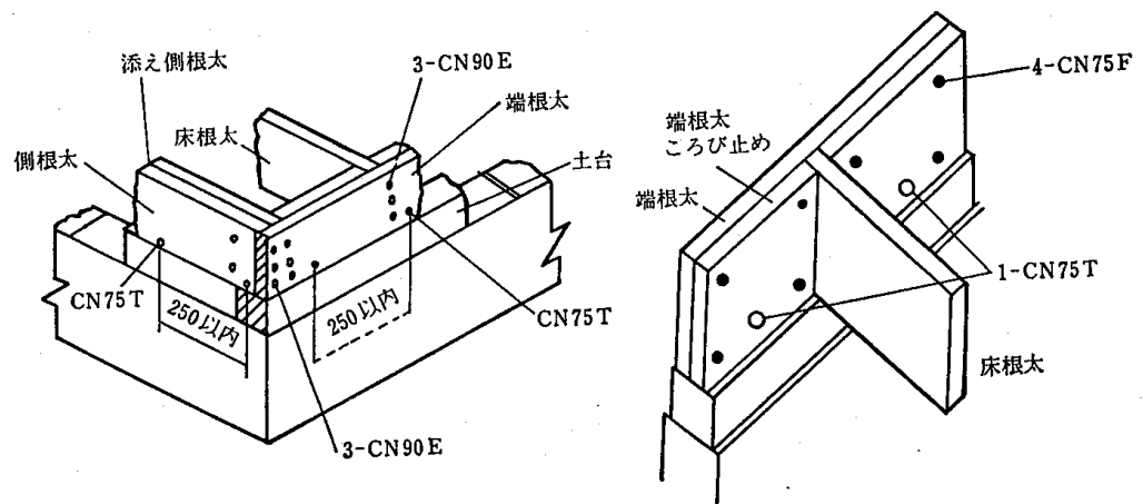
4.5-5 図 床根太と同寸法によるころび止め
