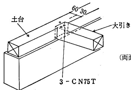
4.4-3 図 土台と大引きの取合
