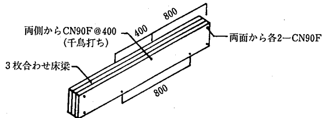
4.5-15図 合わせ床梁のつくり方
