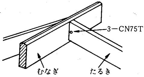
4.10-7 図 むなぎとたるきの仕口
