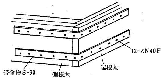
4.5-12図 隅角部の補強
