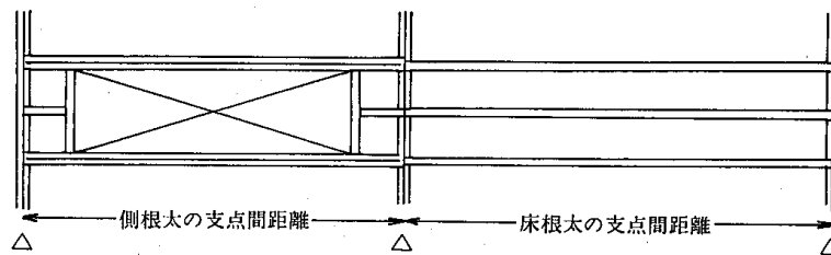
4.5-9 図 側根太の支点間距離のとり方
