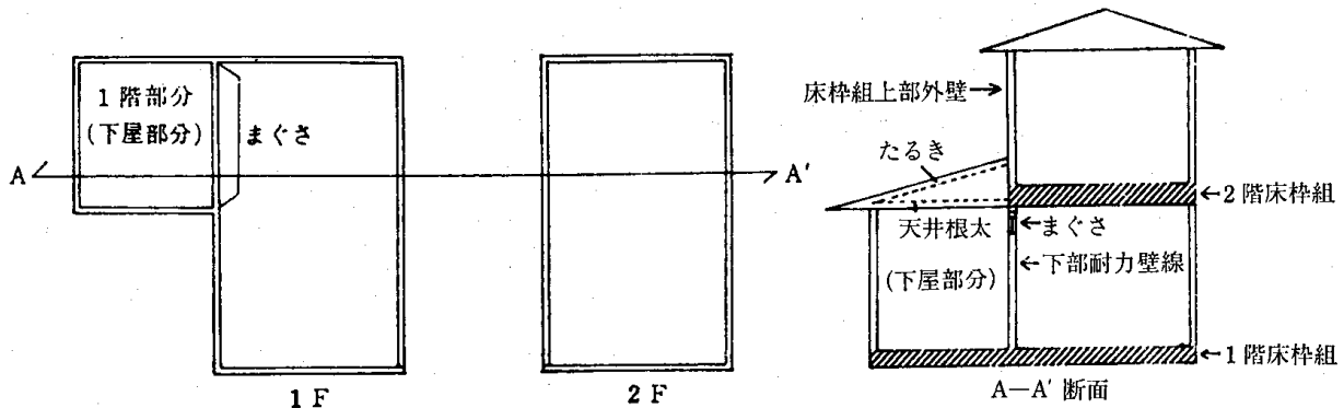
4.5-13図 床枠組等の構成 (下部に耐力壁を設ける場合)
