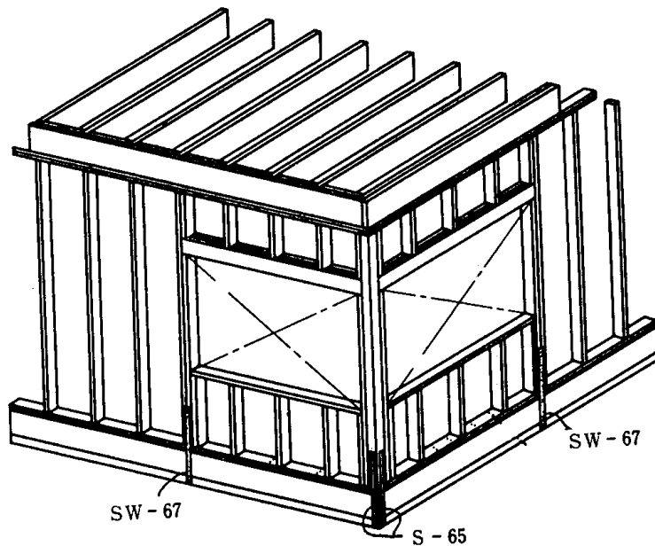
4.7-12図 両面開口部詳細
