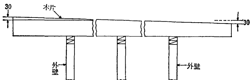
4.10—24図 陸屋根の勾配のとり方
