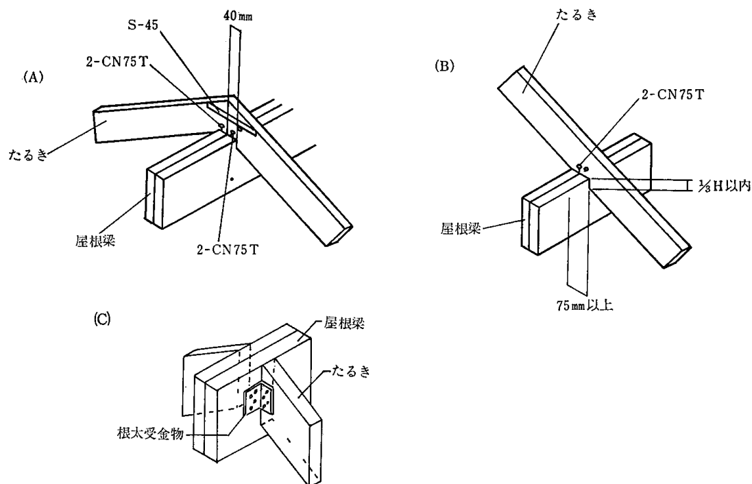
4.10—15図 屋根梁とたるき接合
