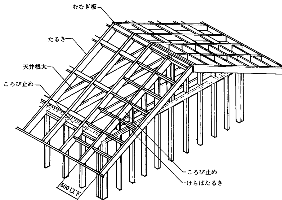
4.10—10図 軒のはりだし方
