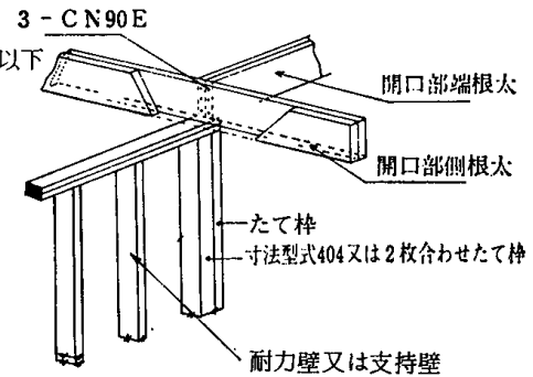
4.5-8 図 開口部端根太端部の支持
