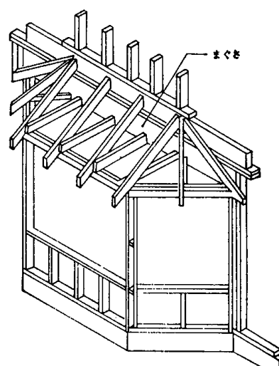
4.7—10図 出窓などのまぐさの入れ方例
