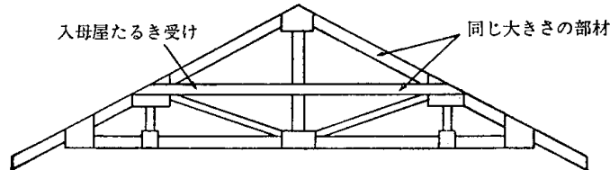
4.10—20図 入母屋たるき受けトラス
