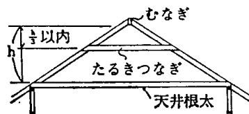
(A) たるきつなぎの取り付け方
