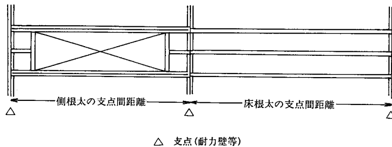
4.5-9 図 側根太の支点間距離のとり方
