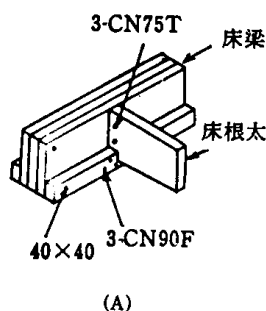
4.5—17図 根太がけの方法と釘打ち
