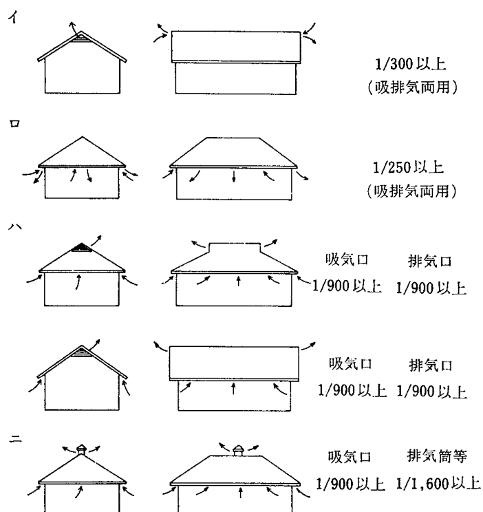
4.11-1 図 換気口の取り方例
