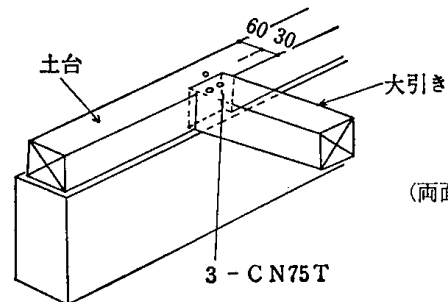
4.4-3 図 土台と大引きの取合
