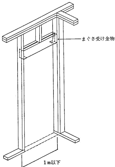
(A)図 まぐさ受け金物の使用例
