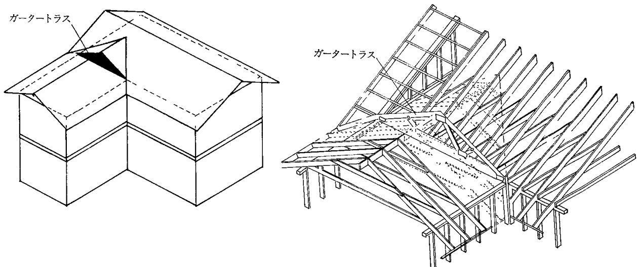
4.10—27図 L字屋根
