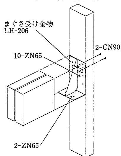
(C)図 金物の取付け方
