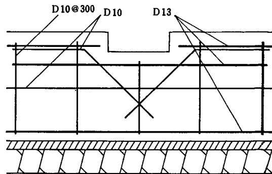
(B) 換気口廻りの補強
