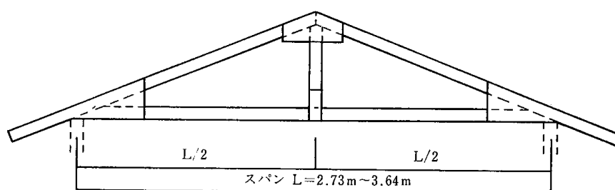
4.10—16図 トラスの種類
