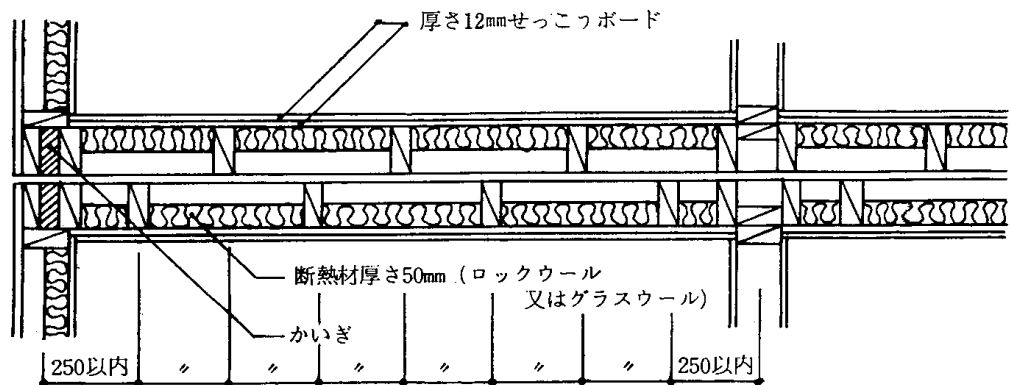
(B) 2重壁とし壁心にせっこボードを入れない場合
