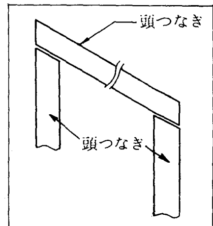
(C) 頭つなぎの納め方
