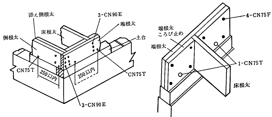
4.5—5 図 床根太と同寸法によるころび止め
