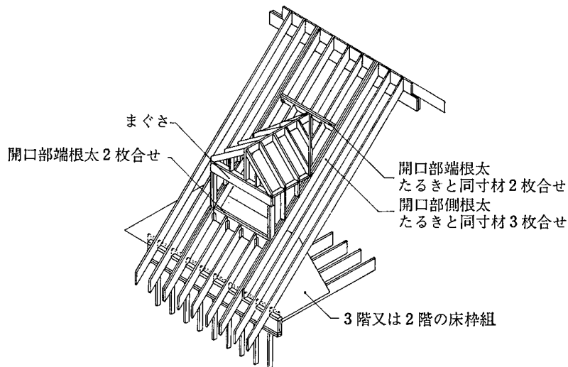
4.10—29図 屋根開口部のとり方
