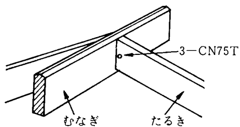
4.10—7図 むなぎとたるきの仕口
