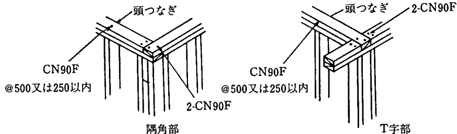
4.7-2 図 頭つなぎ釘打ち
