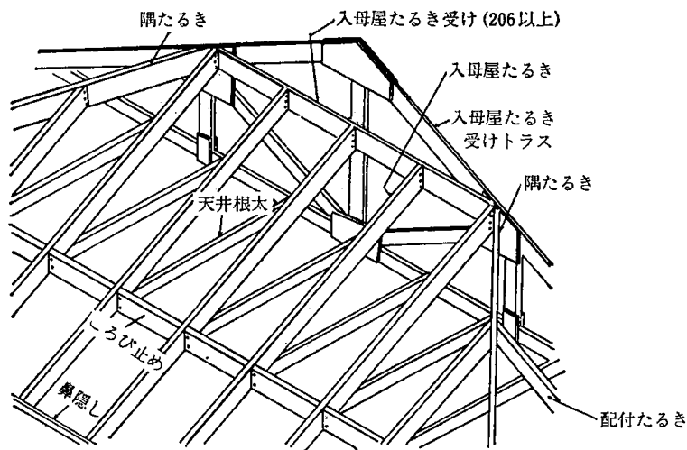
4.10—21図 入母屋の構成図
