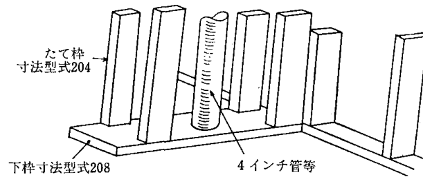
4.7—17図 太い管を壁中に配する方法例
