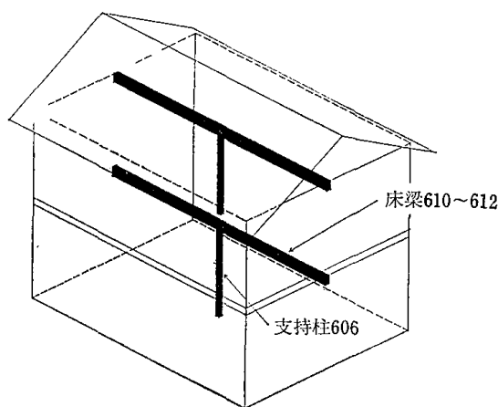
4.8—1図 支持柱
