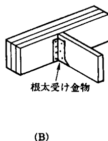
4.5—17図 根太がけの方法と釘打ち
