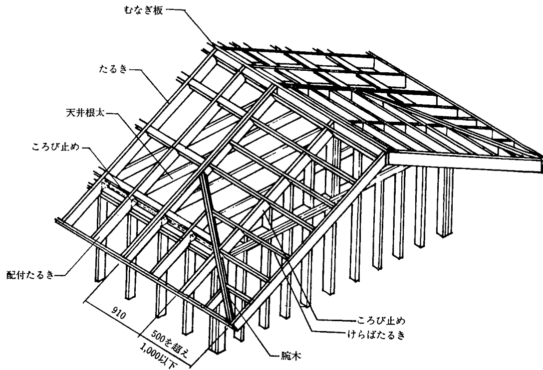
(B) けらばの出が1.0m 以下
