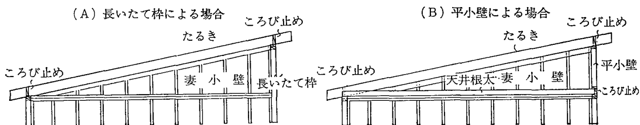
4.10—22図 片流れ屋根の構成
