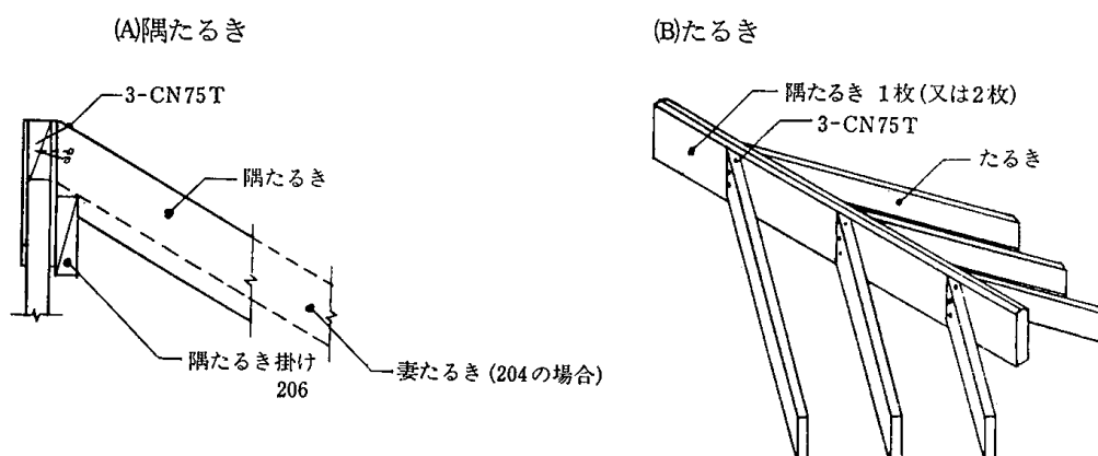
4.10—18図 寄棟部分のおさまり
