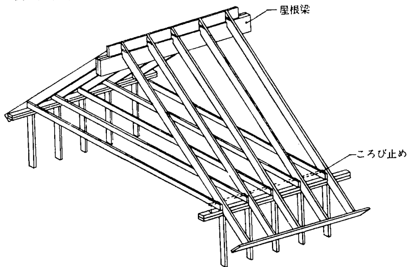
(B) 屋根梁方式
