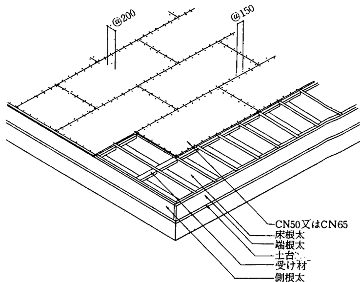
4.5—21図 床下張材の張り方と釘打ち
