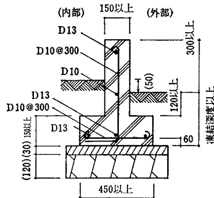
3.5—1 図 3階建の布基礎詳細
