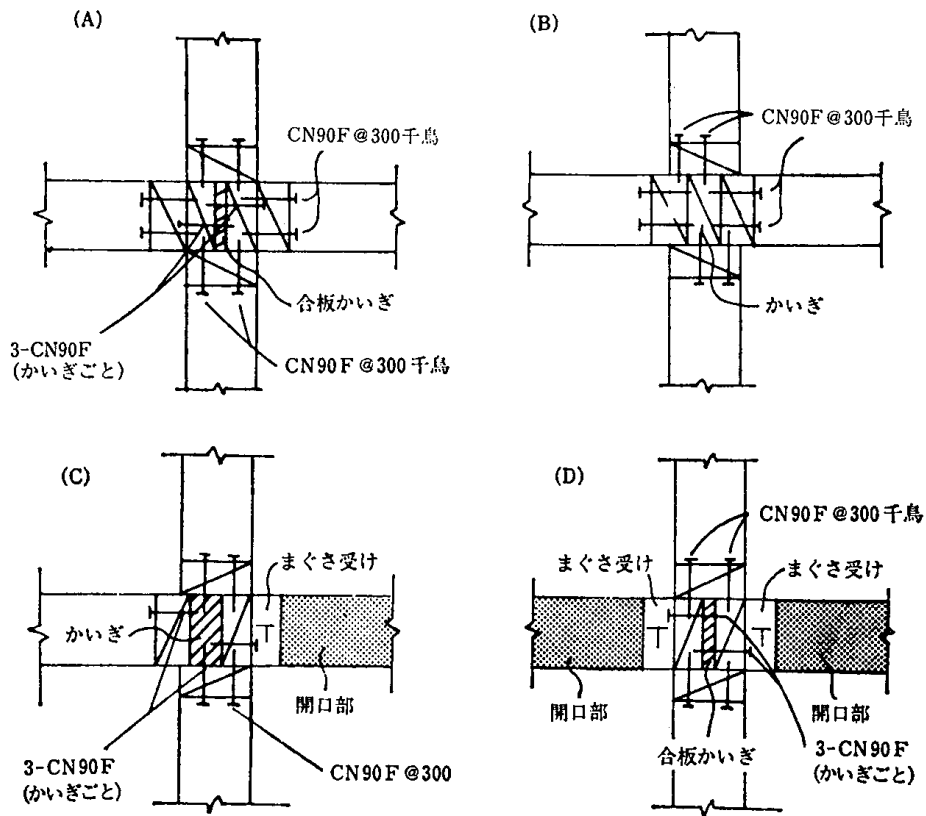
4.7-5 図 耐力壁が十字壁に接合する場合の隅柱の構成
