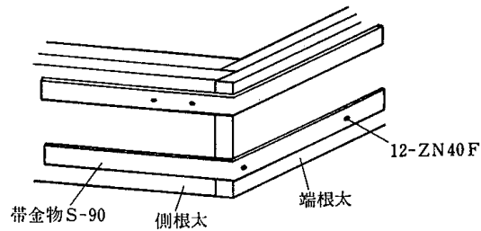
4.5—12図 隅角部の補強
