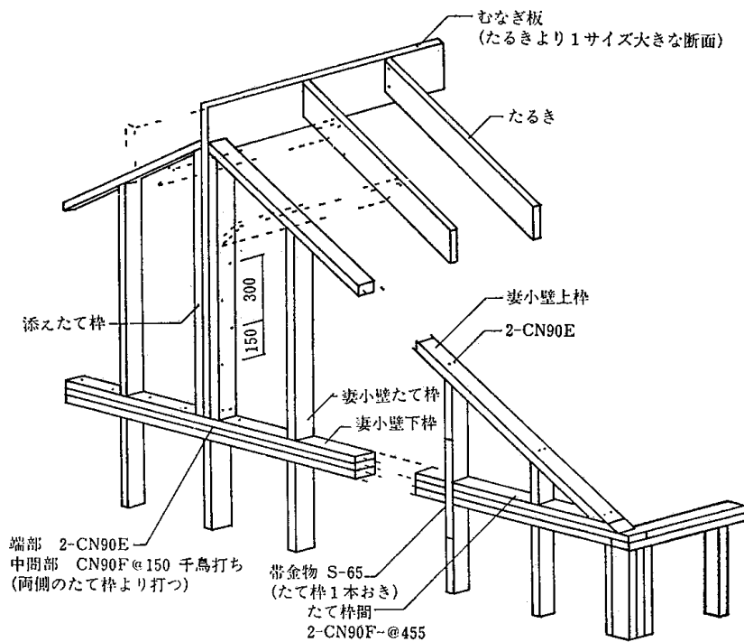
4.10—6 図 むなぎの支持
