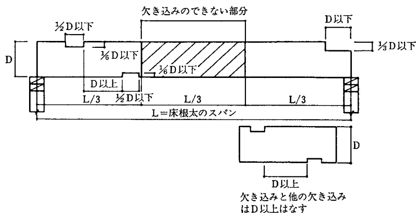
4.5—18図 床根太の欠き込みの制限
