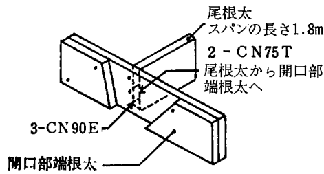
4.5-7 図 尾根太の釘打ち
