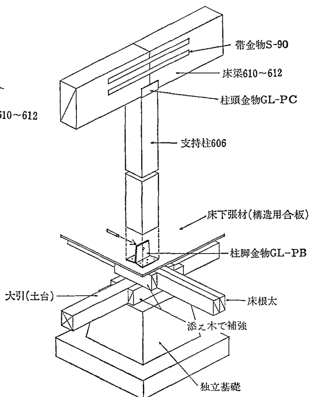
4.8—2図 支持柱と梁及び床との納まり
