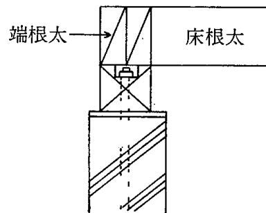
4.4-2 図 座金ぼり
