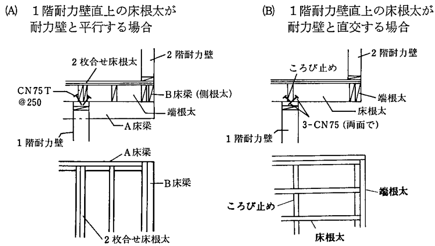
4.5—11☒ オーバーハングした場合の床枠組と壁枠組の緊結
