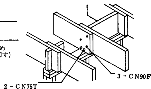
4.5—2 図 床根太の継手
