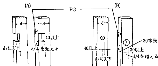
4.7—15図 たて枠の欠き込みと穴あけ
