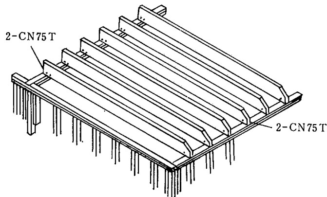
4.10—2 図 天井根太と頭つなぎの釘打ち
