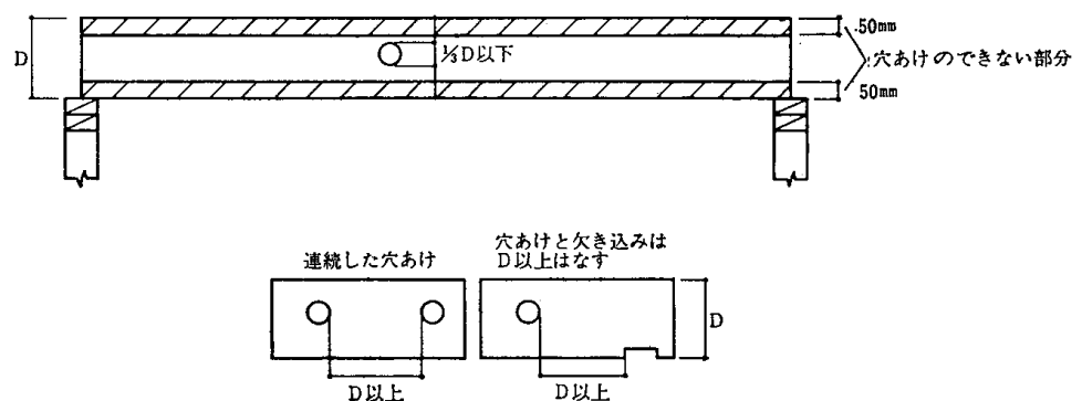
4.5—19図 床根太の穴あけの制限
