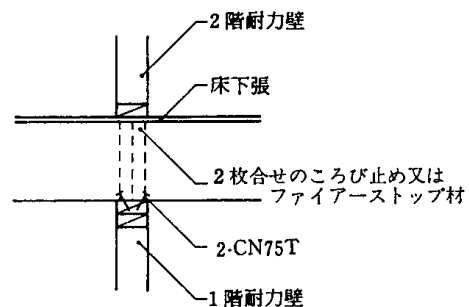
4.5—24図 「 40\text{m}^2 を超える区画」の床下張り
