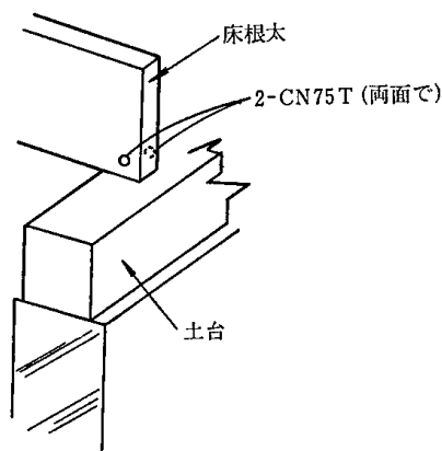
4.5—1 図 床根太と土台と釘打ち
