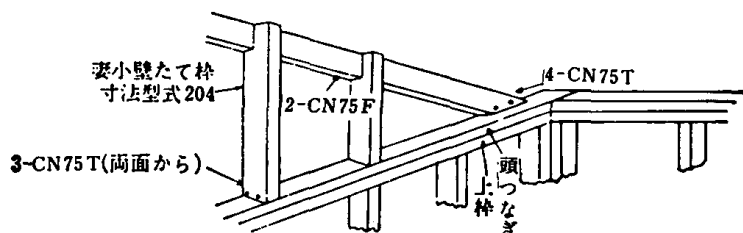
4.10—23図 妻小壁の詳細
