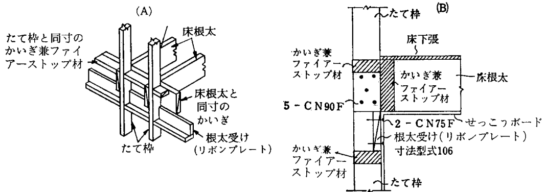
4.7-20図 スキップフロアの構成例
