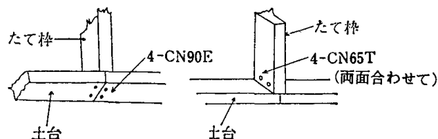
4.4—6 図 土台を下枠として使用する場合の継手
