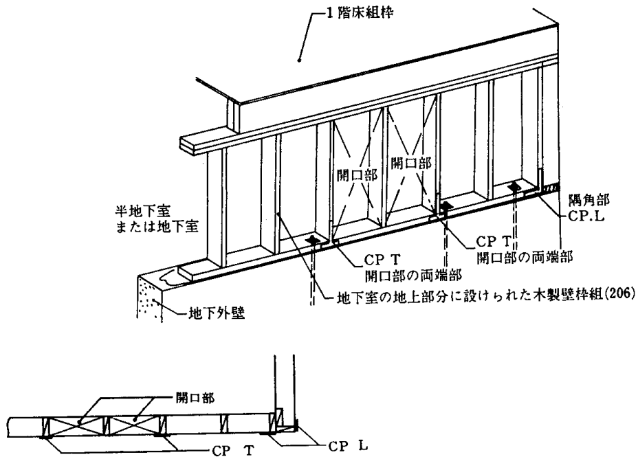
3.3-3 図 木造の壁の構成 (A) 隅角部及び開口部両端部の補強
