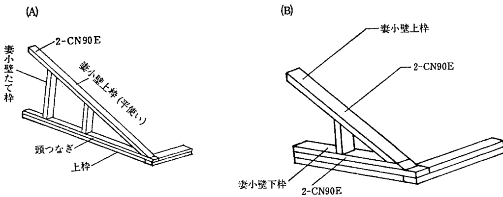
4.10—5 図 妻小壁
