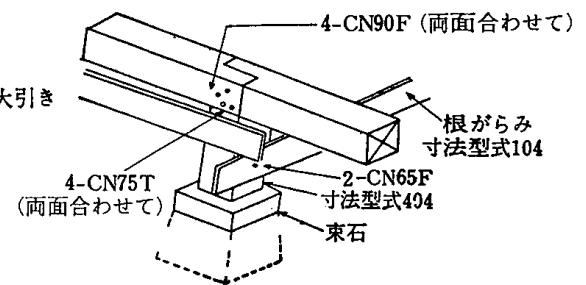
4.4-4 図 大引きの継手
