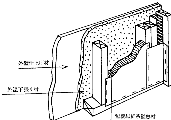
8.6—4 図 壁の断熱材の施工例
