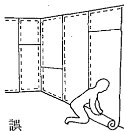
防湿材の施工（防湿層は寸法の大きいものを用いる）
