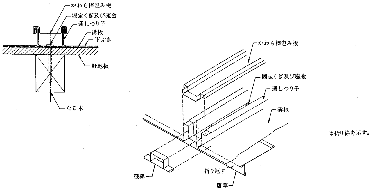
参考図 5.2.8 かわら棒ぶきの工法 (心木なしの場合)
