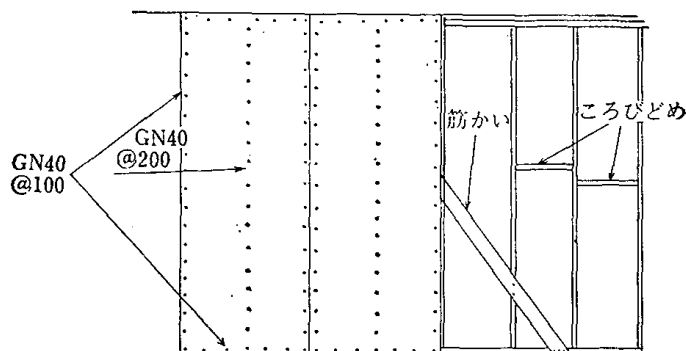
9.6—4図 耐力壁のせっこうボードの釘打ち
