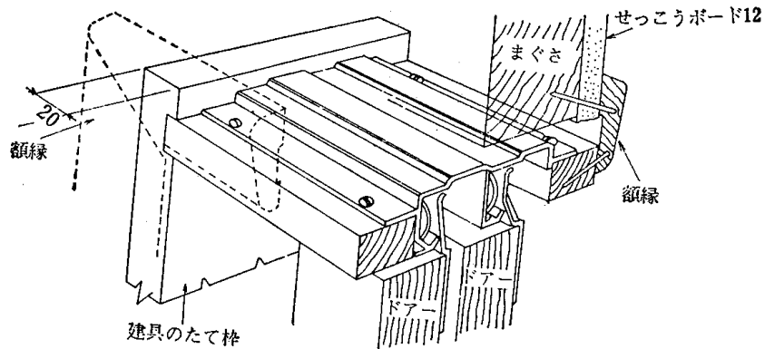
10.6-1 図 枠付き引違い戸
