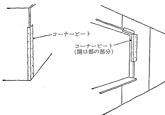
9.6—6図 コーナービートの取り付け
