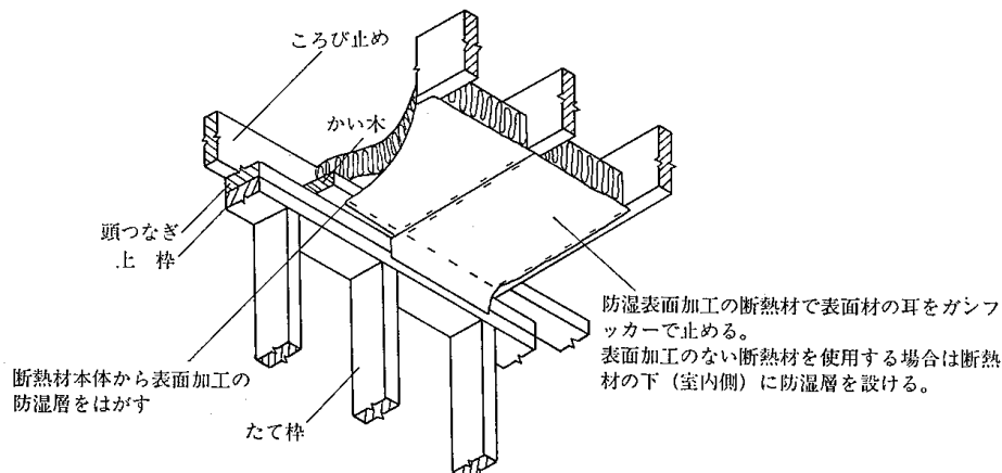
8.6—5 図 天井の断熱材の施工例
