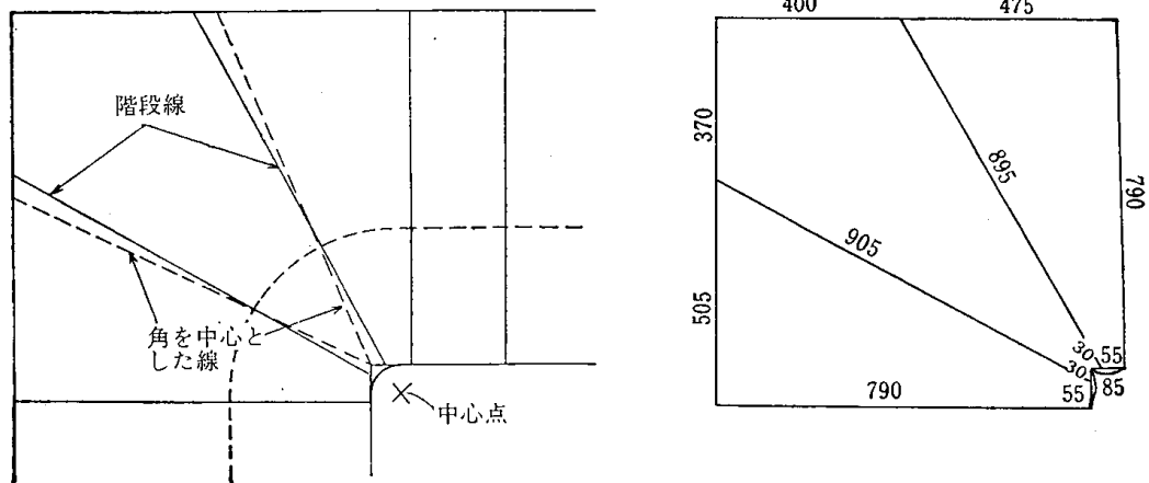
3 図 曲がり階段の形状と寸法
