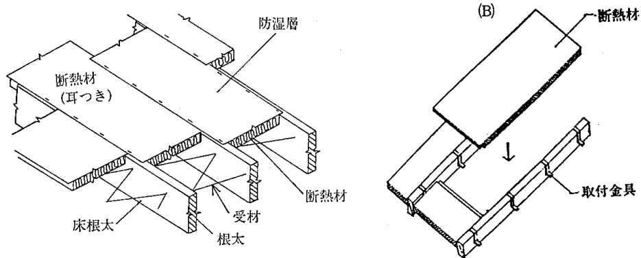
8.6—3 図 床の断熱材の施工例 (A) 耳付きコルツ状断熱材 (B) ボード状断熱材
