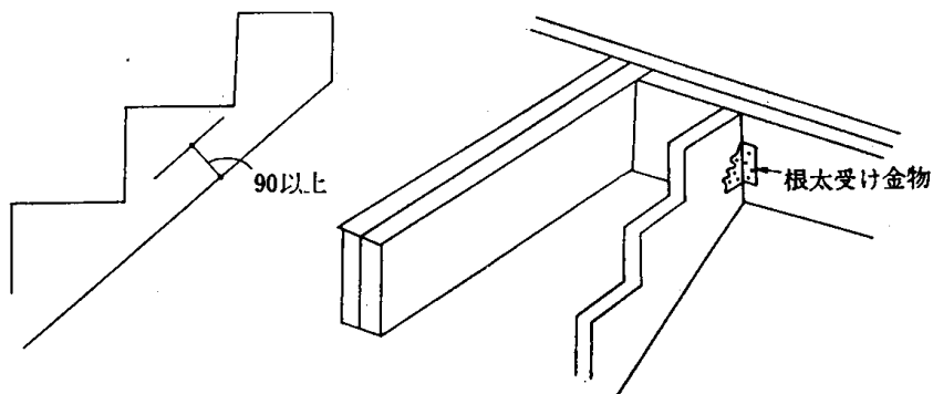
10.7-1 図 寸法型式210によるささら桁
