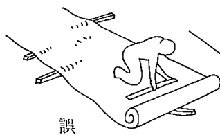
誤正防湿層の加工（床を清掃し踏みつけない）
