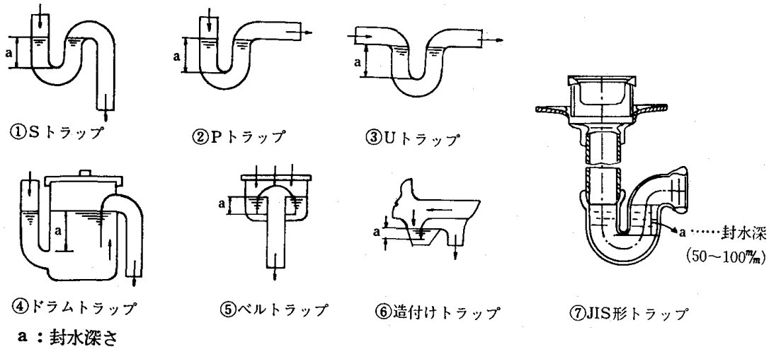
参考図 トラップの種類
