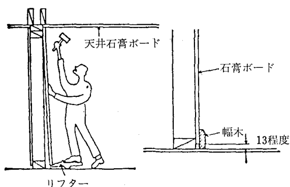
9.6—5図 壁せっこうボードのはり方とおさまり
