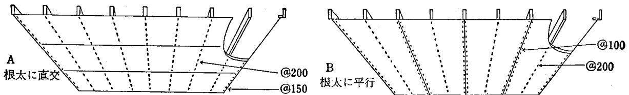
9.6—3 図 天井せっこうボードの張り方
