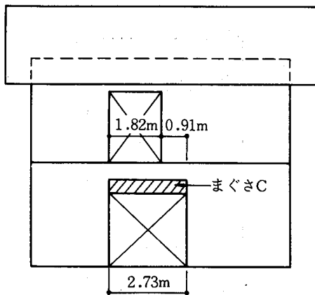
47表 まぐさスパン表⑬ (2階床根太がまぐさCと平行の場合)
