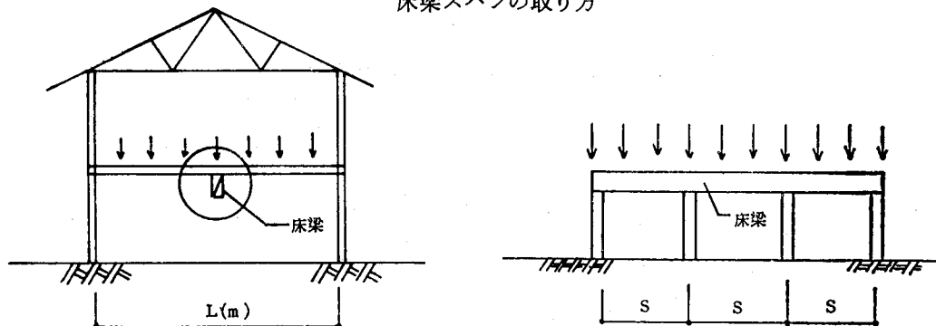
床梁スパンの取り方
