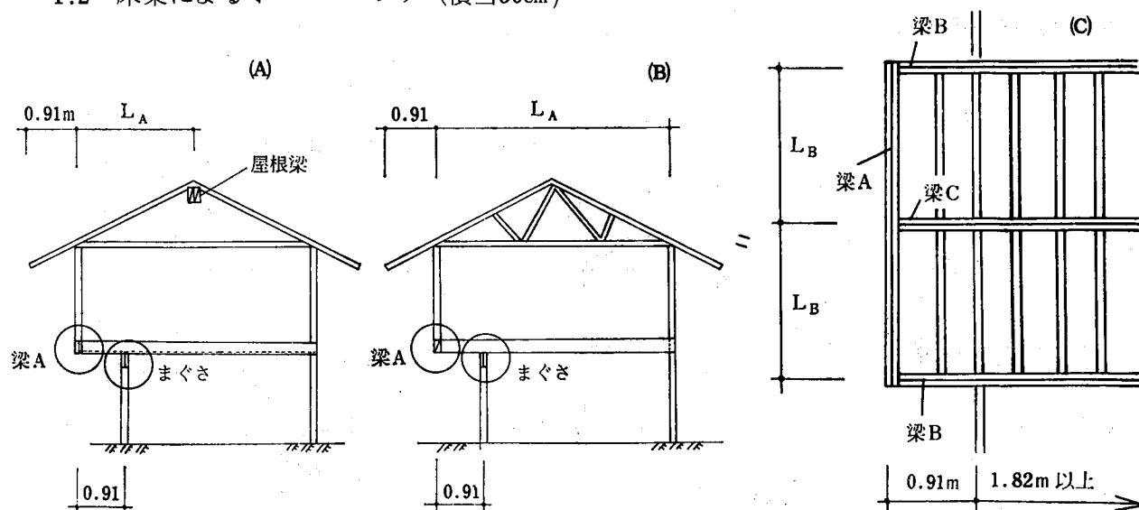
58表 オーバーハング床梁スパン表③
