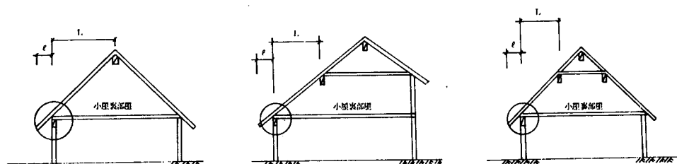
まぐさが支持する屋根荷重幅の取り方
