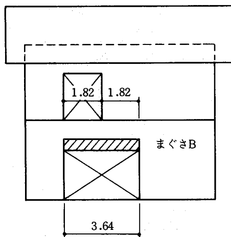
46表 まぐさスパン表⑫ (2階床根太がまぐさBと直交の場合)
