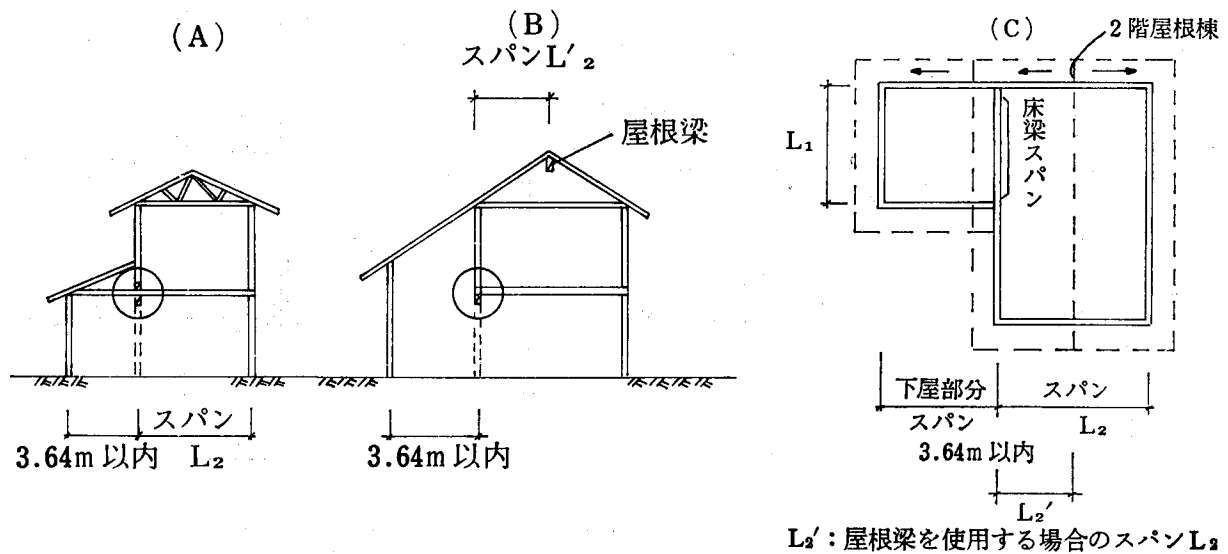
セットバック部分の壁開口位置及び大きさ
