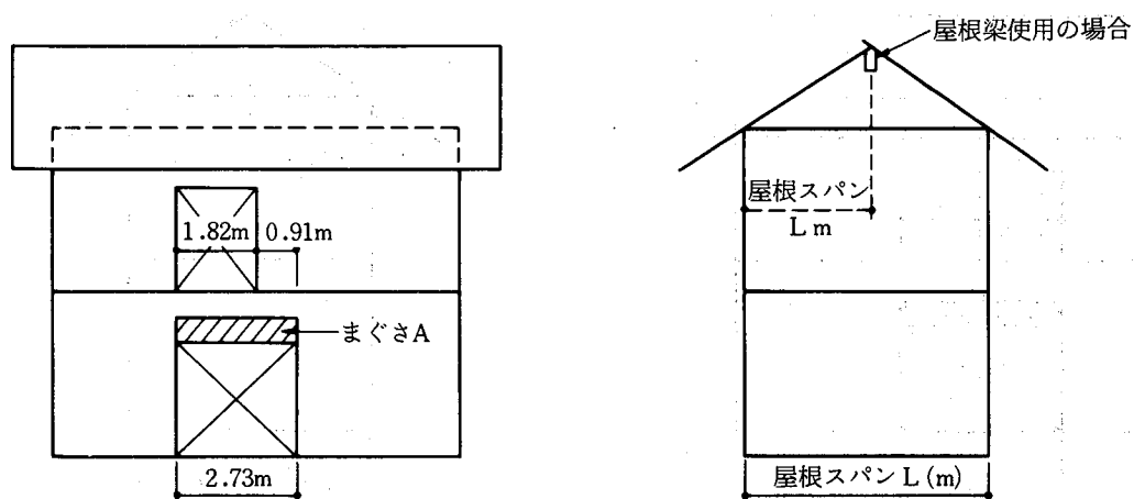
45表 まぐさスパン表⑪ (2階床根太がまぐさAと直交の場合)
