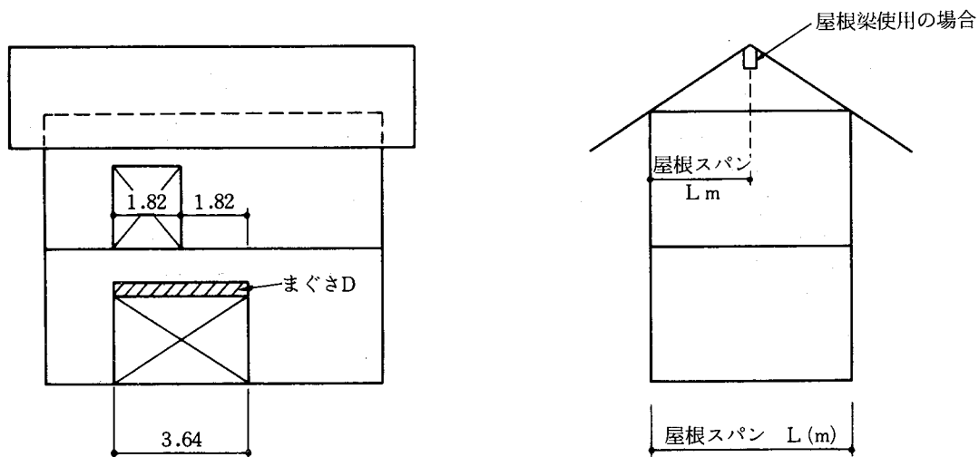
48表 まぐさスパン表⑭ (2階床根太がまぐさDと平行の場合)
