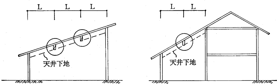
屋根梁間隔の取り方
