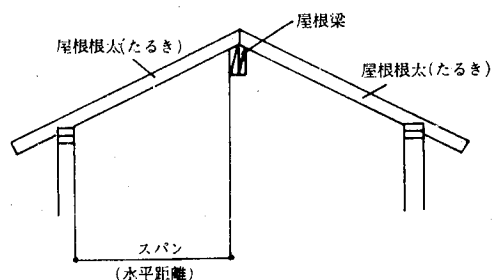
B : 屋根梁方式
