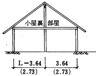
80表 たて枠間隔表③ (L=3.64m、勾配6/10~8/10)
