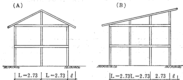
79表 たて枠間隔表② (L=2.73m、勾配5/10以下)
