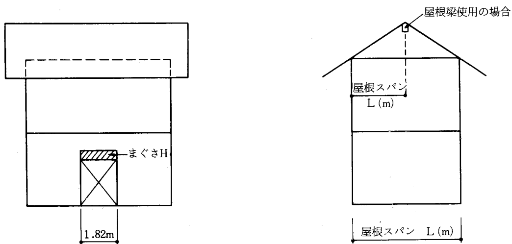
52表 まぐさスパン表⑬ (2階床根太がまぐさHに平行の場合)
