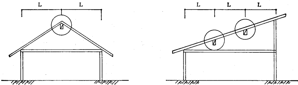
屋根梁間隔の取り方
