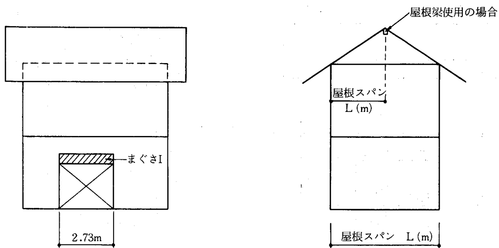
53表 まぐさスパン表⑬ (2階床根太がまぐさ I に平行の場合)
