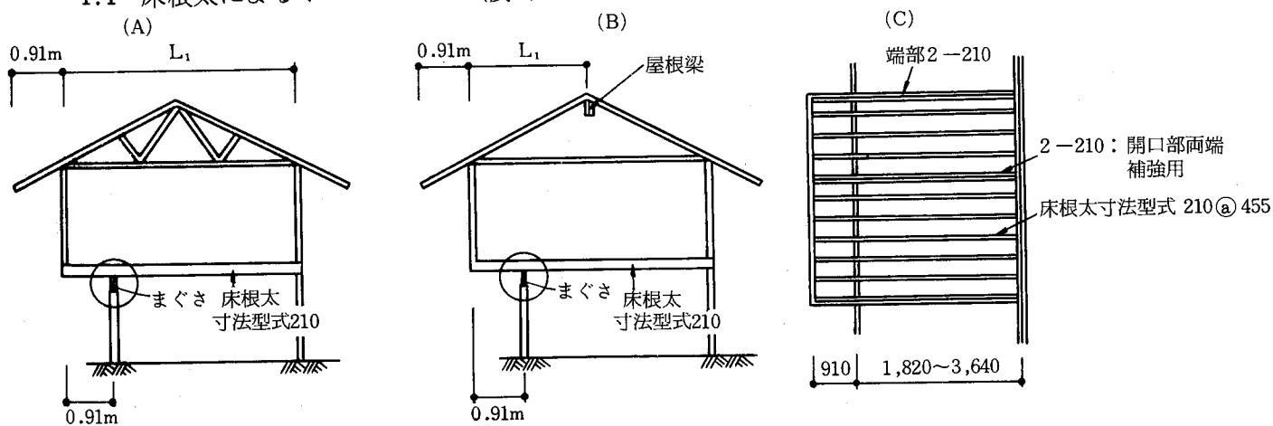
56表 オーバーハング下部の開口部まぐさスパン表① (製材による合わせまぐさ)
