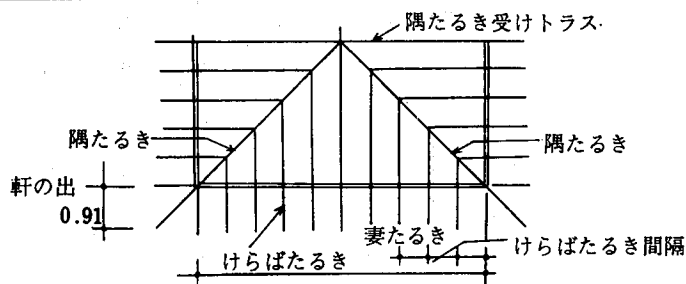
74表 隅たるき受けトラスの使用部材及びガセットへの釘打ち本数表③
