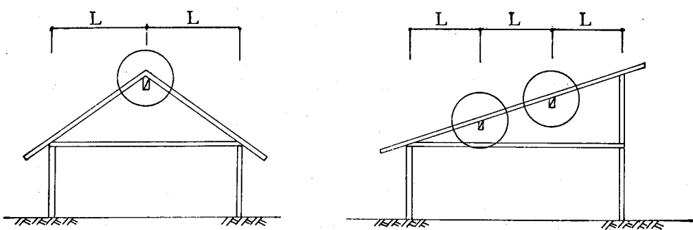
屋根梁間隔の取り方
