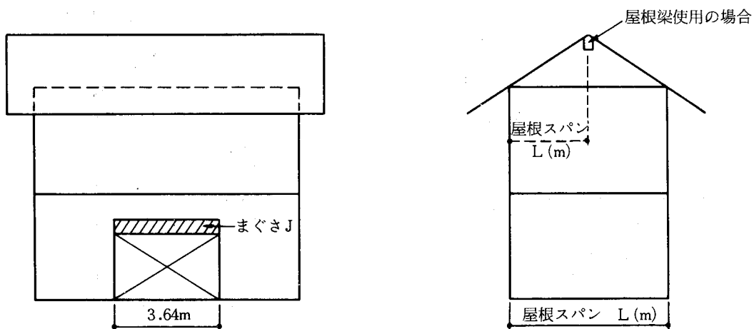
54表 まぐさスパン表② (2階床根太がまぐさ Jに平行の場合)
