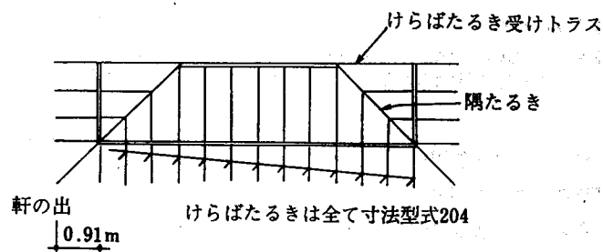
76表 けらばたるき受けトラスの使用部材及びガセットへの釘打ち本数表⑤
