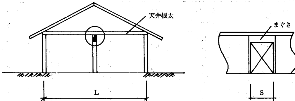
43表 まぐさスパン表⑨
