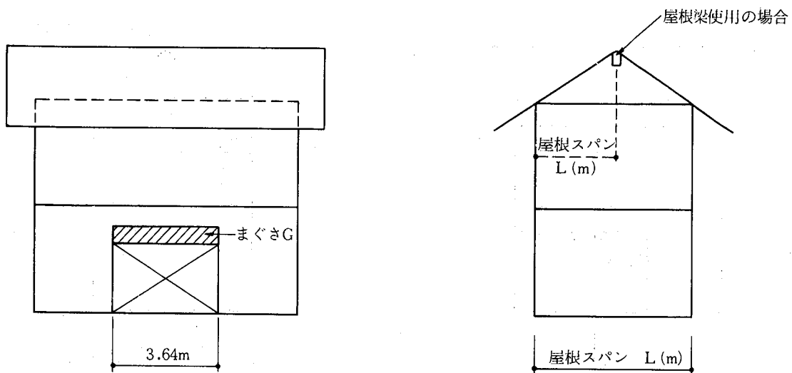
51表 まぐさスパン表①⑦ (2階床根太がまぐさGと直交の場合)
