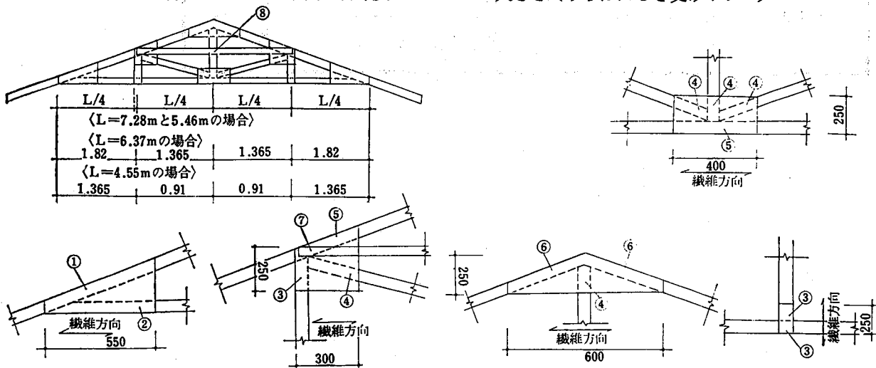
合板ガセット継手箇所番号及びガセットの大きさ(けらばたるき受けトラス)
