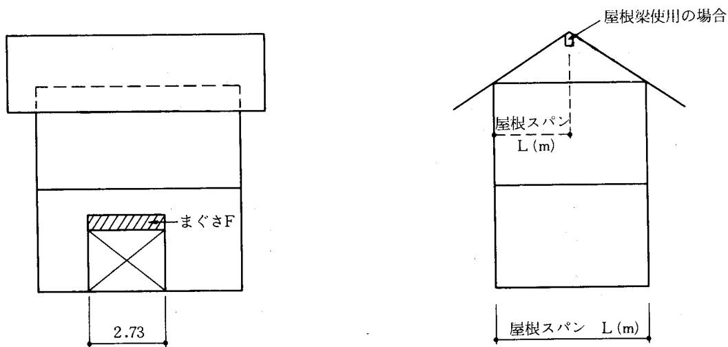
50表 まぐさスパン表⑩ (2階床根太がまぐさFと直交の場合)
