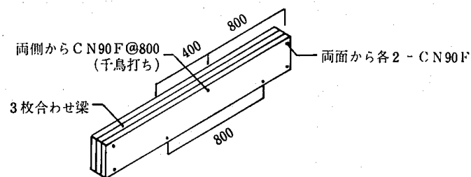
25図 合わせ梁のつくり方
