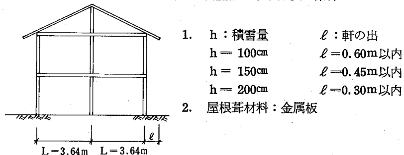
73表 たて枠間隔（その1）（ L=3.64\text{m} 勾配5/10以下）
