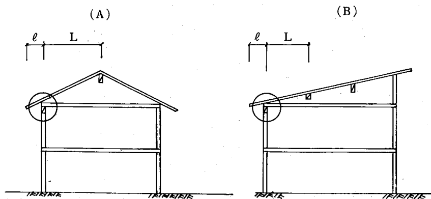
35図 まぐさが支持する屋根荷重の取り方
