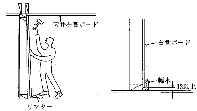
94図 壁せこうボードのはり方とおさまり
