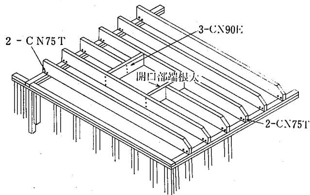
62図 天井根太における小さな開口部
