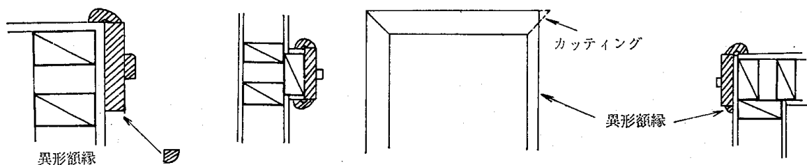
104図 異形額縁
