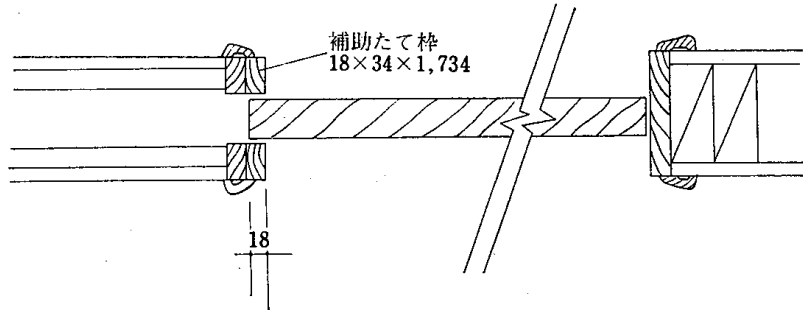
121図 補助たて枠の取り付け
