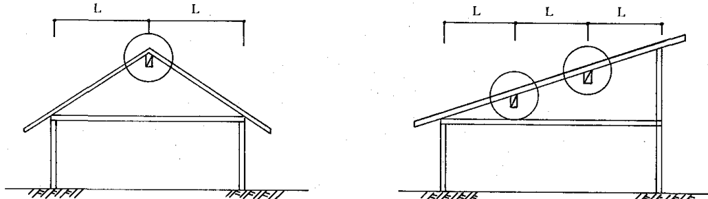
3図 屋根梁間隔の取り方
