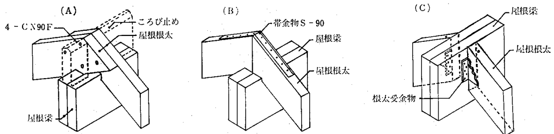
72図 屋根梁と屋根根太のおさまり
