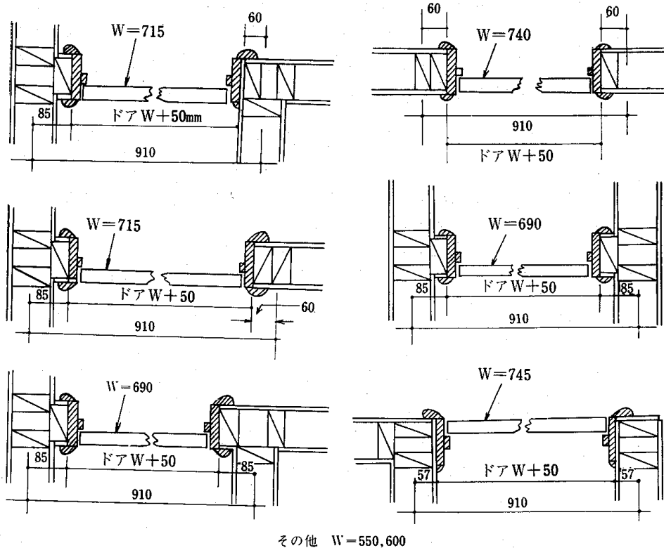
106図 各ドアの幅と開口部のおさめ方
