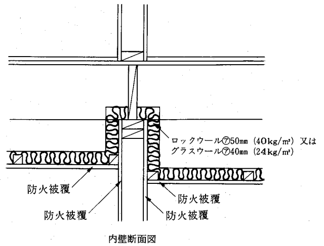
16.3図 防火被覆の取合部
