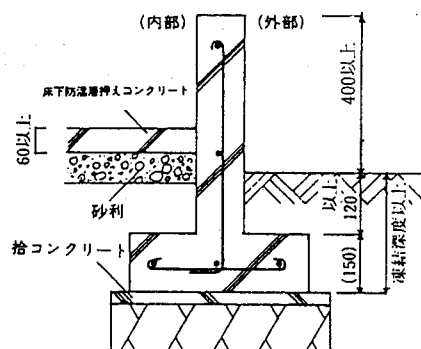
参考図Ⅱ.4 床下防湿層抑えコンクリート
