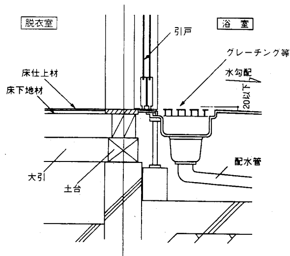
「浴室出入口の施工例（ユニットバスの場合）」
