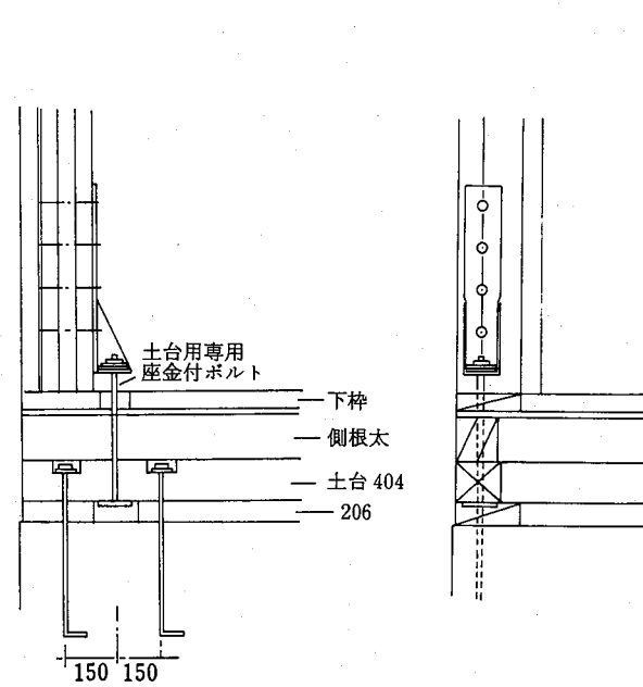
(A-2) 比較的引き抜き応力が小さい場合の施工例
