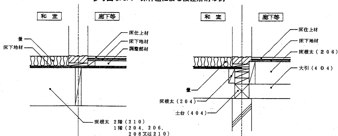
参考図 I. 3.1 床枠組による段差解消の例
