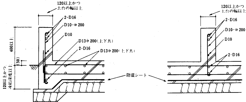
参考図 Ⅱ. 2 ベタ基礎詳細図 (mm)
