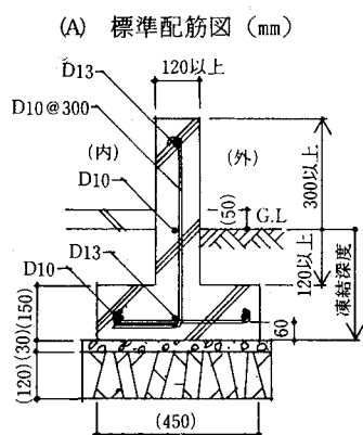
イ. 布基礎詳細図 単位 mm
