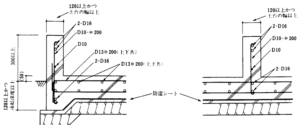
ロ. べた基礎詳細図 単位 mm
