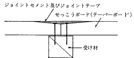
ニ. テーピング処理
