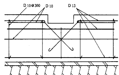
ハ. 床下換気孔廻りの補強
