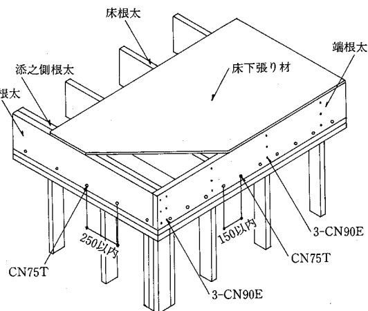
○端根太ころび止めを省略する場合
