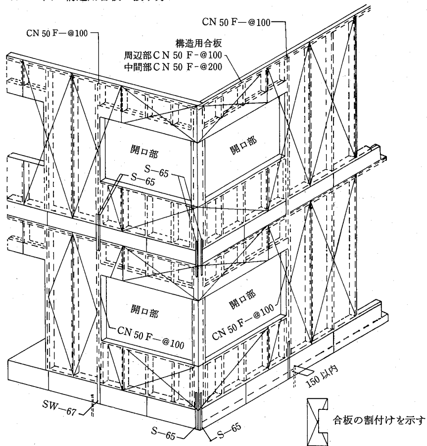
4.7-11図 構造用合板の張り方
