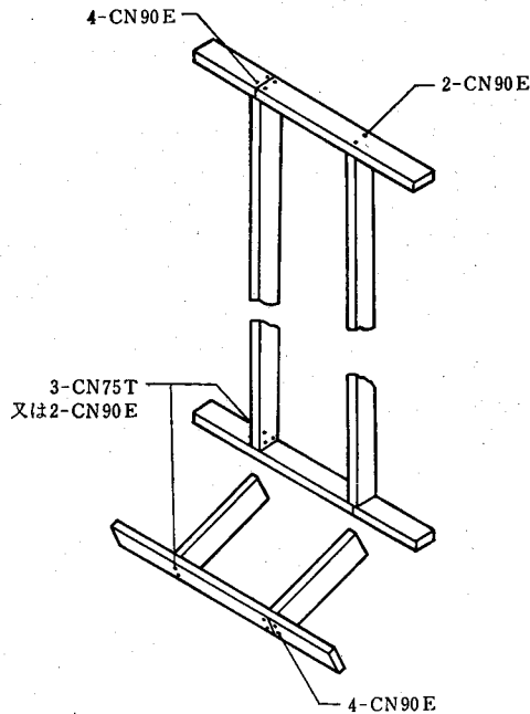
4.7-2図 頭つなぎ釘打ち
