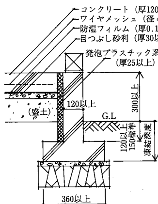
内断熱施工例
