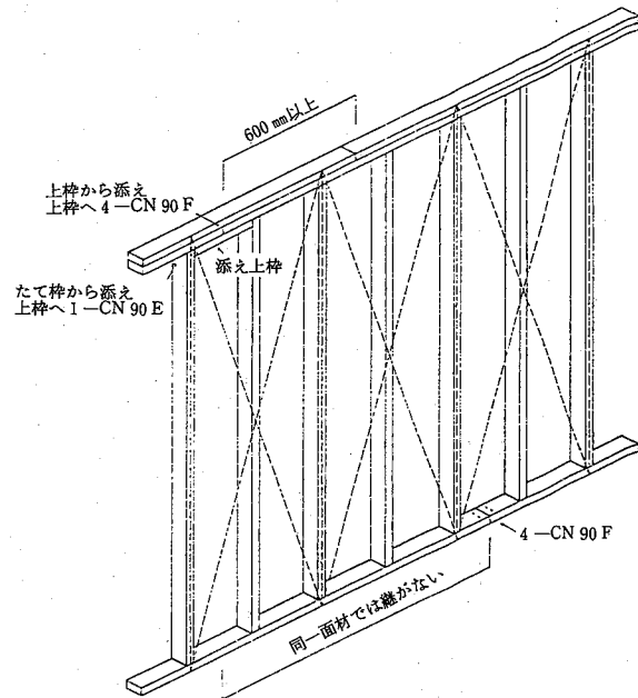
4.7-2図 頭つなぎ釘打ち
