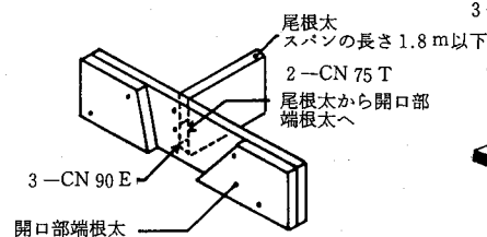
4.6-7図 尾根太の釘打ち
