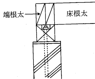
4.5-2図 座金ばり
