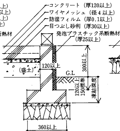
外断熱施工例
