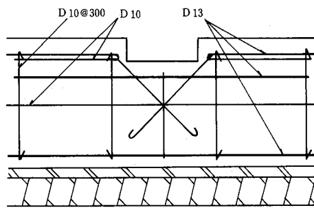
(B) 換気口廻りの補強
