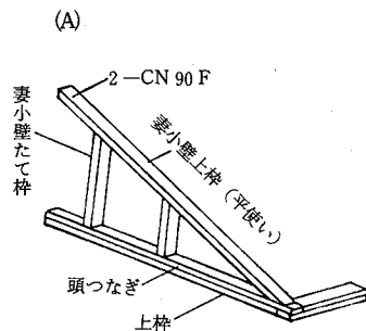
4.9-5 図 妻小壁
