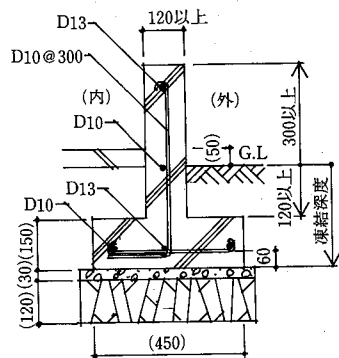
(A) 標準配筋図 (mm)
