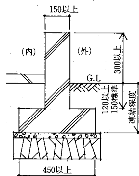
(B) 多雪区域 2階建
