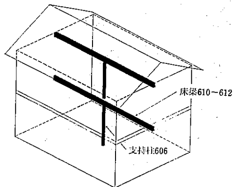
4.8-1図 支持柱
