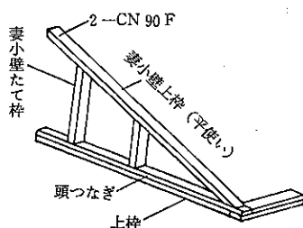
4.9-5 図 妻小壁
