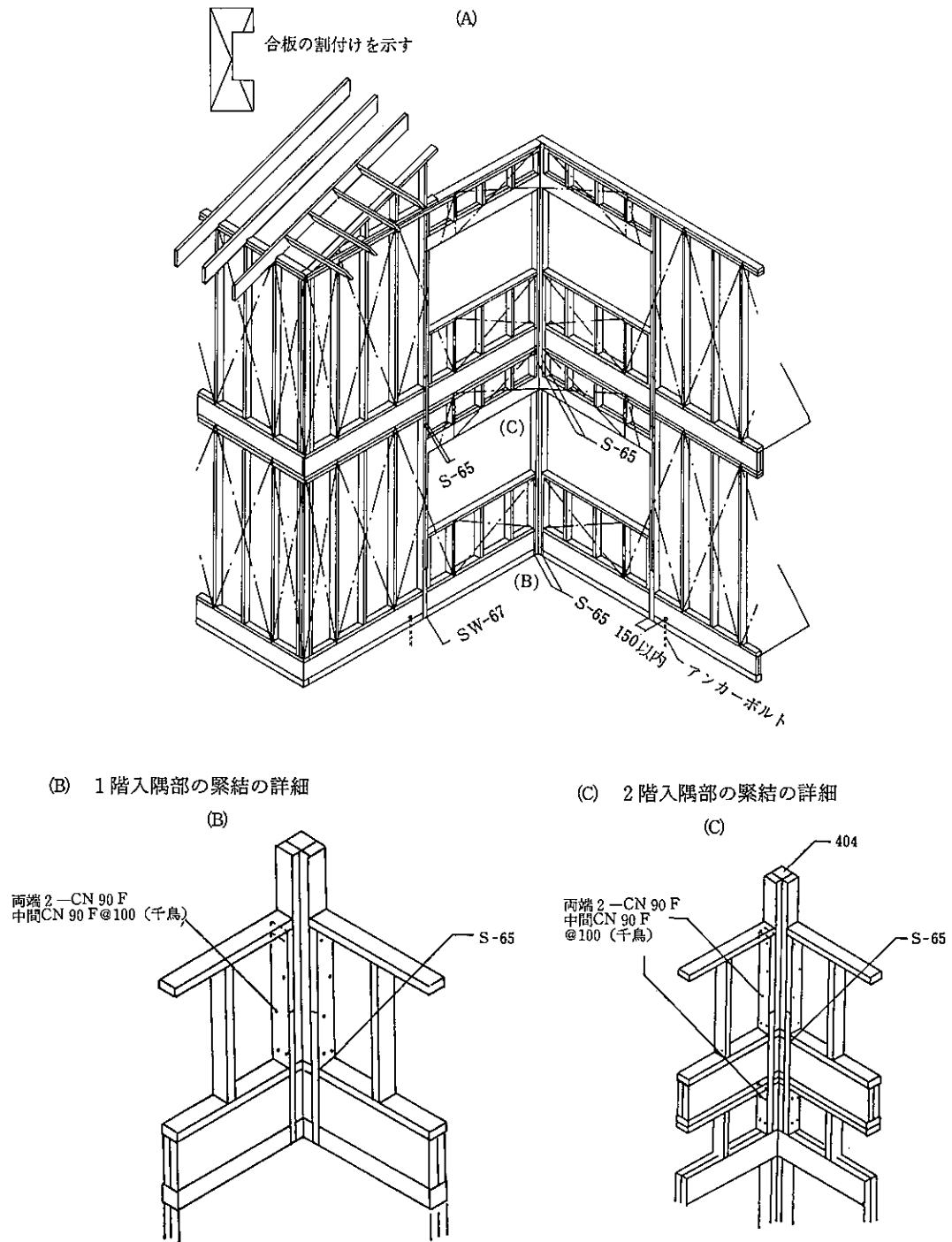
4.7-14図 入隅部の補強
