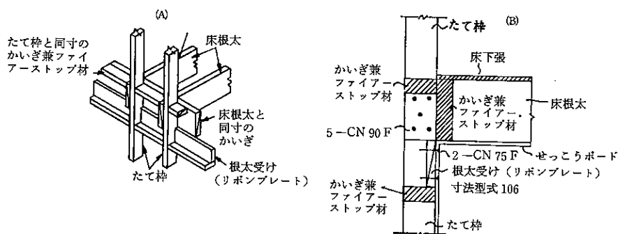
4.7-20 図 スキップフロアの構成例
