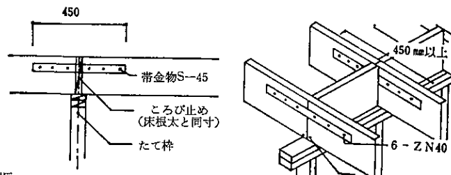
(C) 帯金物
