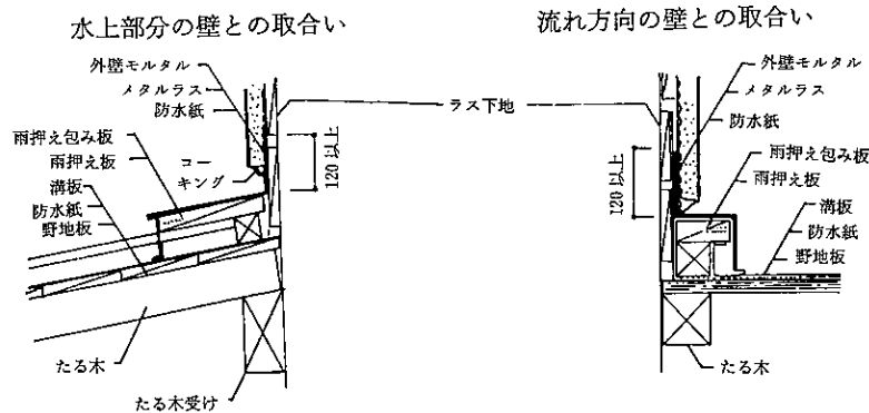
参考図 5.2.10
