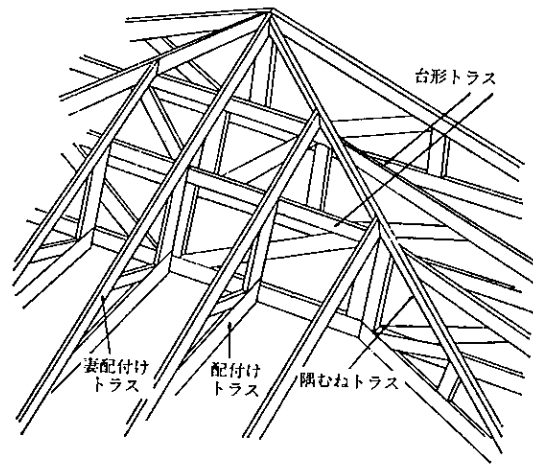
4.9-19 図 トラスによる寄棟のおさまり例
