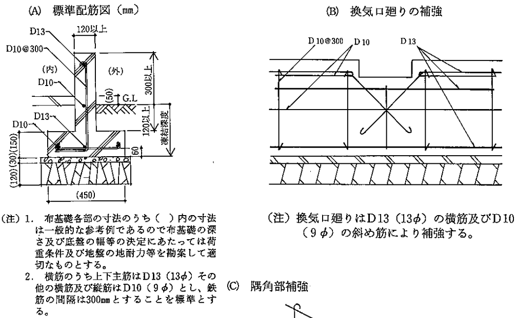
3.4-2図 布基礎詳細
