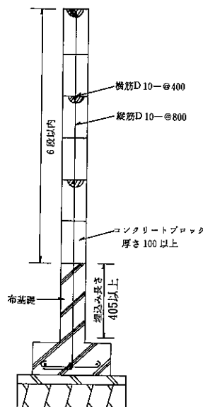
3.4-3図 腰壁詳細 (一般地例)
