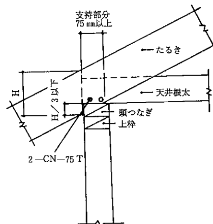
4.9-8 図 たるきのおさまり
