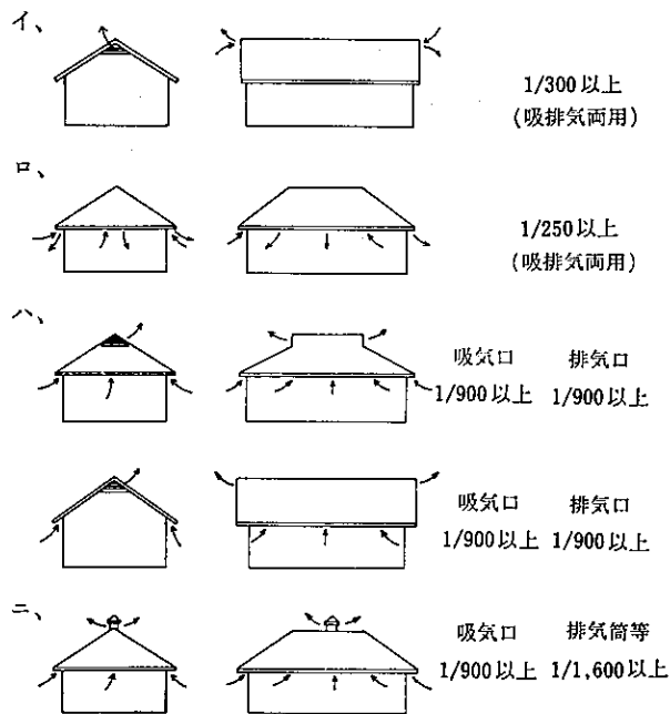
4.10-1 図 換気口の取り方例
