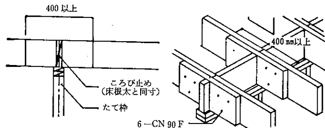
(B) 添え木
