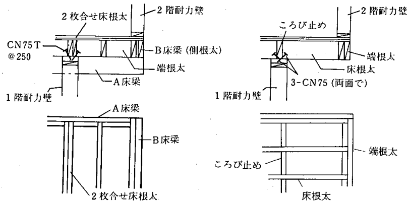
4.6-12図 隅角部の補強
