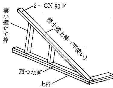
4.9-5 図 妻小壁
