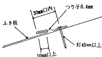
参考図 5.2.2 つり子止め
