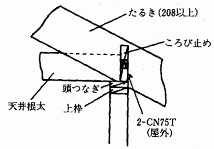
4.9-12 図 たるきのころび止め
