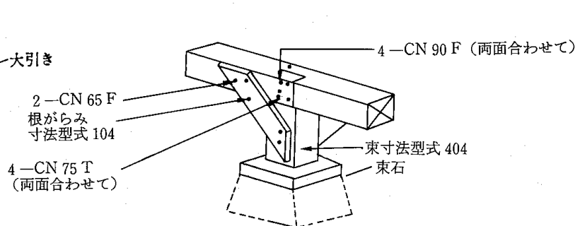
4.5-4図 大引きの継手
