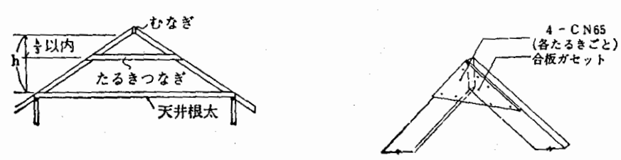
4.9-12 図 たるきのころび止め
