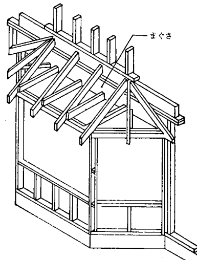
4.7-10図 出窓などのまぐさの入れ方例
