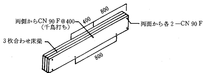
4.6-15図 合わせ床梁のつくり方
