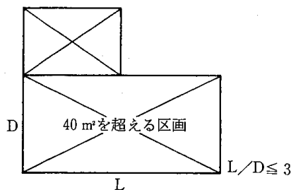
4.6-22図 40㎡を超える区画の形状比
