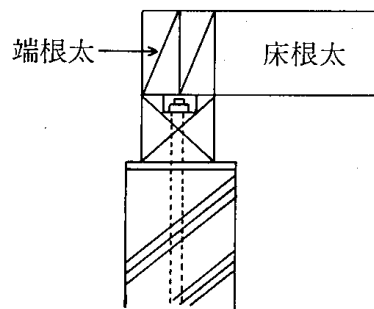
4.5-2図 座金ぼり
