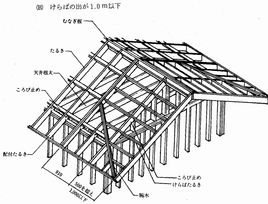
4.9-11 図 たるきつなぎ
