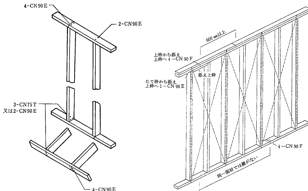
(B)図 たて枠相互間の中間位置で継ぐ場合
