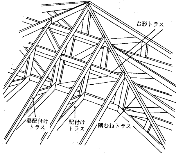
4.9-19 図 トラスによる寄棟のおさまり例
