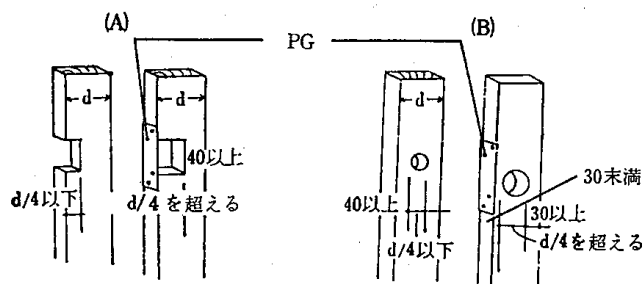
4.7-15図 たて枠の欠き込みと穴あけ
