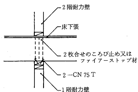
4.6-24図 「40㎡を超える区画」の床下張り
