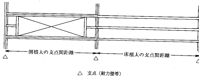
(A) 開口部が支点間の中にある場合
