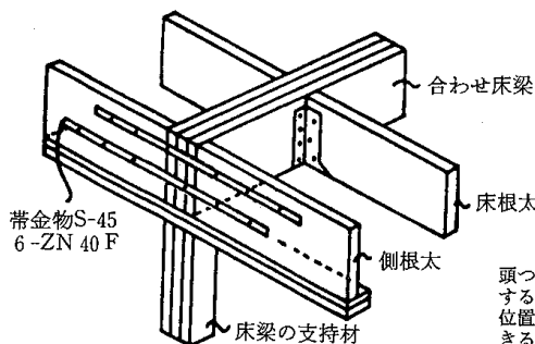
(A) 床梁の支持(壁の上)
