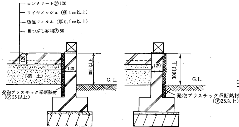
3.4-4図 土間コンクリート床
