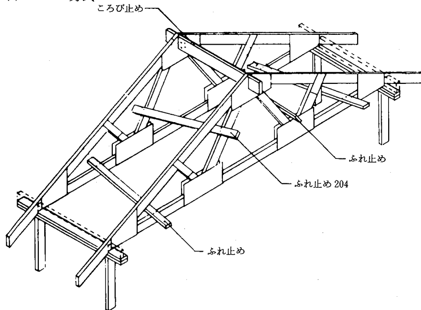
(C) トラス方式
