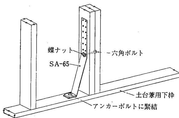
4.7-13図 ストラップアンカーの取付け方
