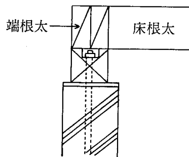
4.5-2図 座金ぼり
