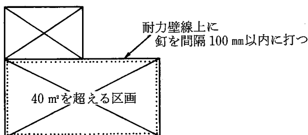
4.6-24図 「 40\text{m}^2 を超える区画」の床下張り
