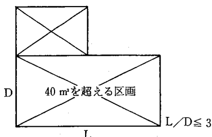
4.6-22図 40\text{m}^2 を超える区画の形状比
