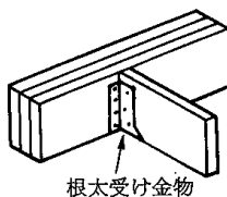
4.6-17図 根太がけの方法と釘打ち
