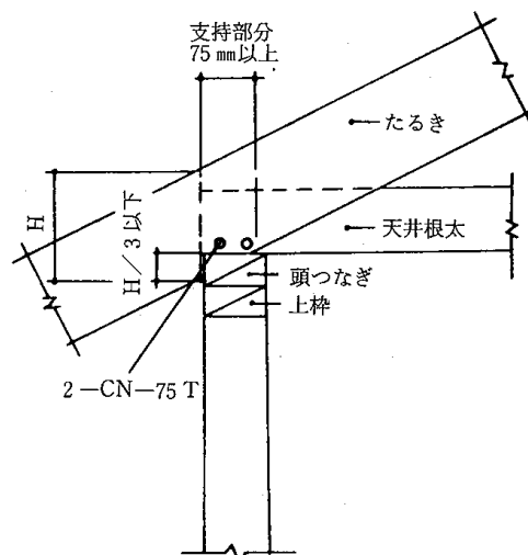
4.9-8 図 たるきのおさまり
