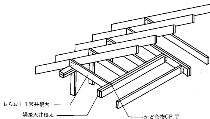
4.9-10 図 軒のはりだし方
