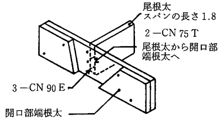
4.6-7図 尾根太の釘打ち
