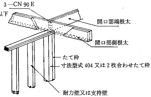
4.6-8図 開口部端根太端部の支持
