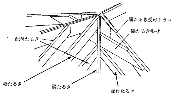
4.9-17 図 寄棟部分の構成
