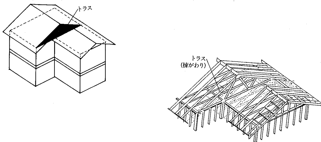
4.9-28 図 棟違い屋根
