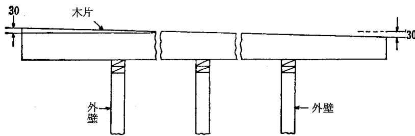
4.9-24 図 陸屋根の勾配のとり方
