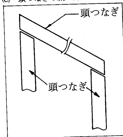
(C) 頭つなぎの納め方
