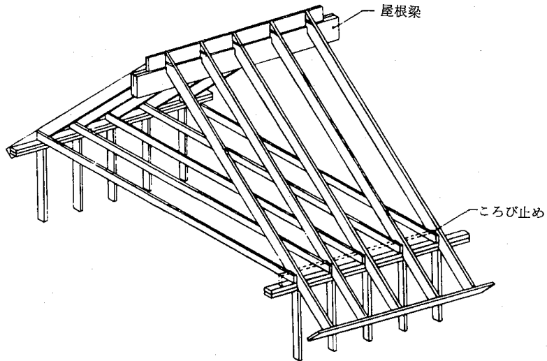
(B) 屋根梁方式
