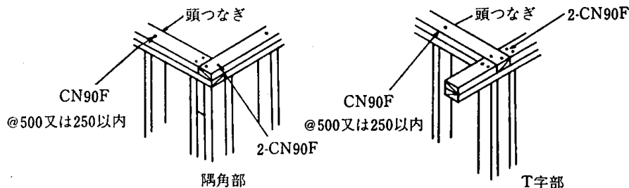
4.7-2図 頭つなぎ釘打ち
