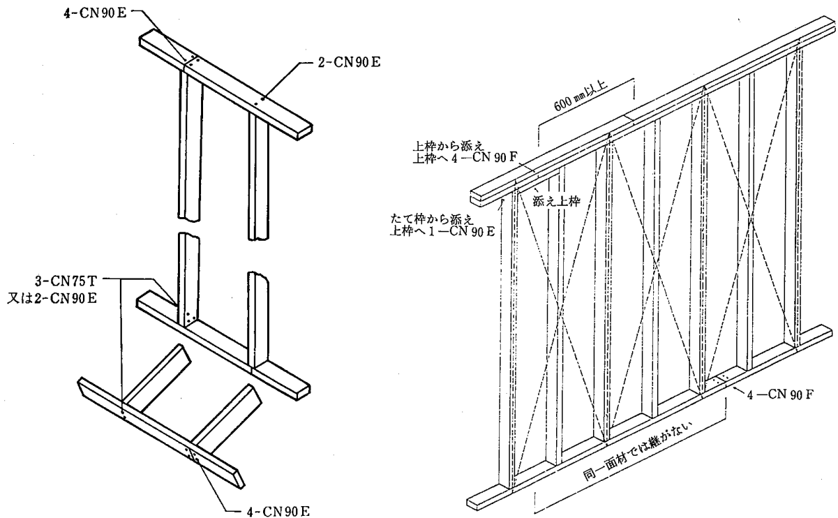
4.7-2図 頭つなぎ釘打ち
