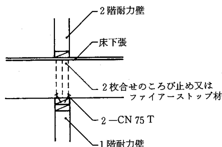
4.6-24図 「 40\text{m}^2 を超える区画」の床下張り
