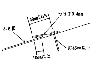
参考図 5.2.2 つり子止め
