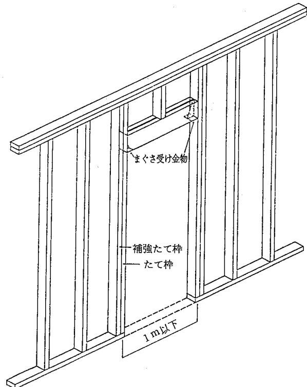
(B)図 外壁で使用する場合の補強
