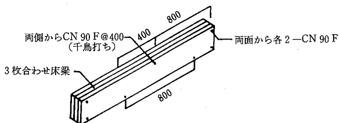
4.6-15図 合わせ床梁のつくり方
