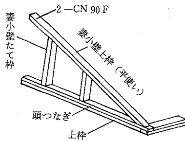
4.9-5 図 妻小壁
