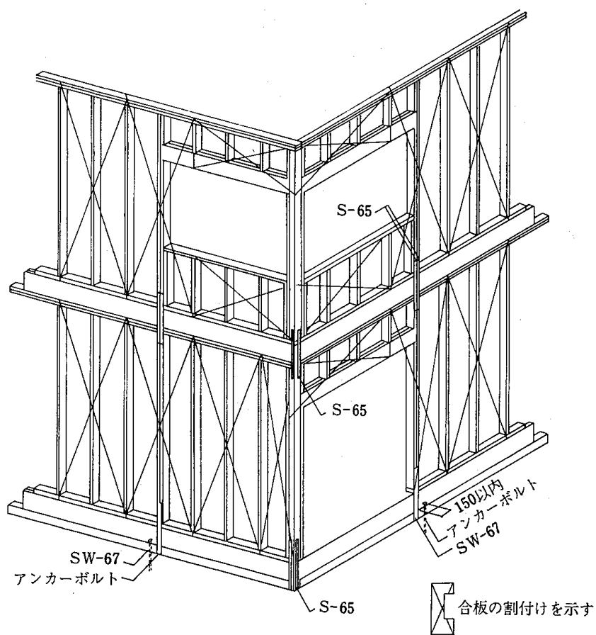
4.7-13図 ストラップアンカーの取付け方
