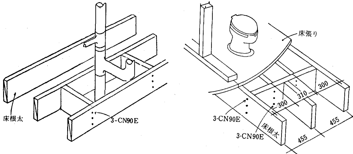
4.6-20図 太い管のおさめ方例
