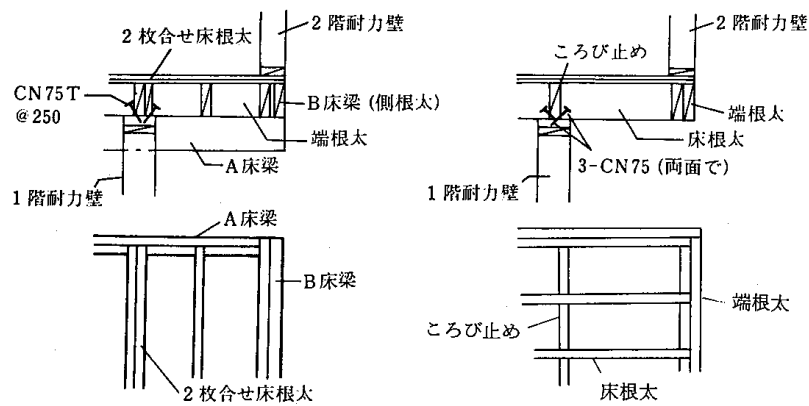
4.6-12図 隅角部の補強
