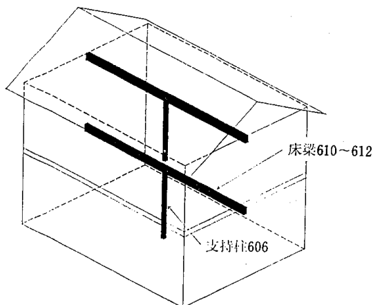
4.8-1図 支持柱
