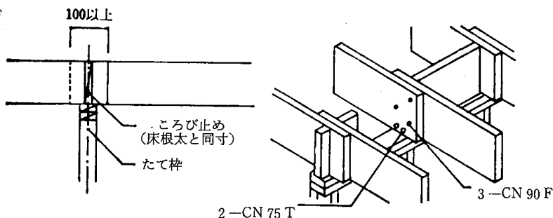
4.6-2図 床根太の継手
