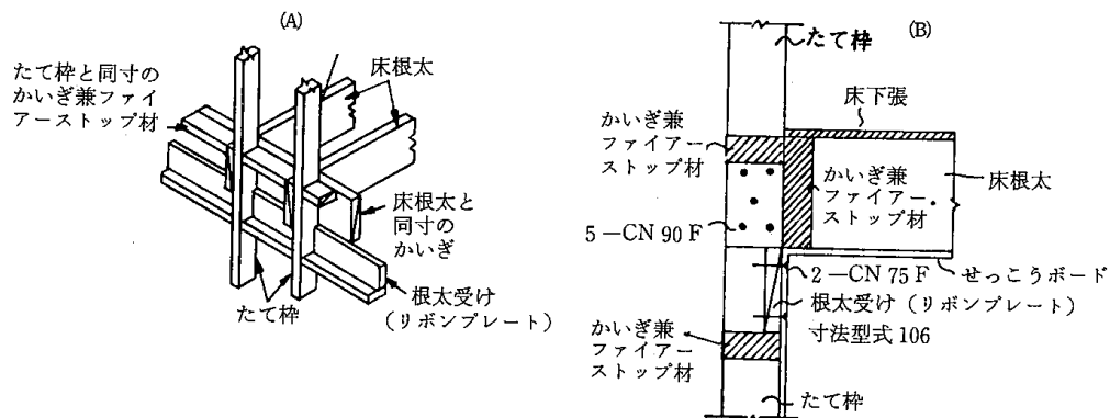
4.7-20 図 スキップフロアの構成例
