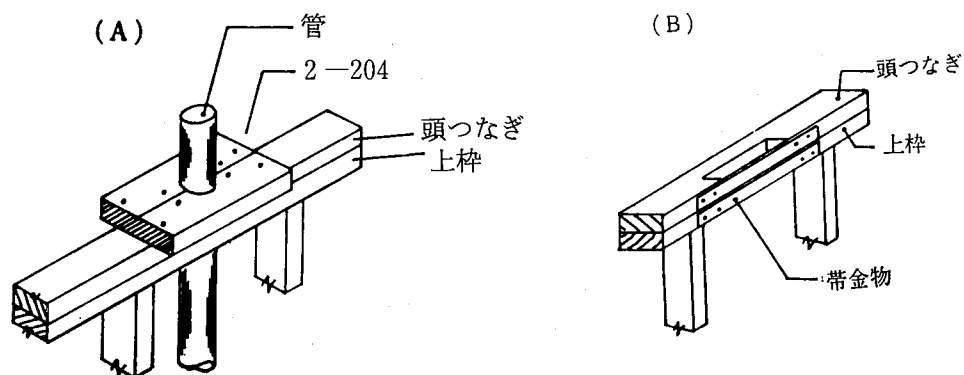
4.6-16図 上枠、頭つなぎの補強
