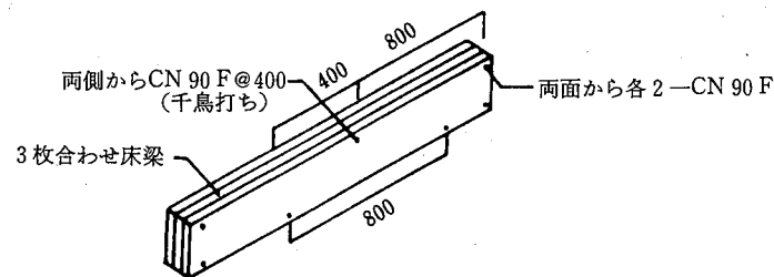
4.5-15図 合わせ床梁のつくり方
