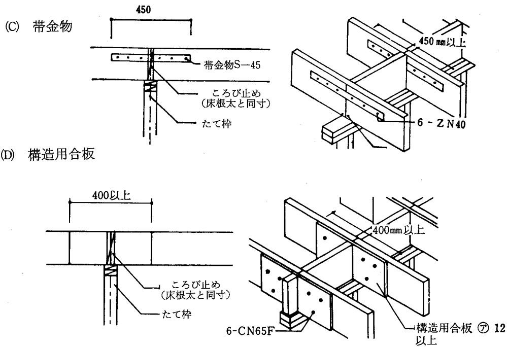
4.5-3図 端根太と側根太又は床根太との仕口 4.5-4図 床の補強
