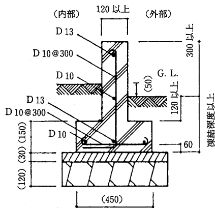
(A) 標準配筋図 (mm)
