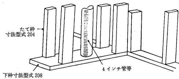
4.6-17 図 太い管を壁中に配する方法例
