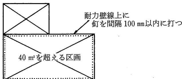
4.5-24図 「40㎡を超える区画」の床下張り
