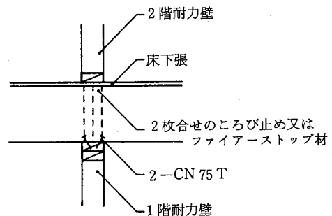
4.5-24図 「40㎡を超える区画」の床下張り
