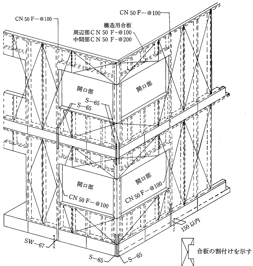
4.6-11図 構造用合板の張り方
