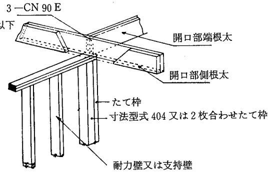
4.5-8図 開口部端根太端部の支持
