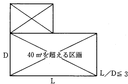
4.5-22図 40㎡を超える区画の形状比
