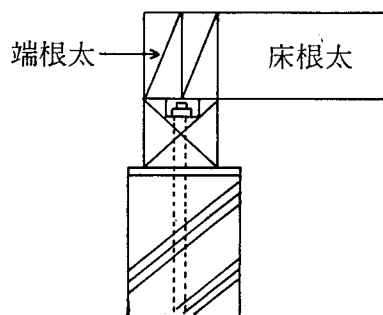
4.4-2図 座金ぼり
