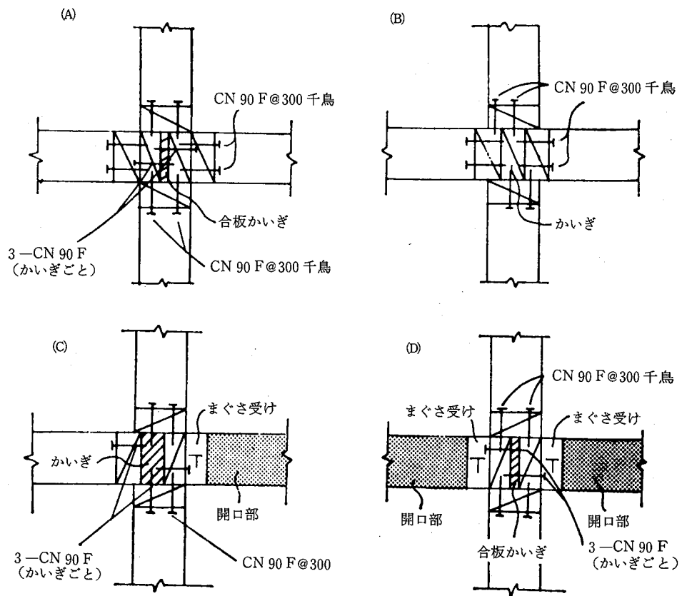
4.6-5図 耐力壁が十字型に接合する場合の隅柱の構成
