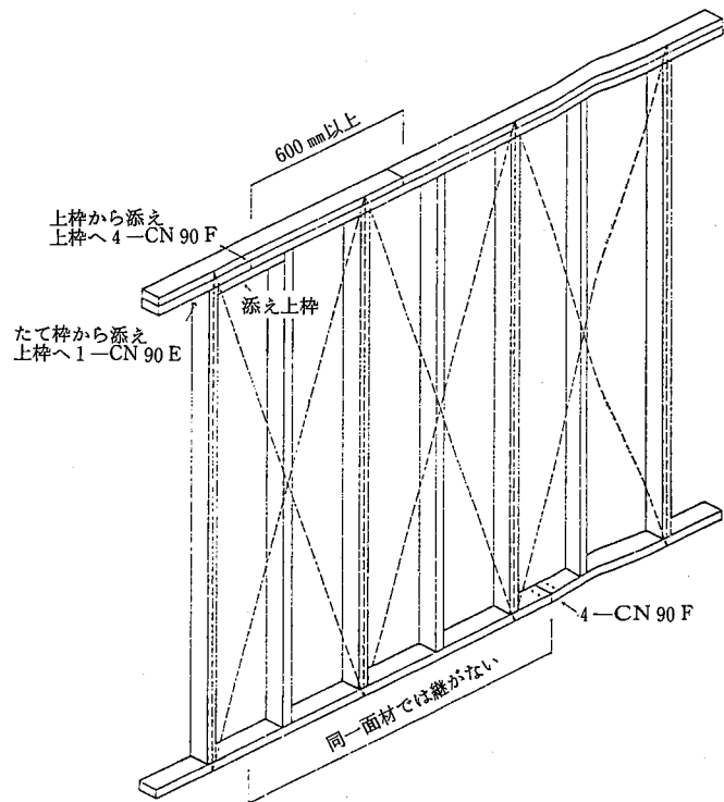
(B)図 たて枠相互間の中間位置で継ぐ場合
