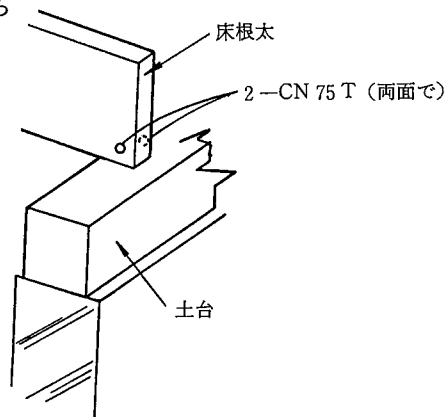
4.5-2図 床根太の継手
