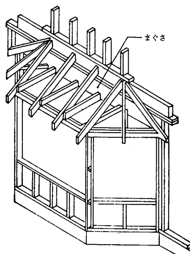
4.6-10図 出窓などのまぐさの入れ方例
