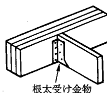
4.5-17図 根太がけの方法と釘打ち
