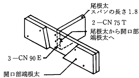
4.5-7図 尾根太の釘打ち
