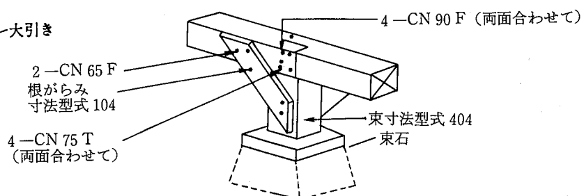
4.4-4図 大引きの継手
