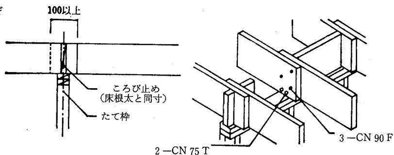
4.5-2図 床根太の継手
