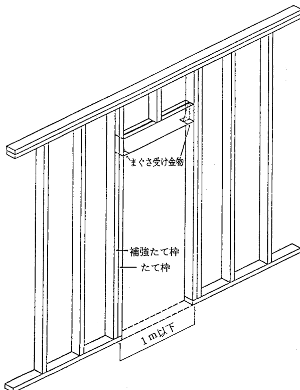
(B)図 外壁で使用する場合の補強
