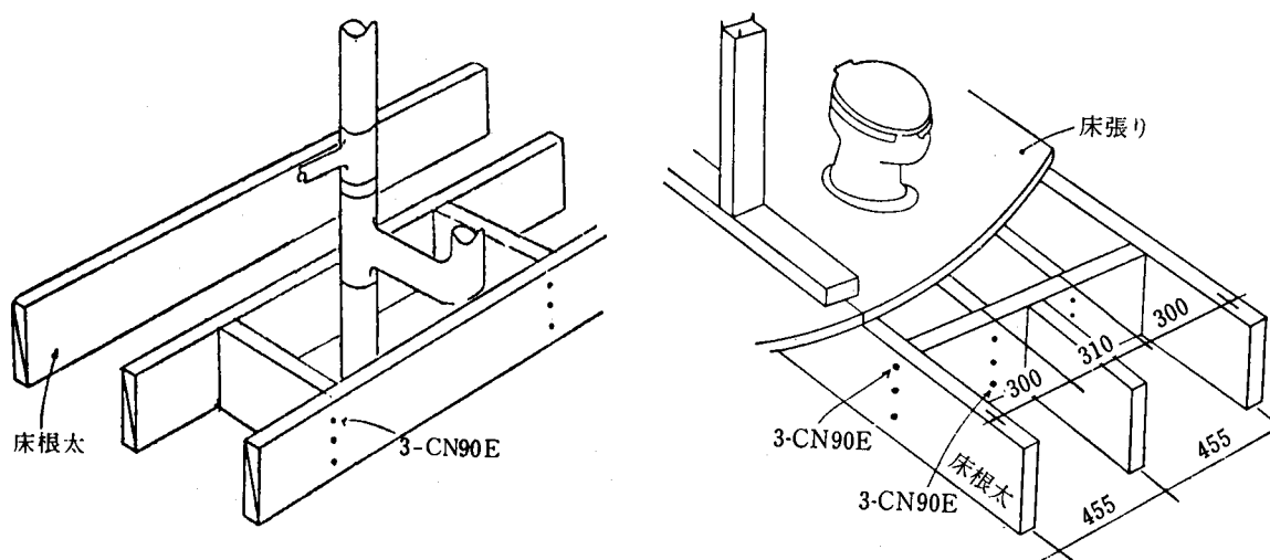
4.5-20図 太い管のおさめ方例
