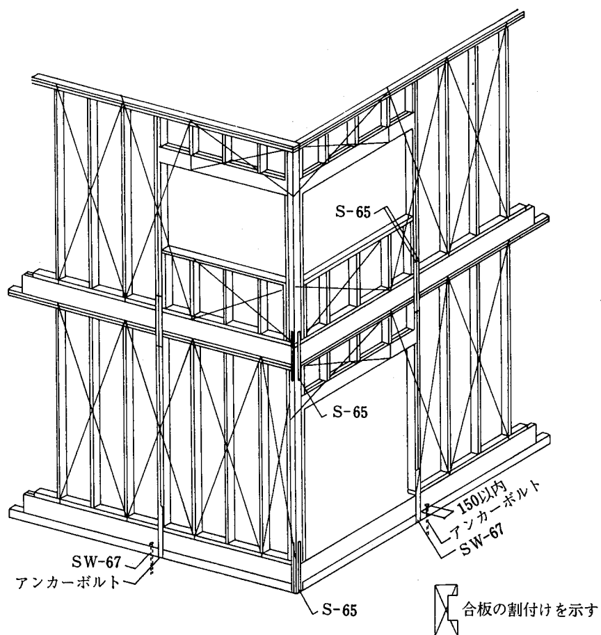
4.6-13図 ストラップアンカーの取付け方
