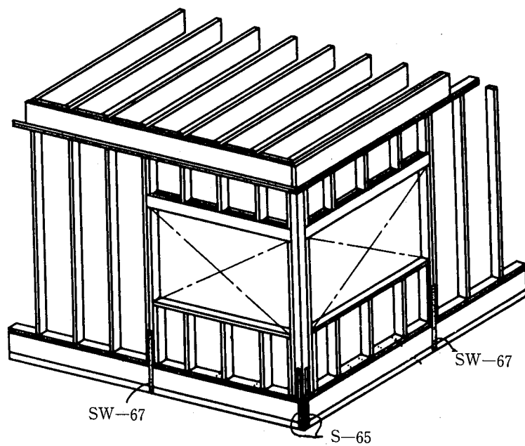
4.6-12図 両面開口部詳細
