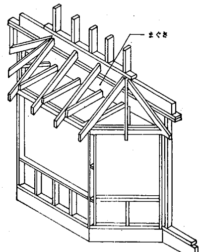
4.6—10図 出窓などのまぐさの入れ方例
