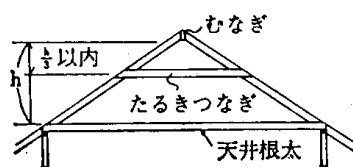
4.8-11図 たるきつなぎ
