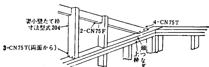
4.8—23図 妻小壁の詳細
