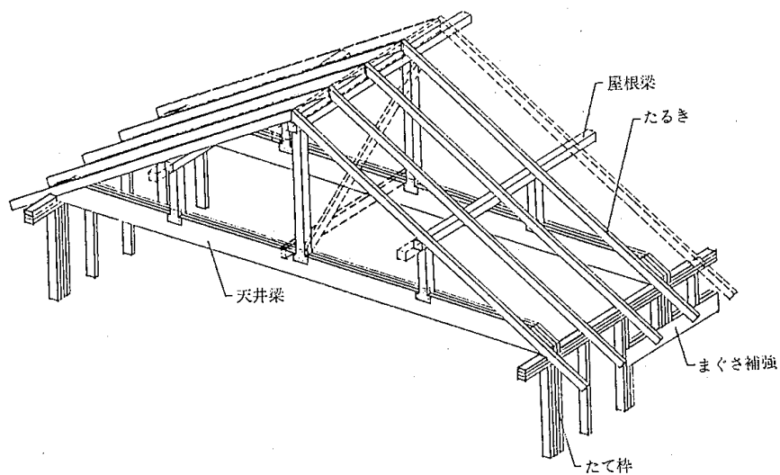
(D) 束建て方式
