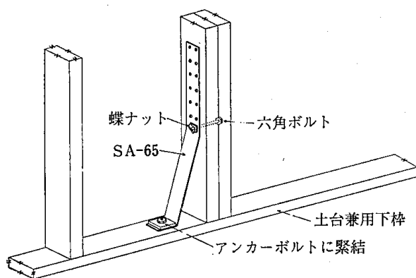
4.6-13図 ストラップアンカーの取付け方
