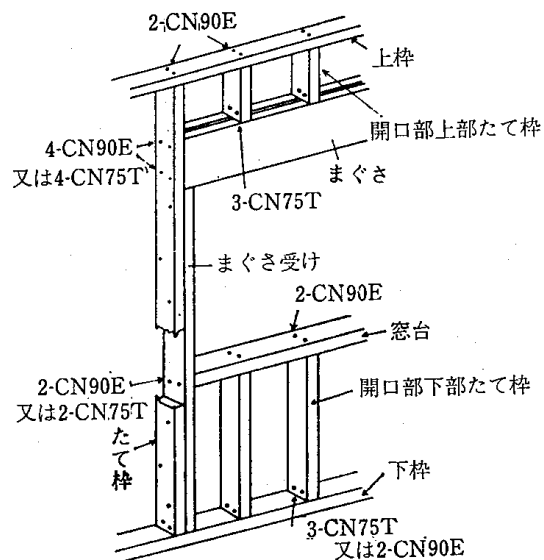
4.6—9図 開口部のまわりの釘打ち
