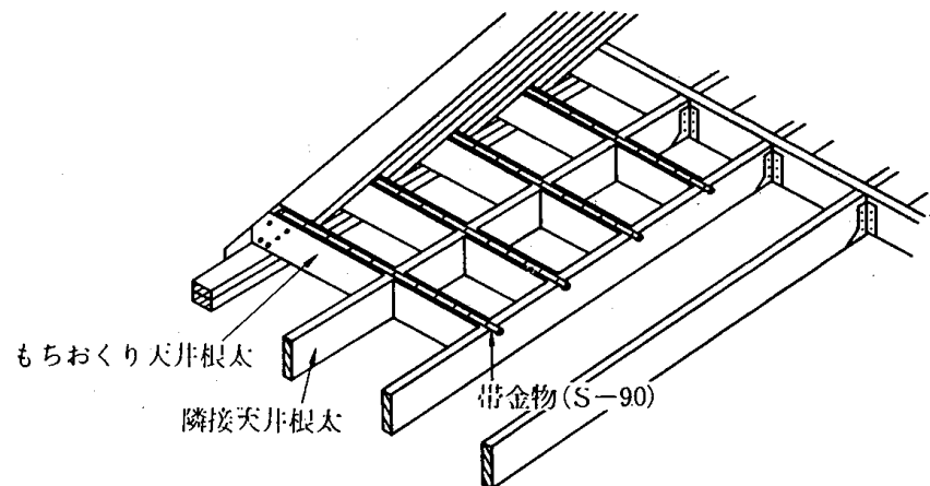
4.8—10図 軒のはりだし方
