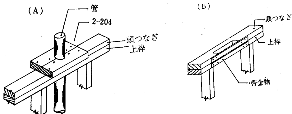
4.6—16図 上枠、頭つなぎの補強
