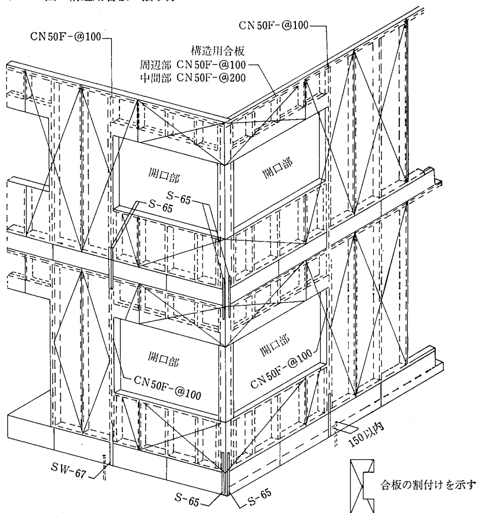
4.6—11図 構造用合板の張り方
