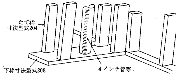
4.6—17図 太い管を壁中に配する方法例
