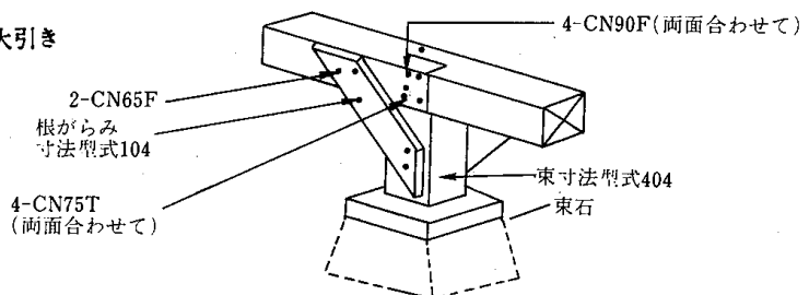
4.4—4 図 大引きの継手
