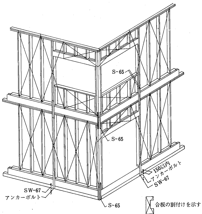
4.6-13図 ストラップアンカーの取付け方
