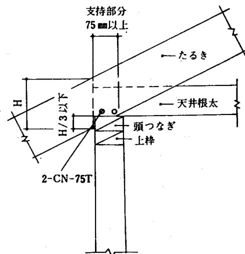
4.8—8図 たるきのおさまり
