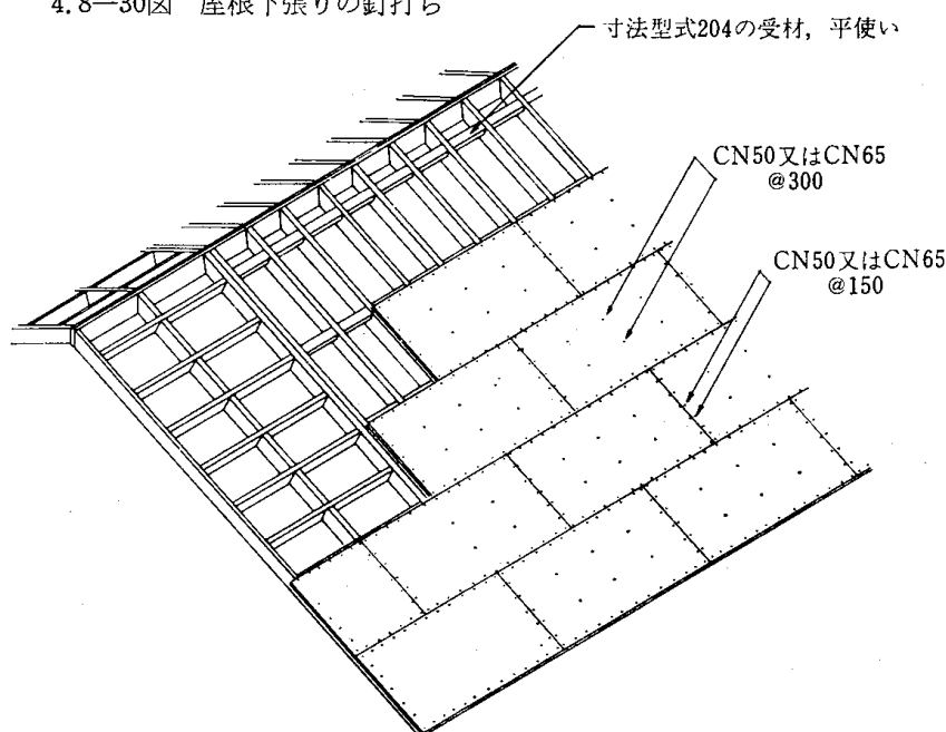
4.8—30 図 屋根下張りの釘打ち
