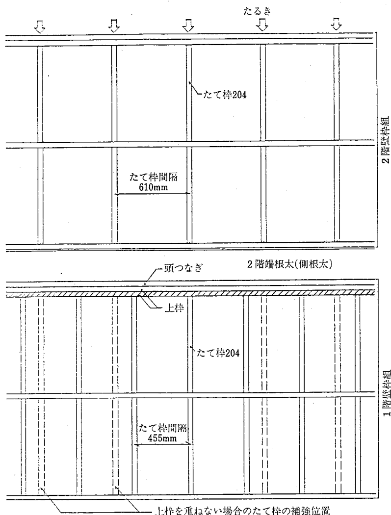
4.6—23図 たるき及び床根太とたて枠の位置がずれる場合の補強
