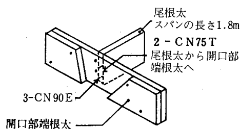
4.5-7 図 尾根太の釘打ち
