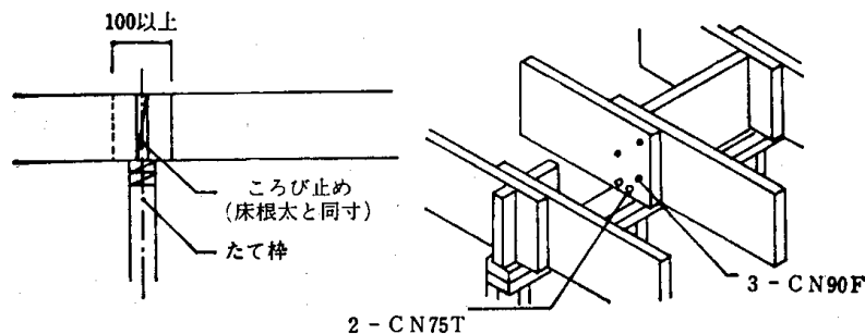
4.5—2図 床根太の継手
