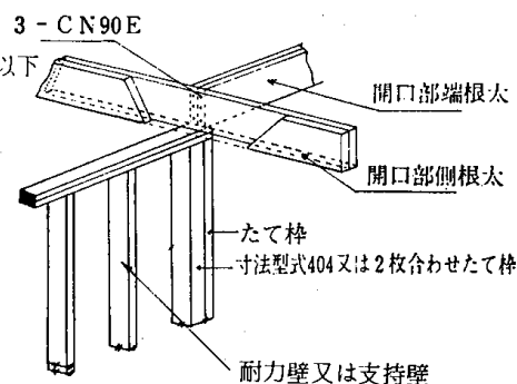
4.5-8 図 開口部端根太端部の支持
