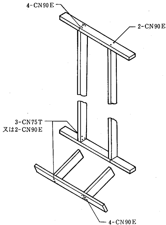
(A)図 たて枠の中央で継ぐ場合
