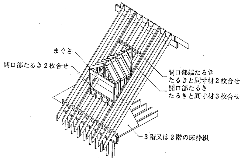
4.8—29図 屋根開口部のとり方
