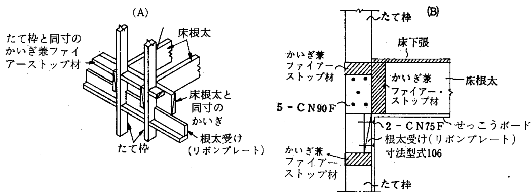
4.6-20図 スキップフロアの構成例
