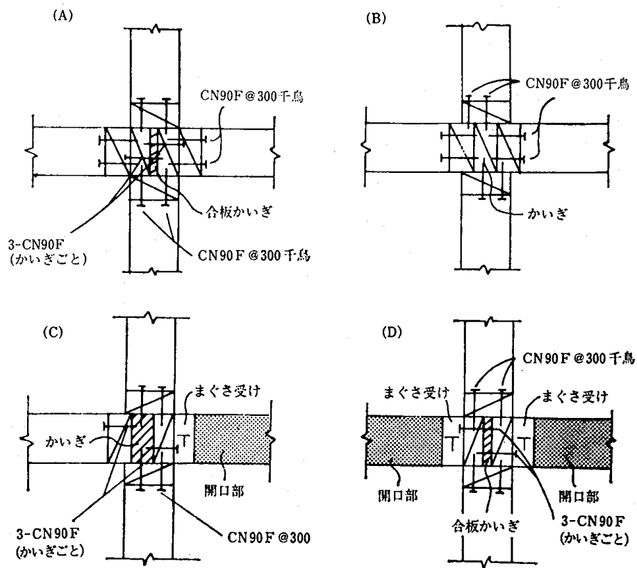
4.6—5 図 耐力壁が十字壁に接合する場合の隅柱の構成
