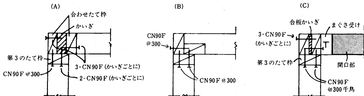
4.6—3図 耐力壁がL字型に接合する場合の隅柱の構成
