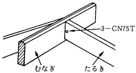
4.8—7図 むなぎとたるきの仕口
