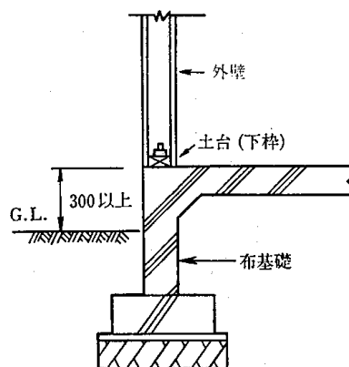
3.4—5 図 床と一体の布基礎
