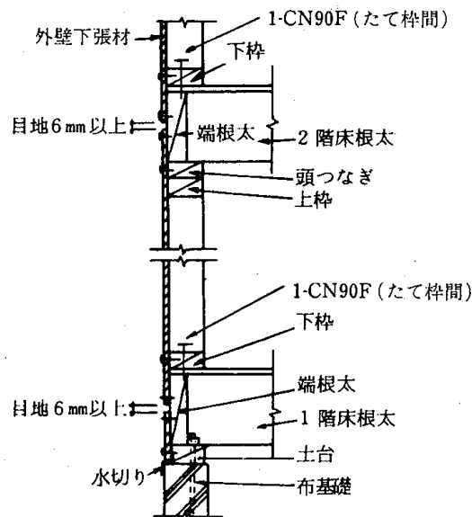
4.6-22図 帯金物（S-65）を省略する場合の壁下張りの張り方
