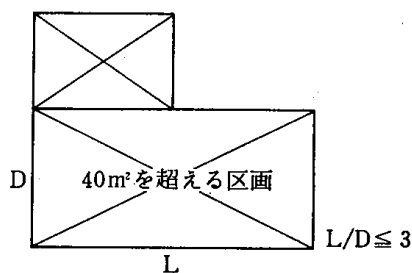
4.5—22図 40\text{m}^2 を超える区画の形状比
