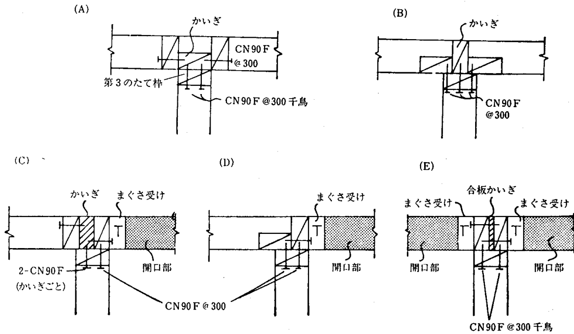
4.6—4 図 耐力壁がT字型に接合する場合の隅柱構成
