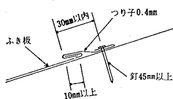
参考図 5.2.2 つり子止め
