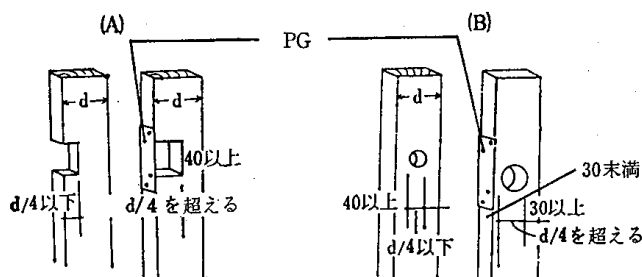
4.6—15図 たて枠の欠き込みと穴あけ
