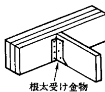
4.5-17図 根太がけの方法と釘打ち
