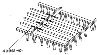
4.8—3図 梁への接合例
