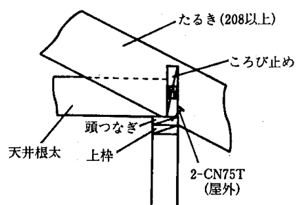
4.8-12図 たるきのころび止め
