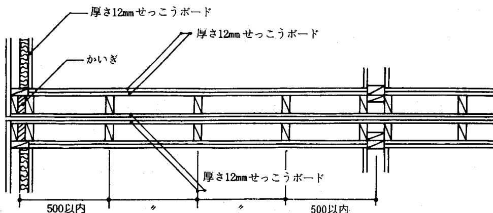
4.6-21図 連続建の住戸間界壁
