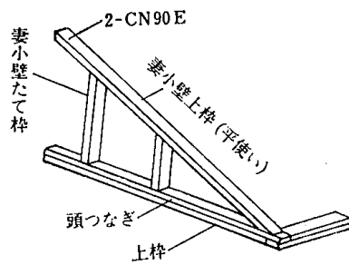
4.8—5図 妻小壁
