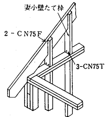
4.8—4図 妻小壁たて枠
