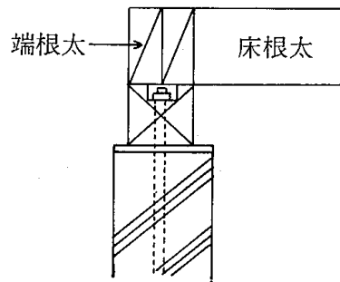
4.4—2 図 座金ぼり
