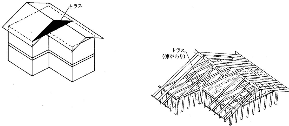
4.8—28図 棟違い屋根
