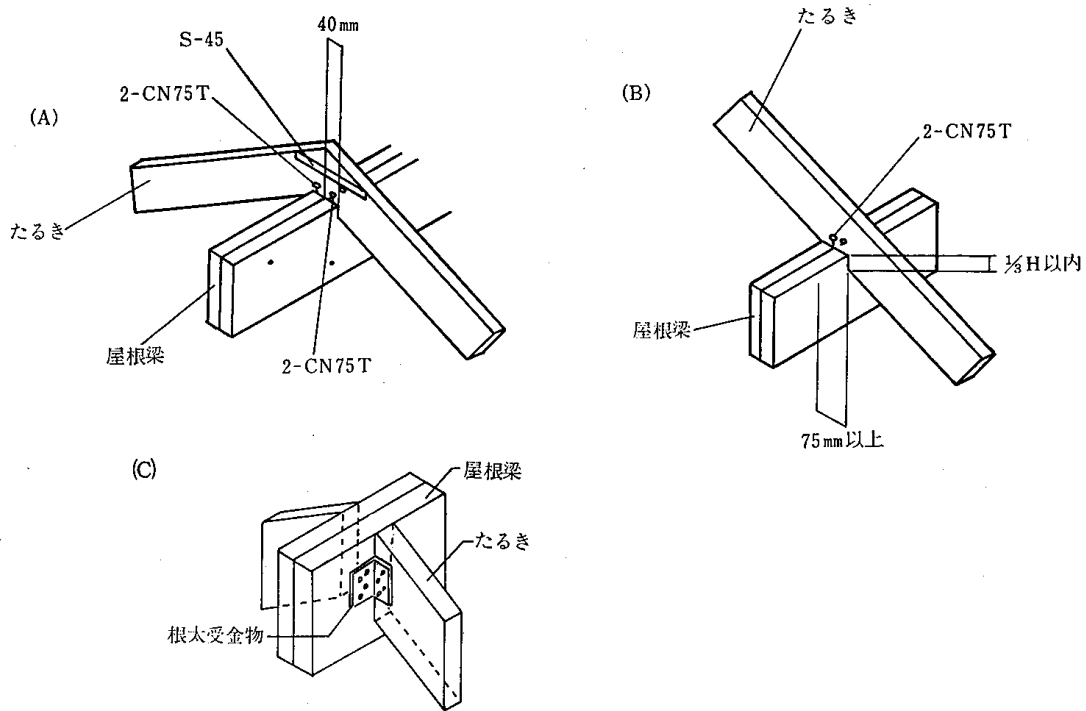
4.8—15図 屋根梁とたるき接合
