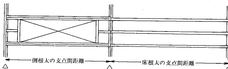
4.5-9 図 側根太の支点間距離のとり方
