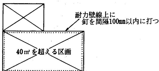
4.5—24図 「 40\text{m}^2 を超える区画」の床下張り
