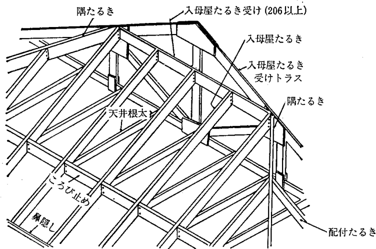
4.8—21図 入母屋の構成図
