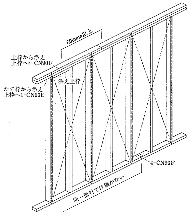
(B)図 たて枠相互間の中間位置で継ぐ場合
