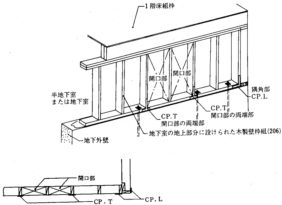
(A) 隅角部及び開口部両端部の補強
