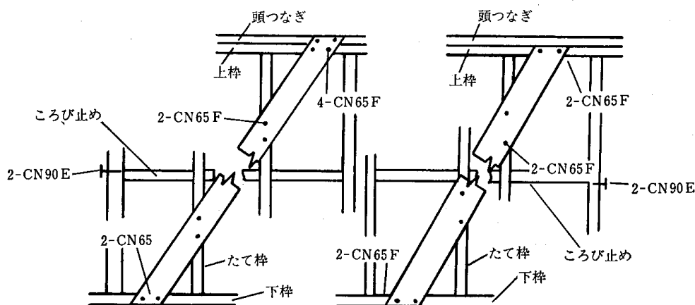
4.6—19図 筋かいの釘打ち
