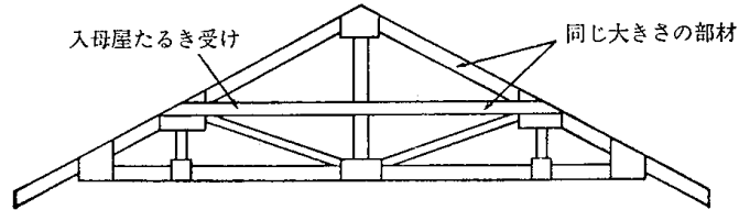
4.8—20図 入母屋たるき受けトラス
