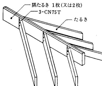
(B)たるき
