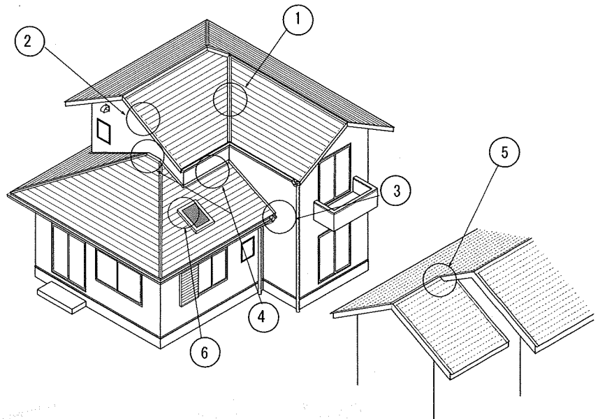
参考図5.2.2-4 雨漏りの発生のしやすい箇所
