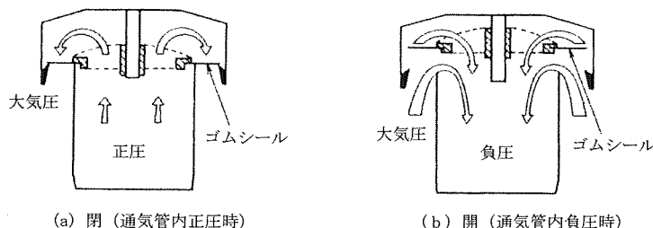
(a) 閉（通気管内正圧時）
