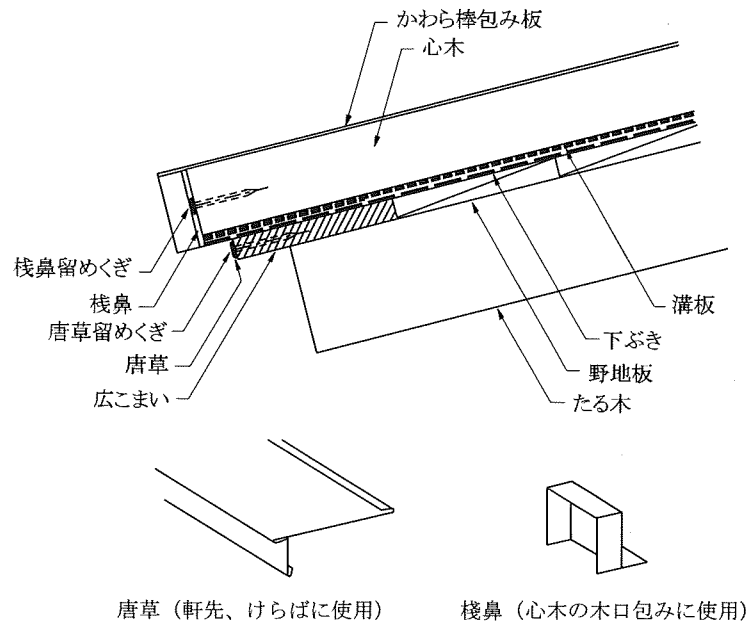
参考図5.3.9 軒部の納まり
