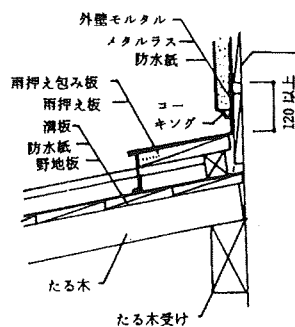
参考図5.3.8-1 水上部分の壁との取合い
