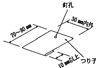
参考図5.3.2-2 つり子止め
