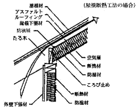
参考図4.13.1-3 外壁と屋根との取り合い部
