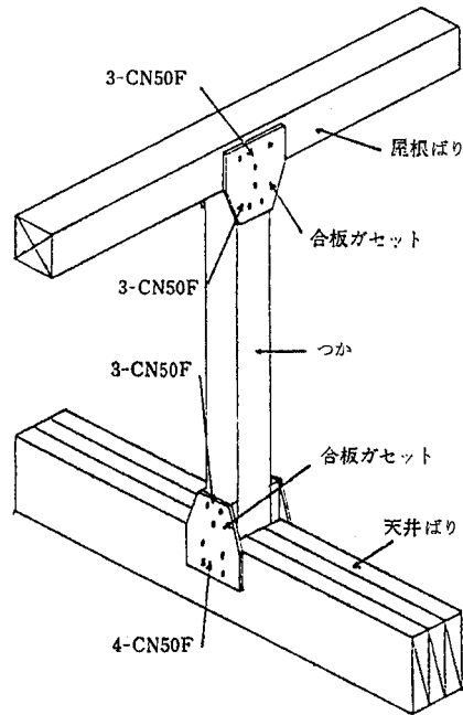
参考図4.12.11.3 屋根ばり、天井ばりとつかとの納まり
