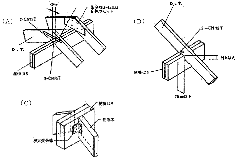
参考図4.12.3.2-3 屋根ばりとなる木接合
