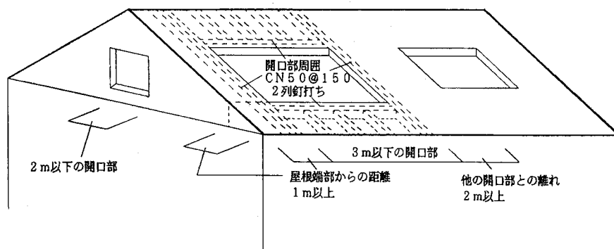
参考図4. 12. 14-1 屋根開口部の取り方
