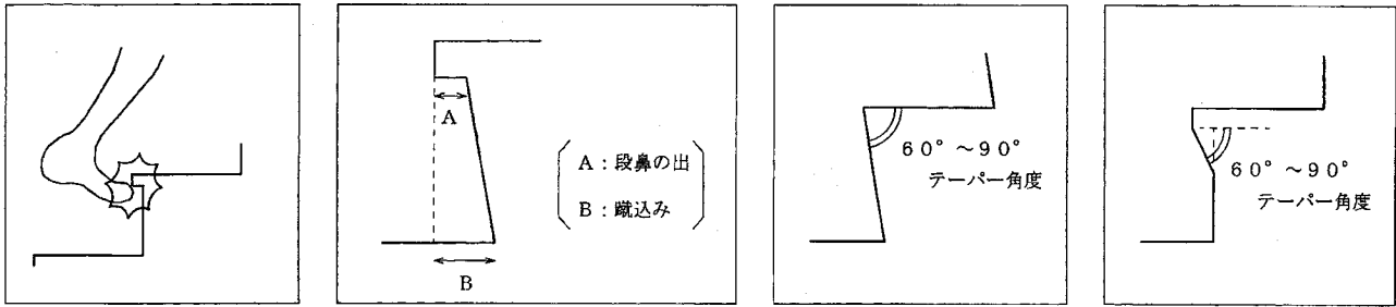
参考図4.4.2-1 蹴込み部分の留意点
