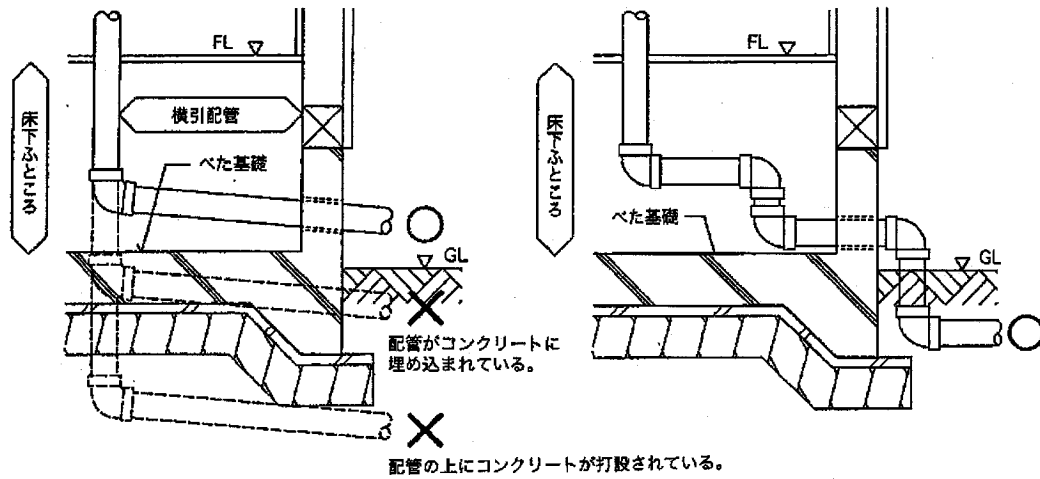
参考図5.9-1べた基礎の場合の配管方法
