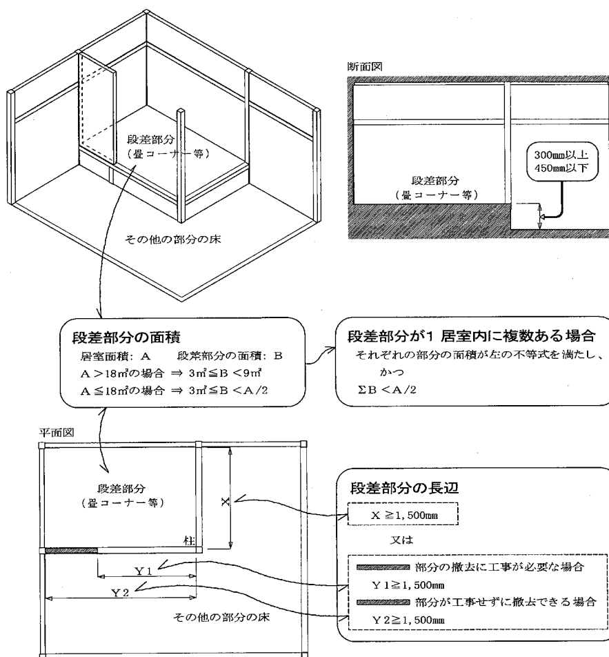
参考図4.3.1-3 300mm以上450mm以下の段差を設けることができる場合
