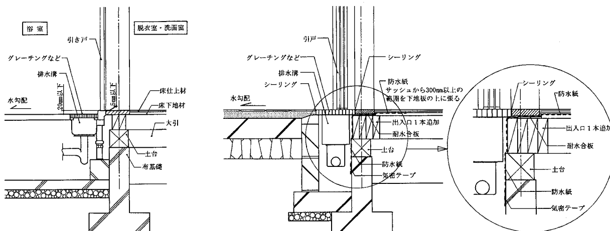
参考図4.3.1-3 浴室出入口段差を20mm以下とする施工例
