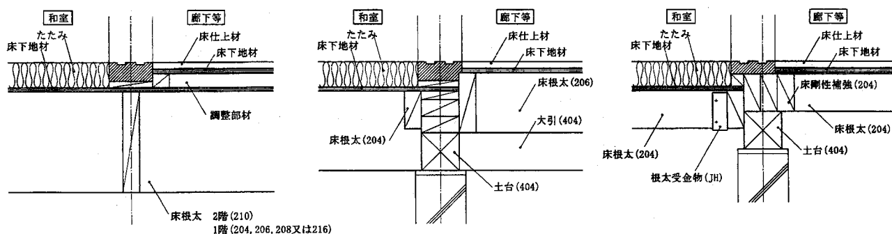
参考図4.3.2 床枠組による段差解消の例
