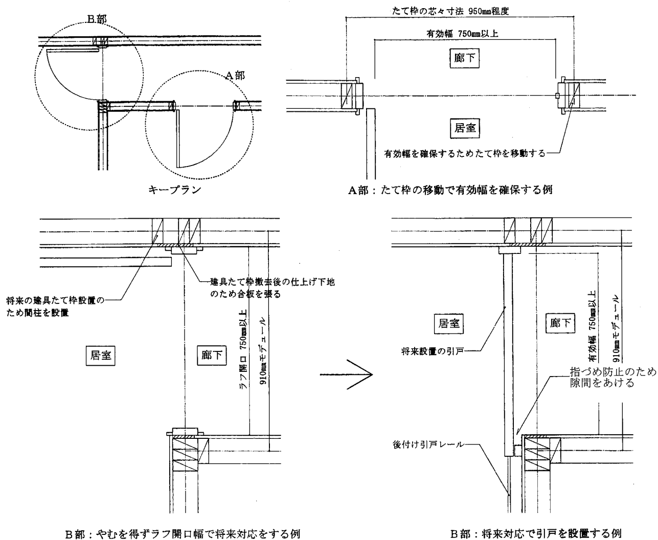
参考図4.6-3 構造上重要なたて枠以外のたて枠を調整して開口幅を確保する場合の例
