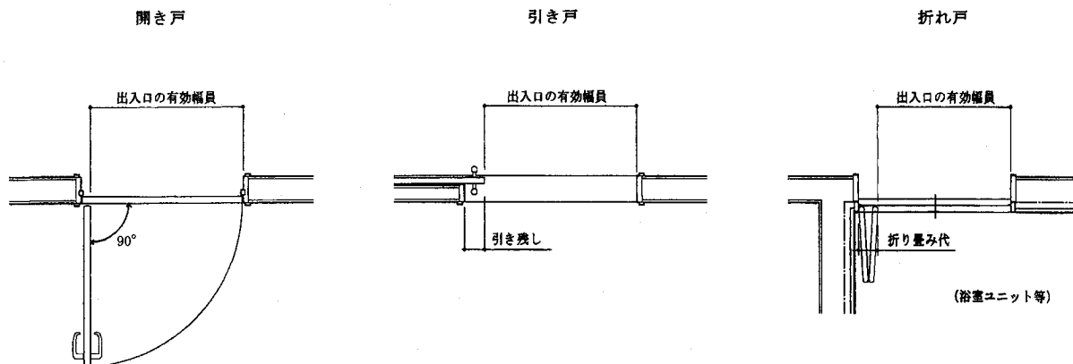
参考図4.6-2 出入口の有効幅員の計測方法
