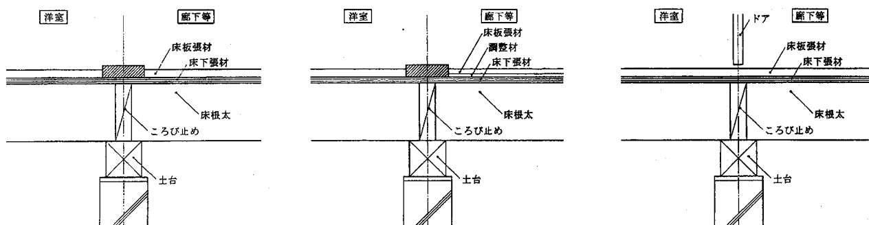
参考図4.3.3 洋室・廊下の段差解消の例
