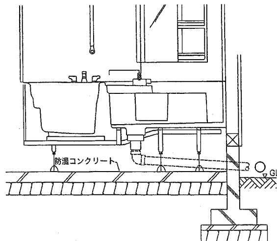
参考図5.9-3 浴室下部の配管方法
