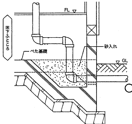
参考図 5.9-2 べた基礎の場合の配管方法（基礎を切り下げた場合）
