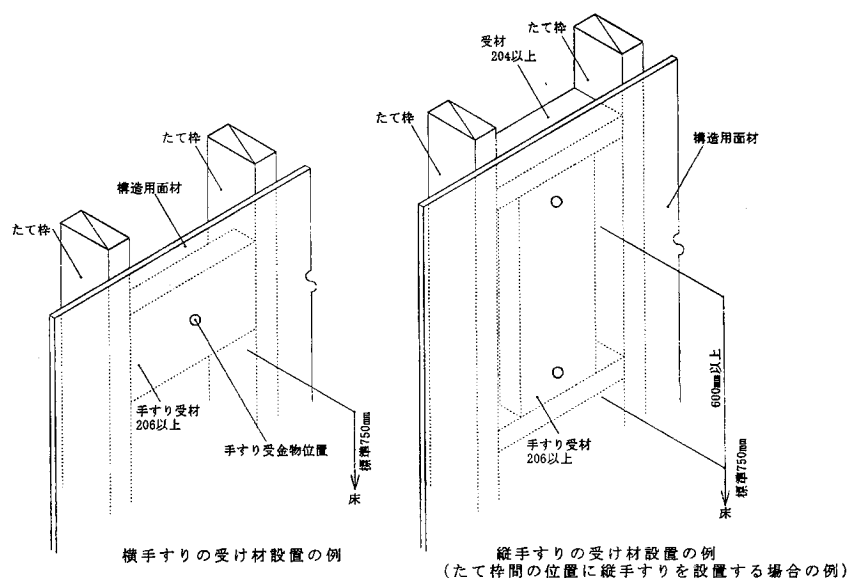
参考図4.5-2 手すり受け材の設置例
