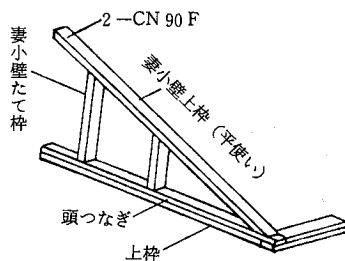
4.9-5図 妻小壁
