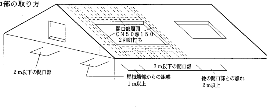
4.9-29 図 屋根開口部の取り方
