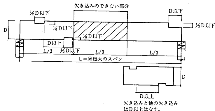
4.6-18図 床根太の欠き込みの制限
