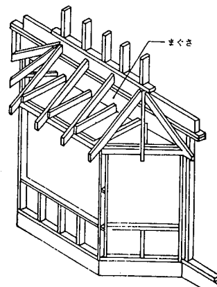
4.7-10図 出窓などのまぐさの入れ方例
