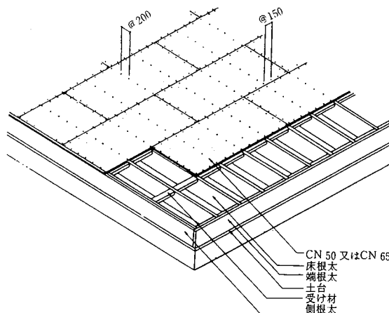
4.6-21図 床下張材の張り方と釘打ち
