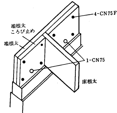
4.6-4図 床の補強
