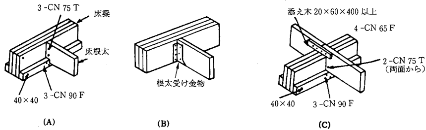
4.6-17図 根太がけの方法と釘打ち
