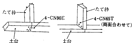
4.5-6図 土台を下枠として使用する際の継手
