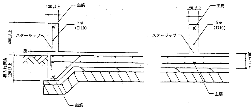
参考図 べた基礎詳細図(mm)
