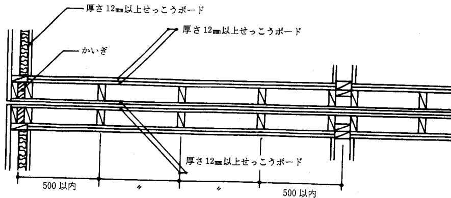
4.7-21 図 連続建の住戸間界壁
