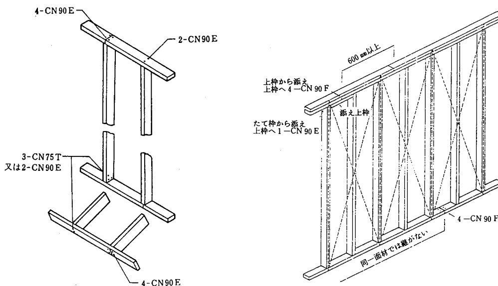
4.7-2 図 頭つなぎ釘打ち
