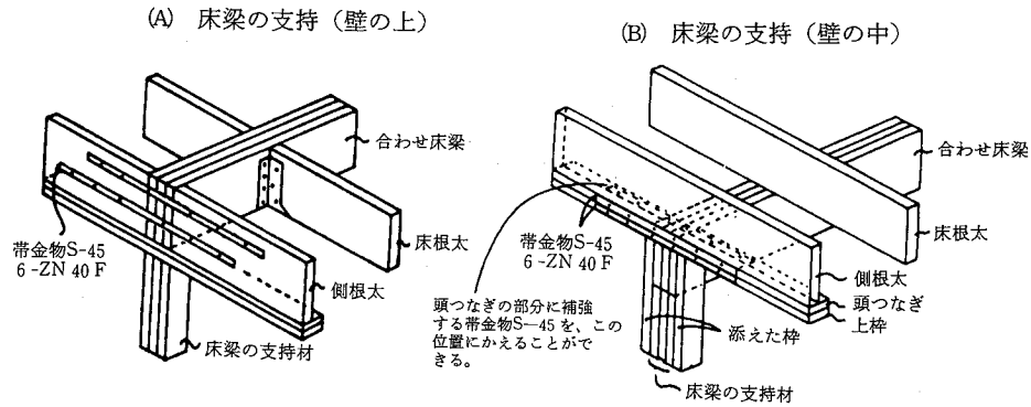
4.6-16図 床梁の支持
