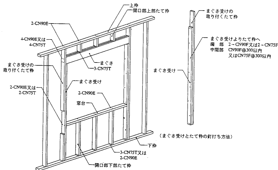
4.7-9図 開口部のまわりの釘打ち
