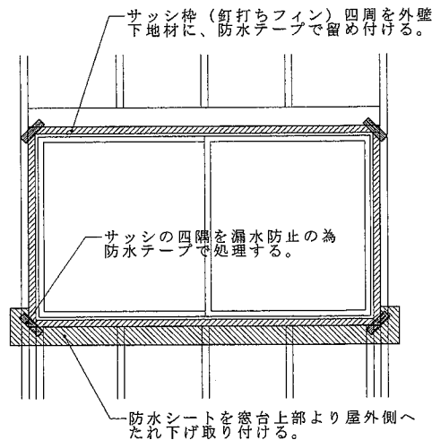
参考図 V. 7.3 建具の取り付け部の施工例 (漏水及び腐朽の防止)
